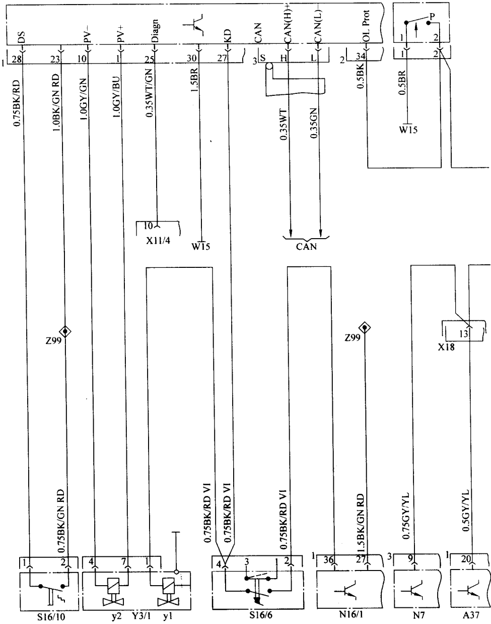
图 6-48 SL320 和 SL600 防盗报警系统电路图之三 (1997 车型)
