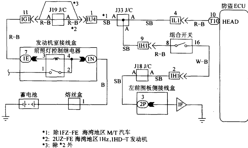
图 2-15 前照灯控制继电器电路
