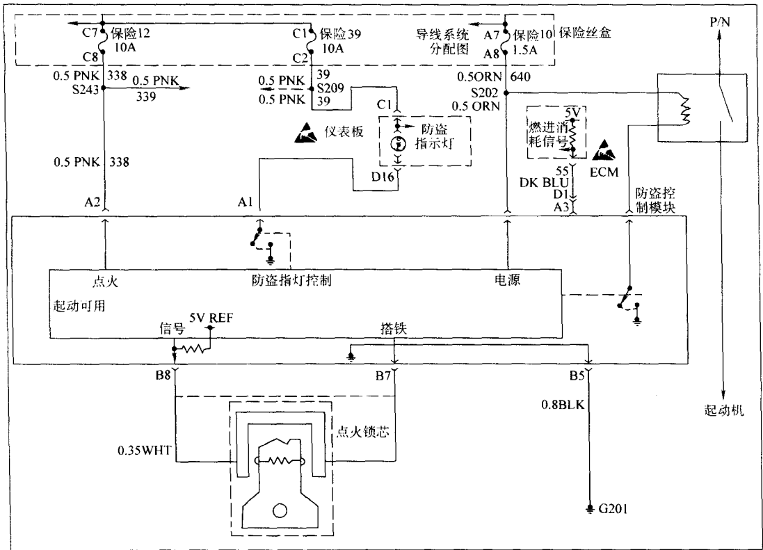
图 10-1 PASS-KEY 防盗系统电路
