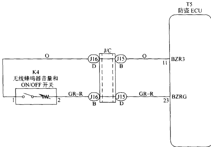
图 2-30 遥控门锁蜂鸣器音量和 ON/OFF 开关电路
