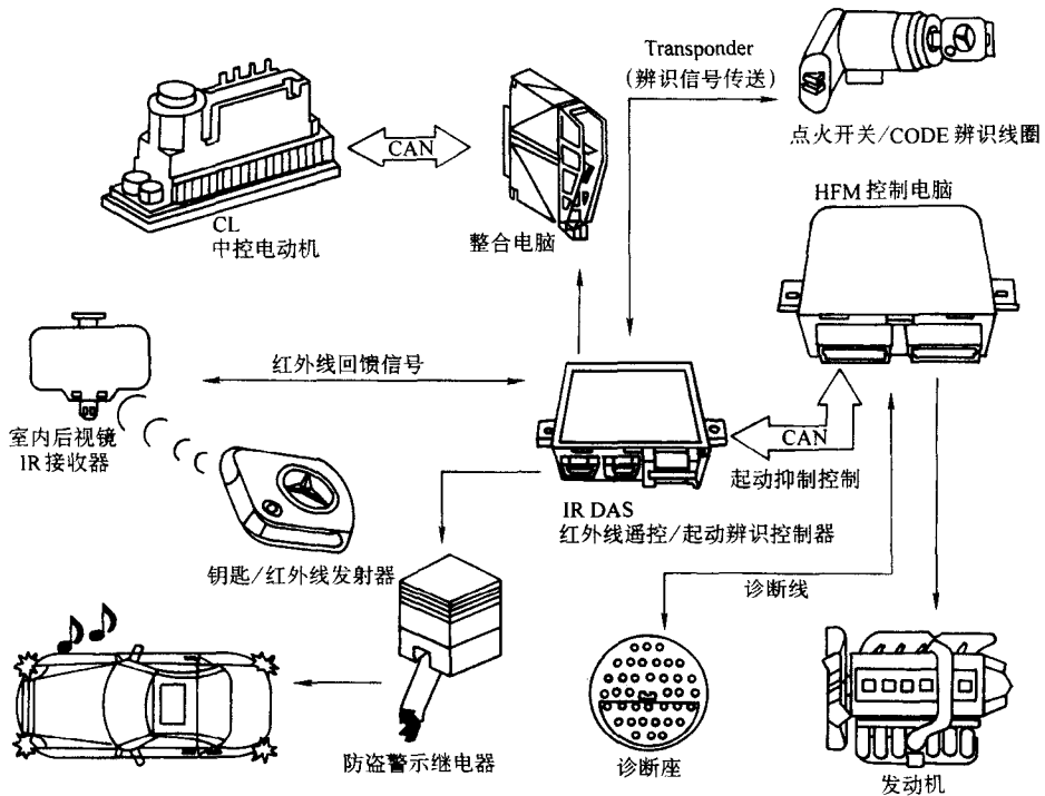
图 6-34 1996 年欧规 W210 底盘中控防盗控制图
