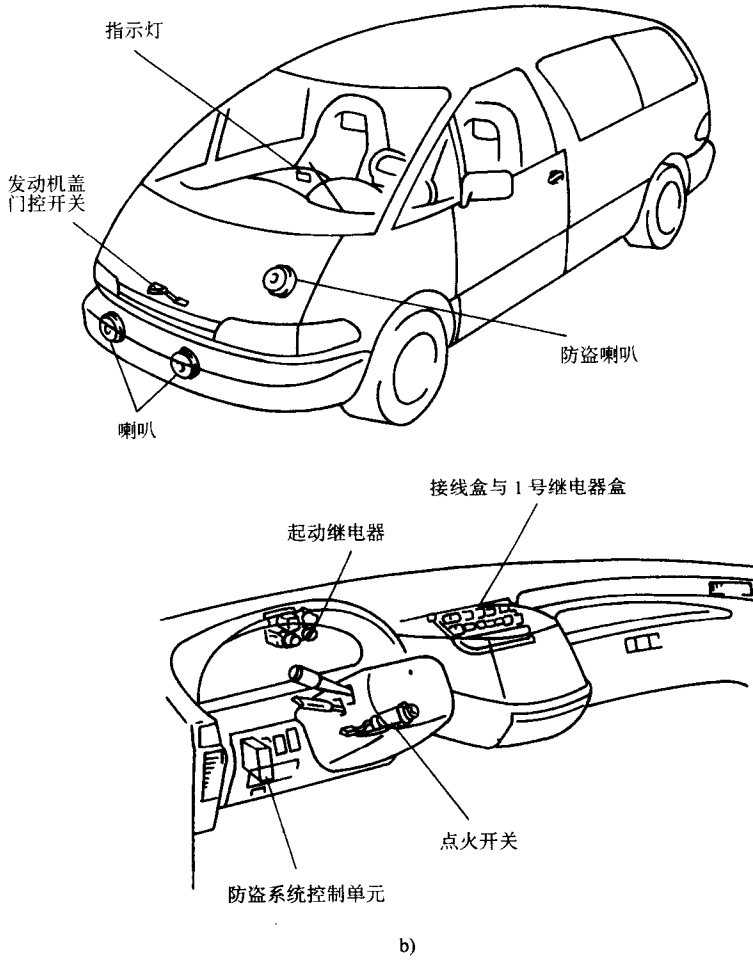
图 2-1 防盗系统元件位置 (续)
