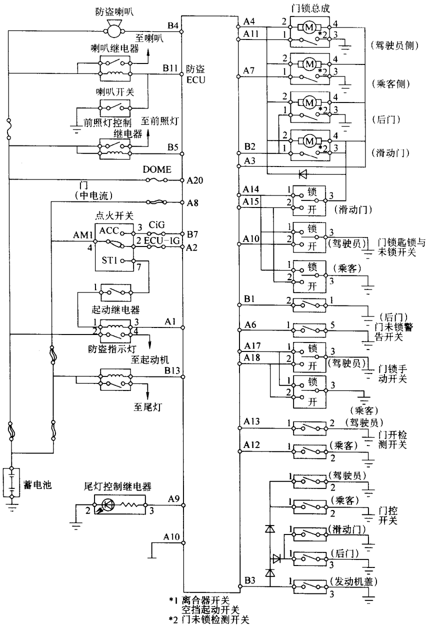
图 2-2 防盗系统电路
