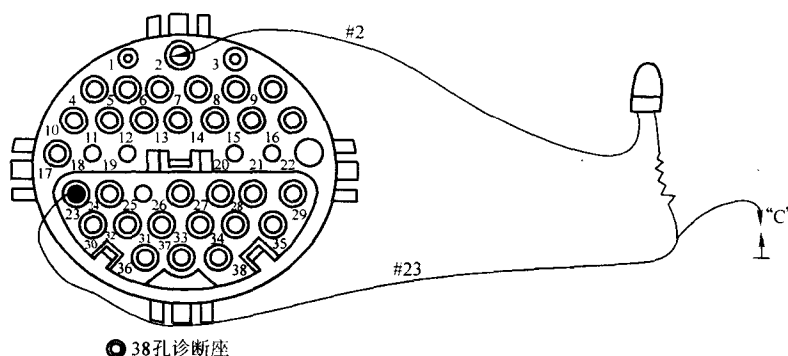
图 6-42 奔驰 W202/140 车型防盗系统故障码读取接线
