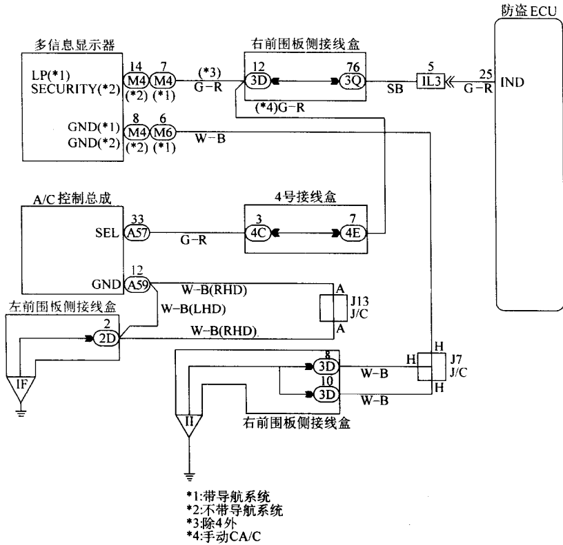
图 2-5 防盗指示灯电路
