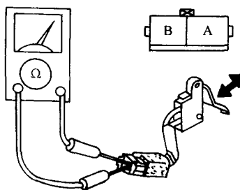
图 4-15 检查行李箱灯开关
