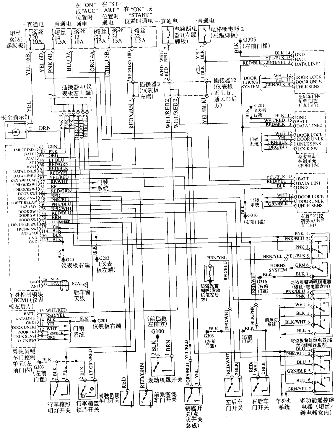
图 3-43 防盗系统电路 (续)
