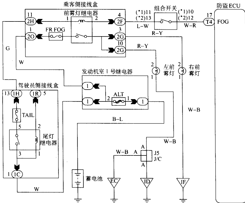
图 2-47 前雾灯开关和继电器电路
