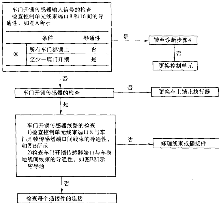
图 3-60 诊断步骤 3 流程 (续)
