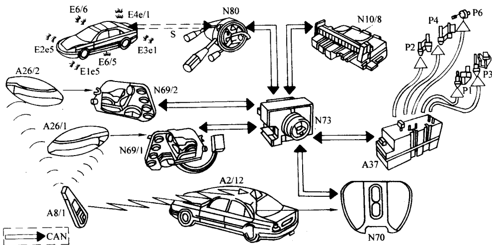
图 6-19 工作控制流程
