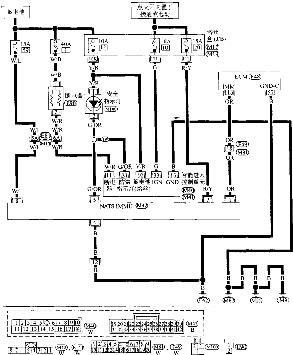
图 3-2 日产风度 A33 防盗系统电路
