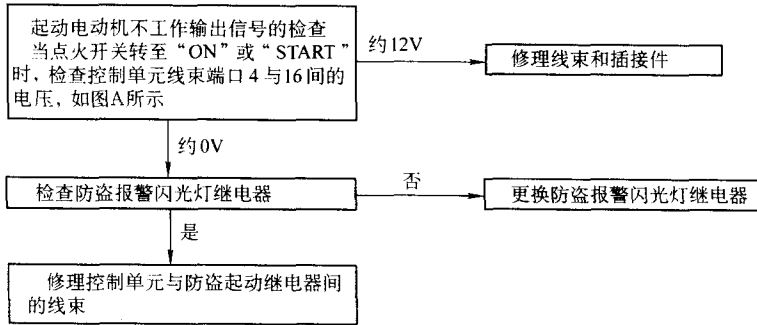
图 3-63 诊断步骤 6 流程 (续)
