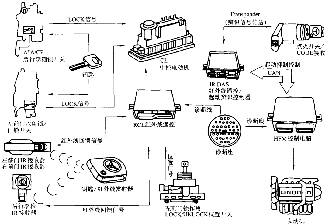
图 6-26 1997 年美规 W129 底盘中控防盗控制图
