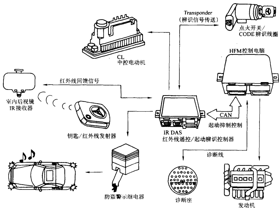
图 6-32 1996 年欧规 W202 底盘中控防盗控制图
