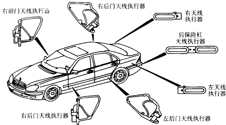
图 6 - 12 各天线执行器说明图
