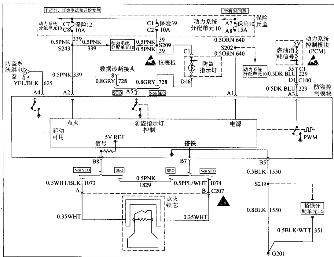
图 10-2 PASS-KEY II 防盗系统电路
