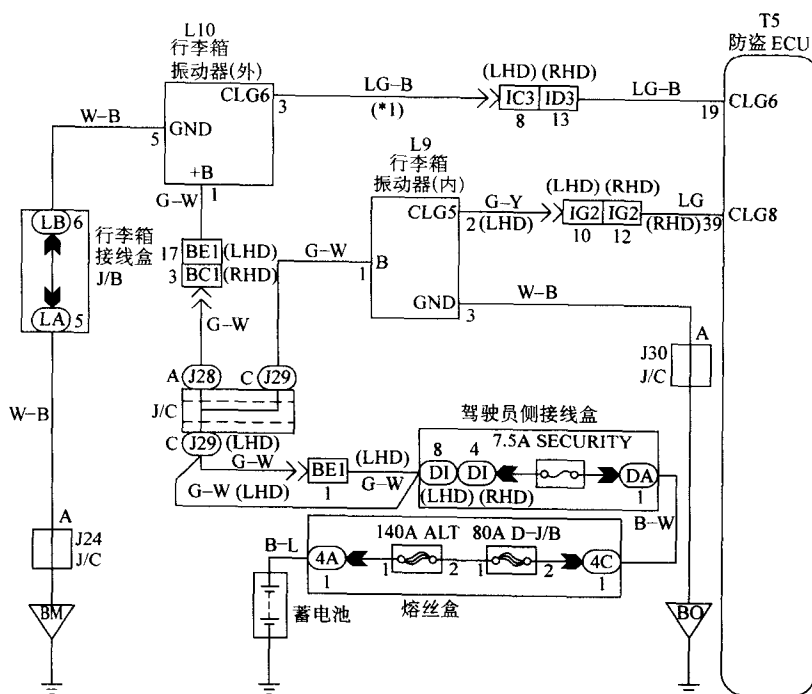
图 2-37 行李箱振动器电路 (内、外)
