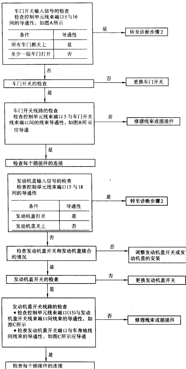
图 3-58 诊断步骤 1 流程 (续)
