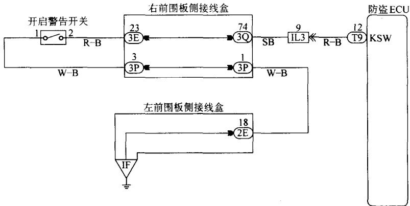
图 2-7 钥匙开启警告开关电路
