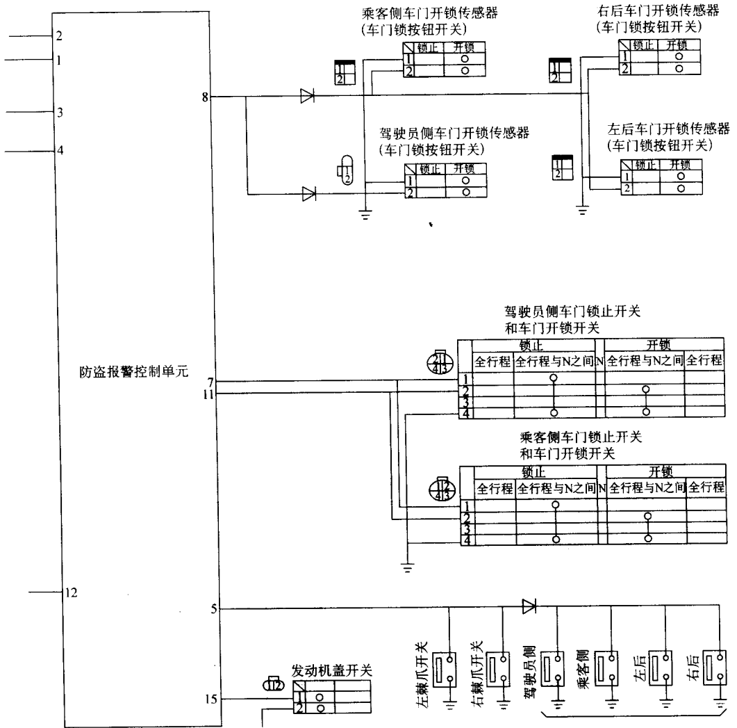
图 3-56 日产风度防盗系统故障诊断速查电路
