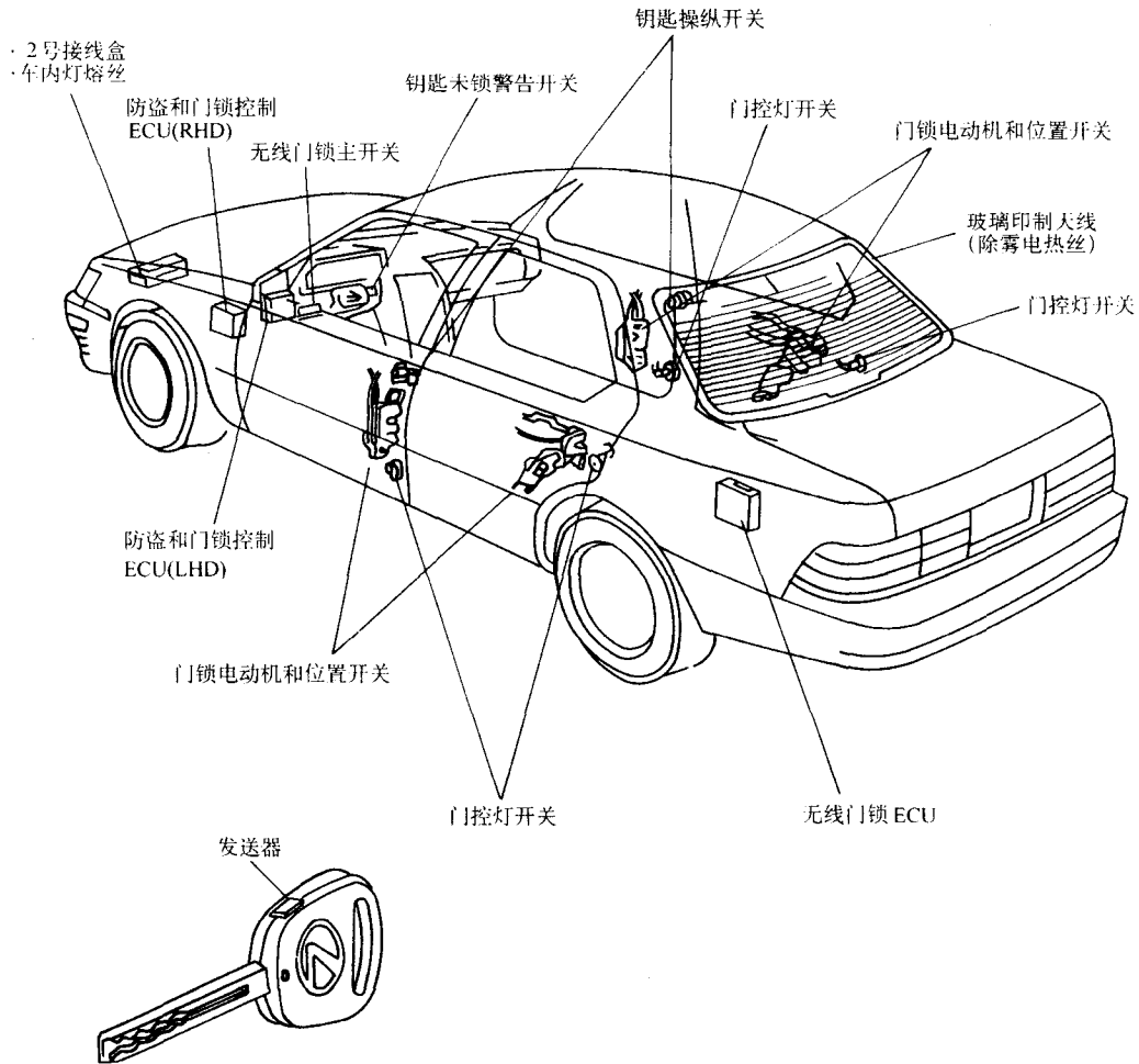
图 2-60 丰田凌志 LS400 与 ES300 无线电遥控的元件布置
