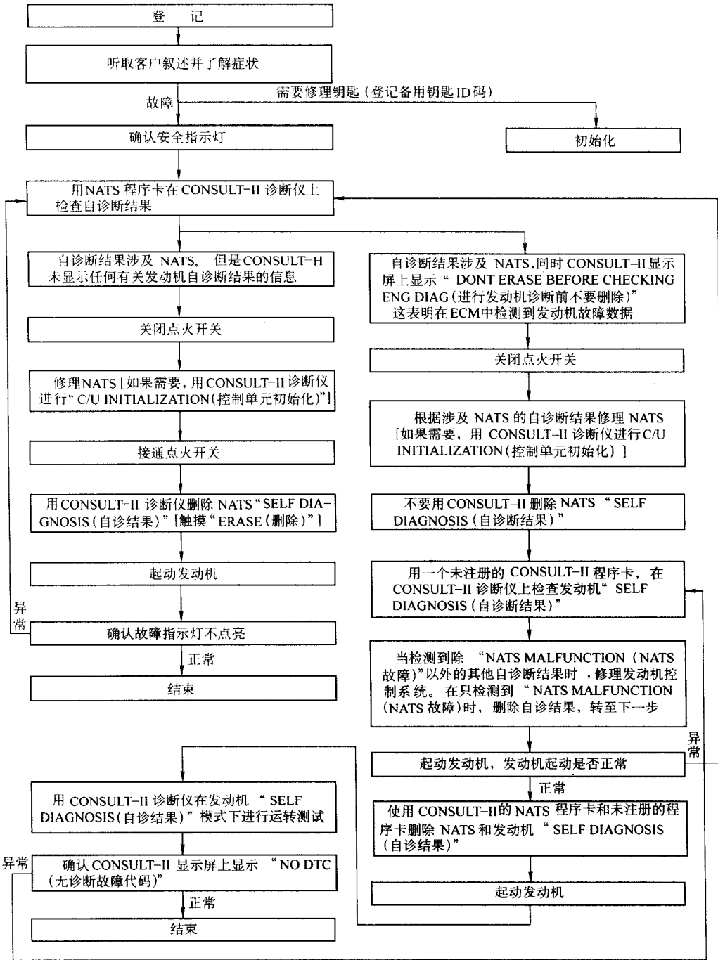
图 3-5 故障诊断程序
