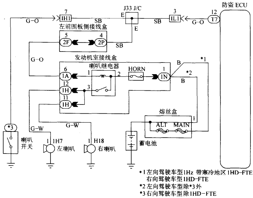
图 2-14 喇叭继电器电路
