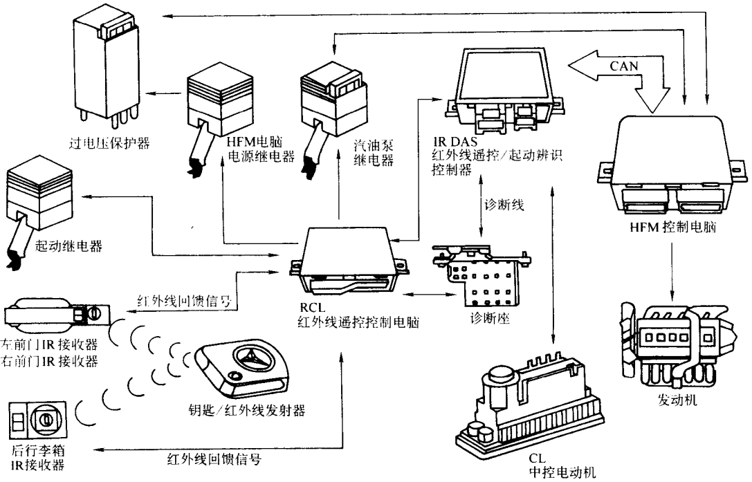
图 6-29 1996 年欧规底盘 W124 中控防盗控制图
