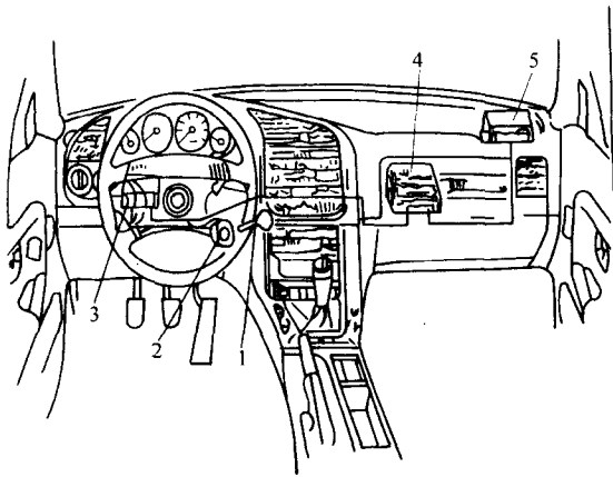
图 7-7 EWS - II 系统各部分零件位置
