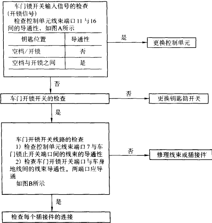
图 3-64 诊断步骤 7 流程 (续)
