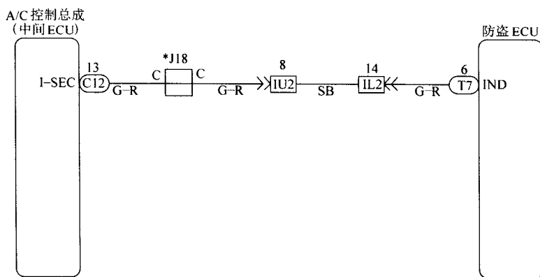
图 2-11 指示灯电路
