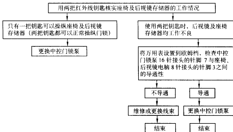
图 5-9 诊断流程
