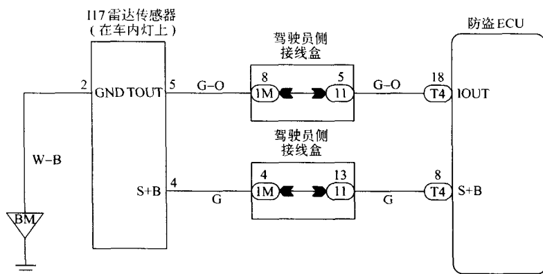
图 2-52 雷达传感器电路
