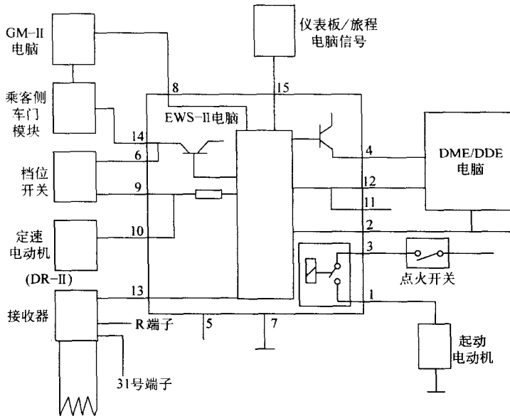
图 7 - 12 EWS - II 系统示意图
