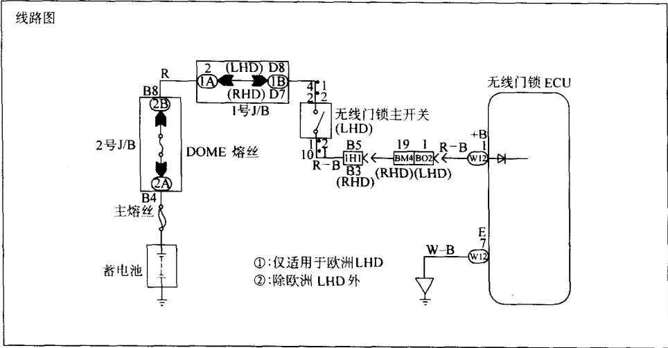
图 2-68 ECU 电源电路检查 (续)
