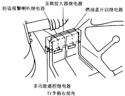
图 3-29 防盗系统元件位置
