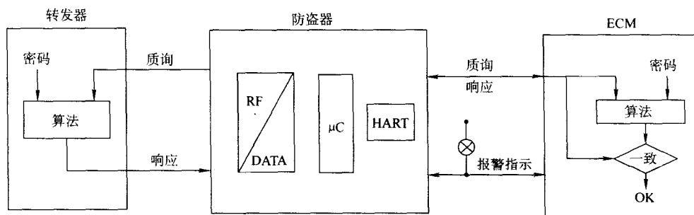
图 10-7 IMO 防盗系统的典型电路
