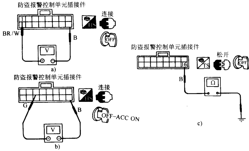
图 3-57 检查电源和搭铁线路
