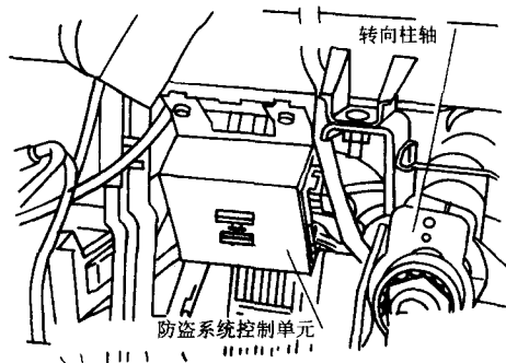
图 3-44 防盗系统控制单元位置
