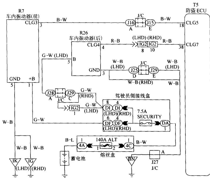
图 2-36 车内振动器电路
