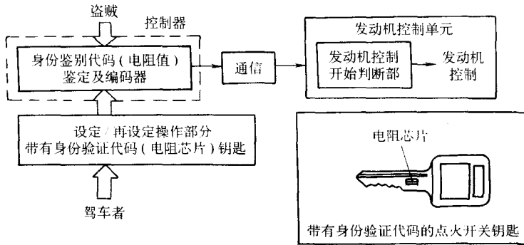
图 1-13 防盗装置的工作过程
