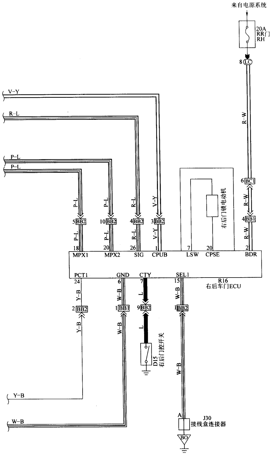
能钥匙系统) 电路 (续)
