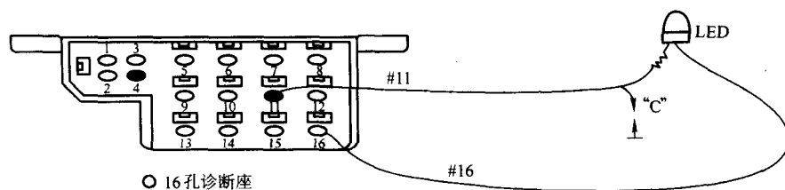
图 6-41 奔驰 W129 车型防盗系统故障码读取接线
