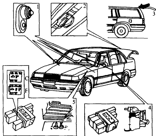
图 8-28 沃尔沃 9 系列中央门锁与防盗系统部件位置之三
