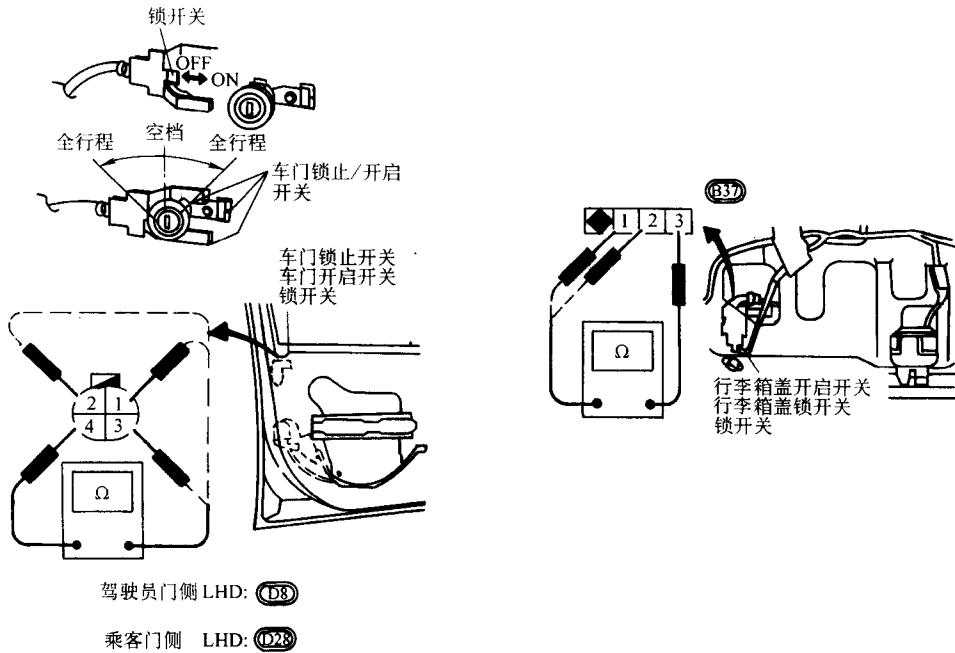
图 3-23 车门锁止开关及车门开启开关位置
