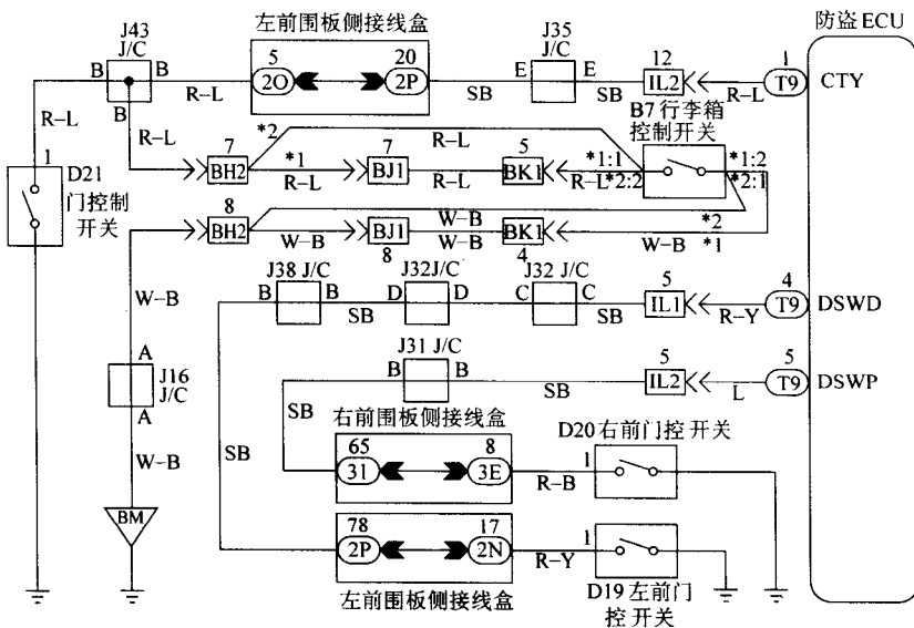
图 2-22 车门开启检测开关电路
