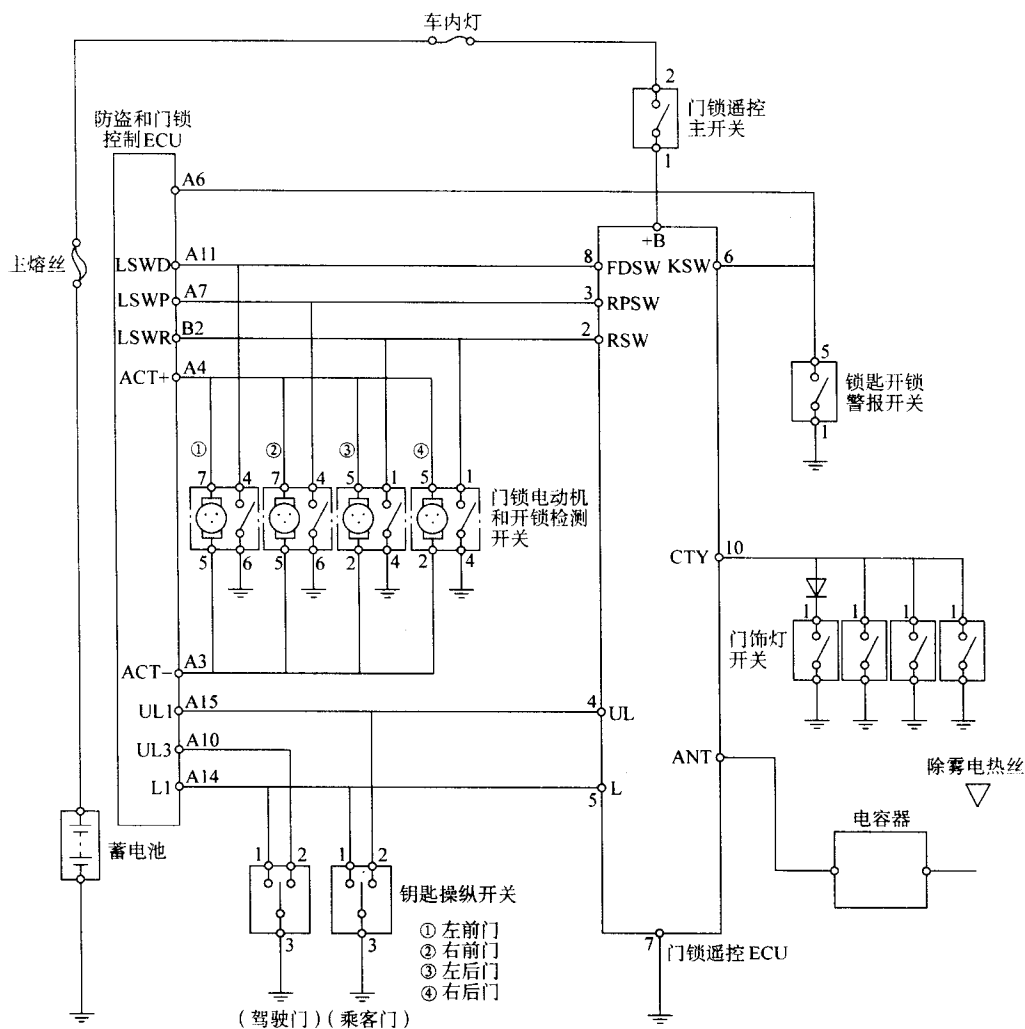
图 2-62 丰田凌志 ES300 无线电遥控系统的电路
