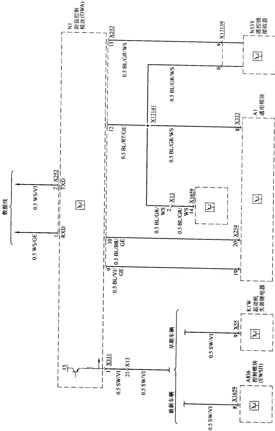
图 7-38 宝马 850ci (E31) 防盗系统数据线、驾驶保护及 QZV 电路 (1996 年车型)
