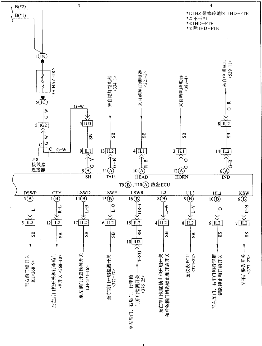
防盗系统电路
