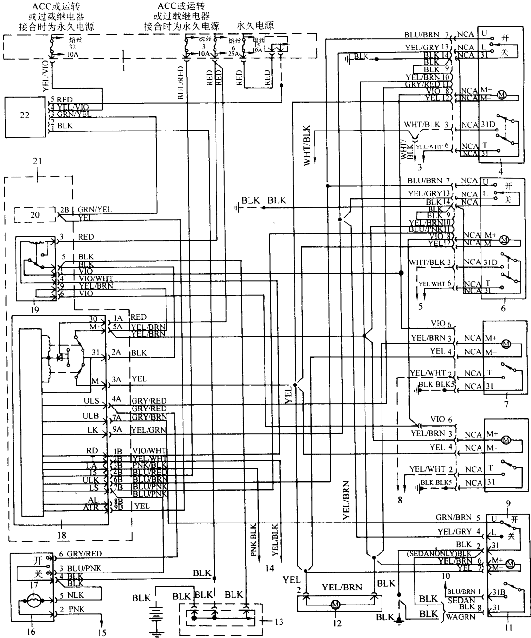
图 8-15 沃尔沃 850 中控遥控及防盗系统电路 (1996 年车型)
