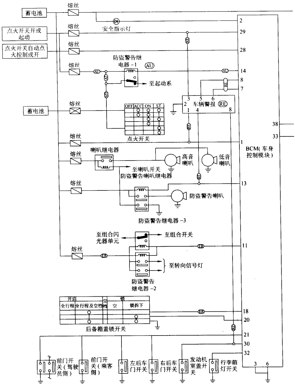
图 3-12 防盗系统原理
