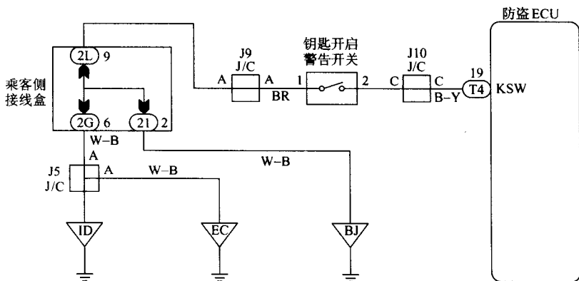
图 2-49 钥匙开启警告开关电路
