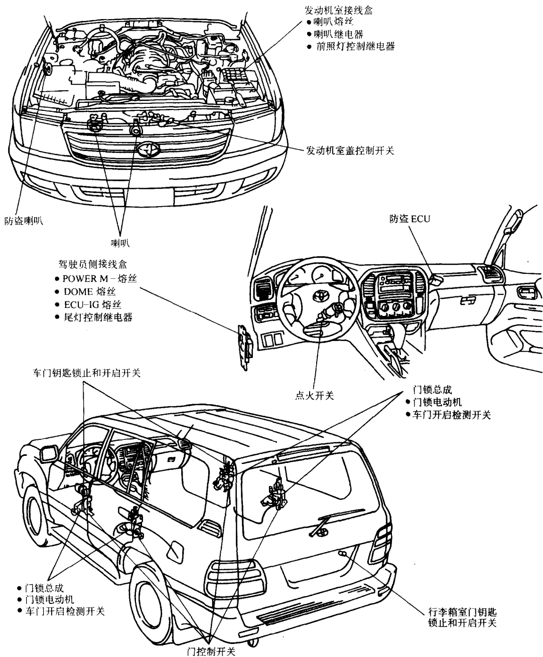
图 2 - 10 防盗系统电控元件位置
