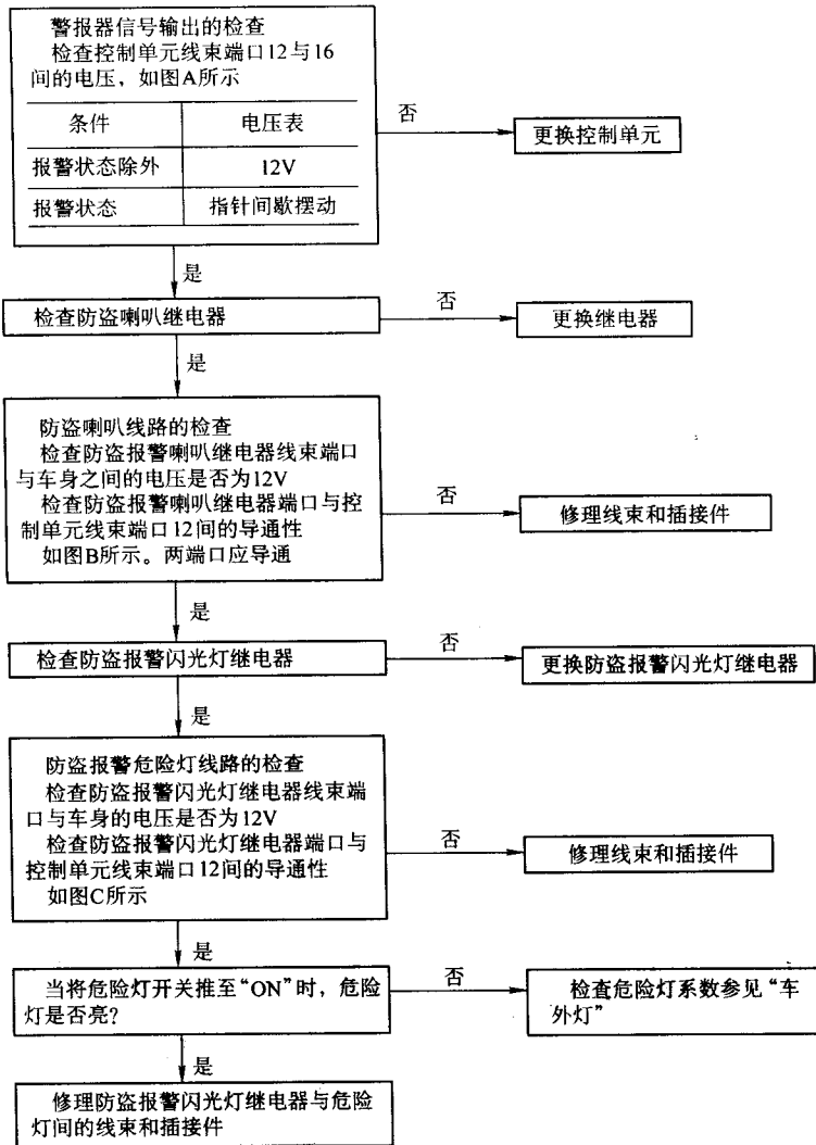
图 3-62 诊断步骤 5 流程 (续)
