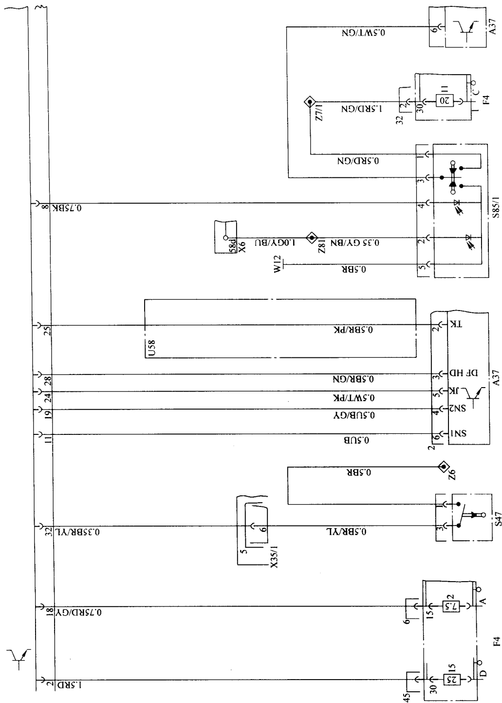
图 6-45 奔驰 S 系列防盗系统电路图之二 (1997 和 1998 车型)
