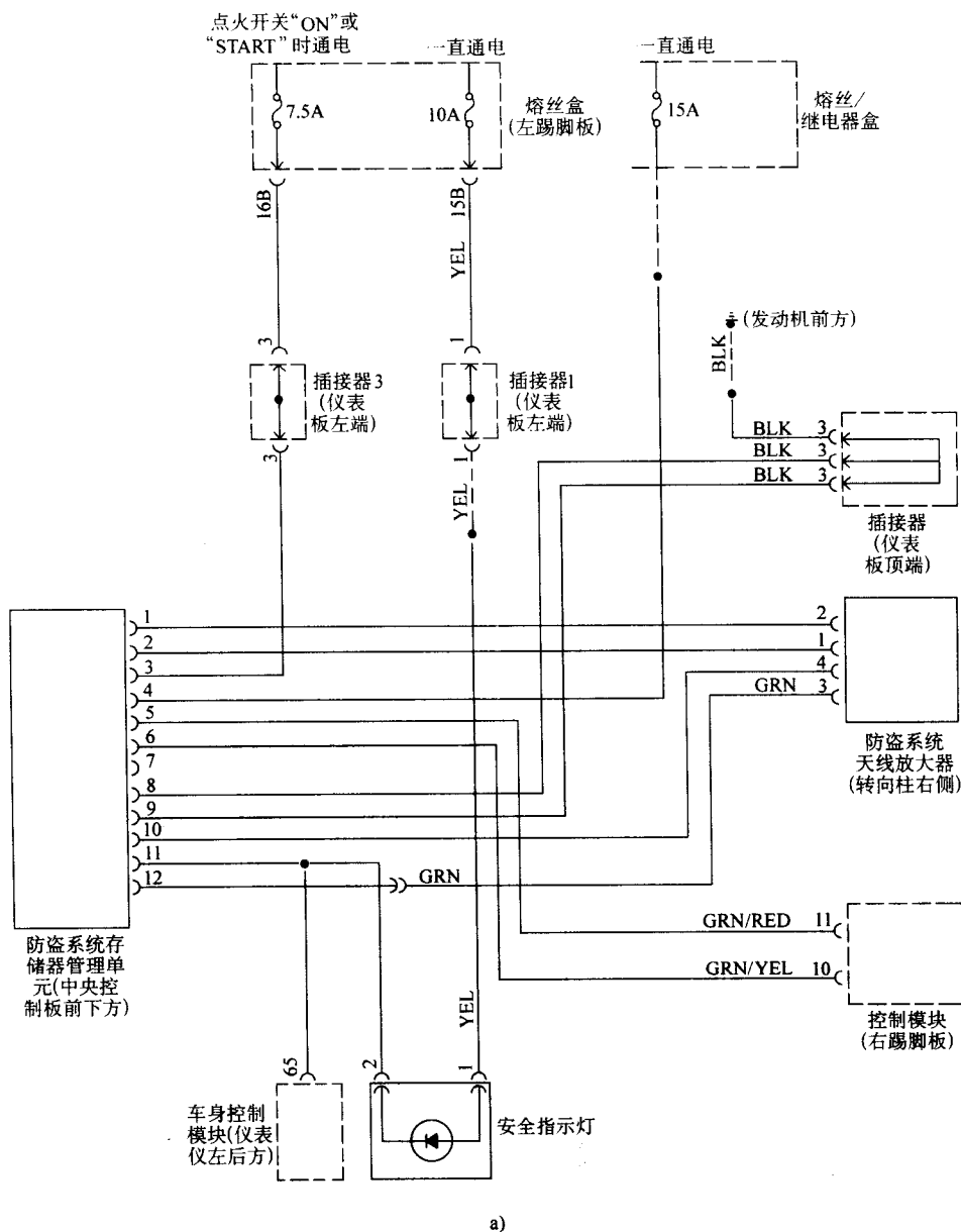
图 3-43 防盜系统电路
