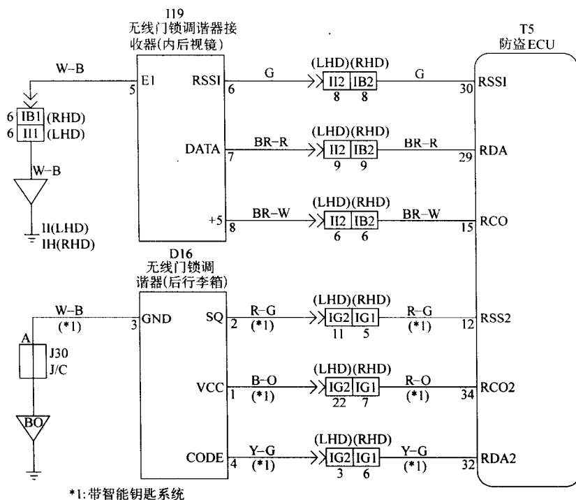
图 2-26 故障码 B1242 检查电路
