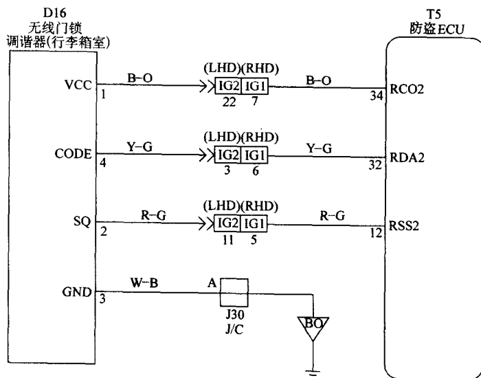
图 2-38 遥控门锁接收器电路 (行李箱室)
