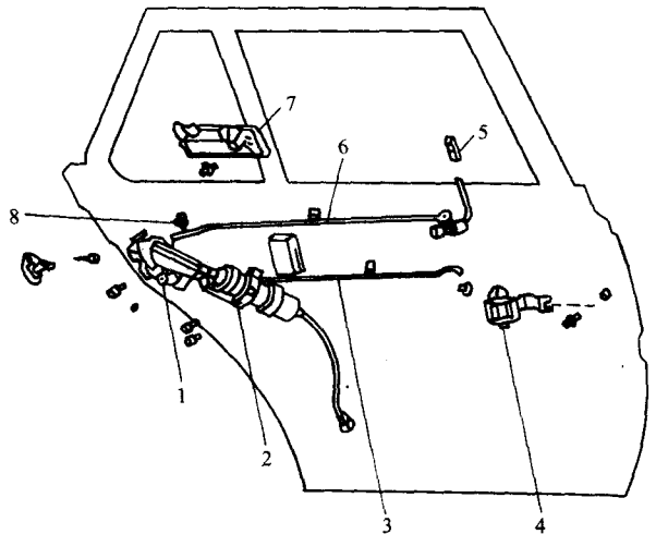
图 1-16 电控门锁布置
