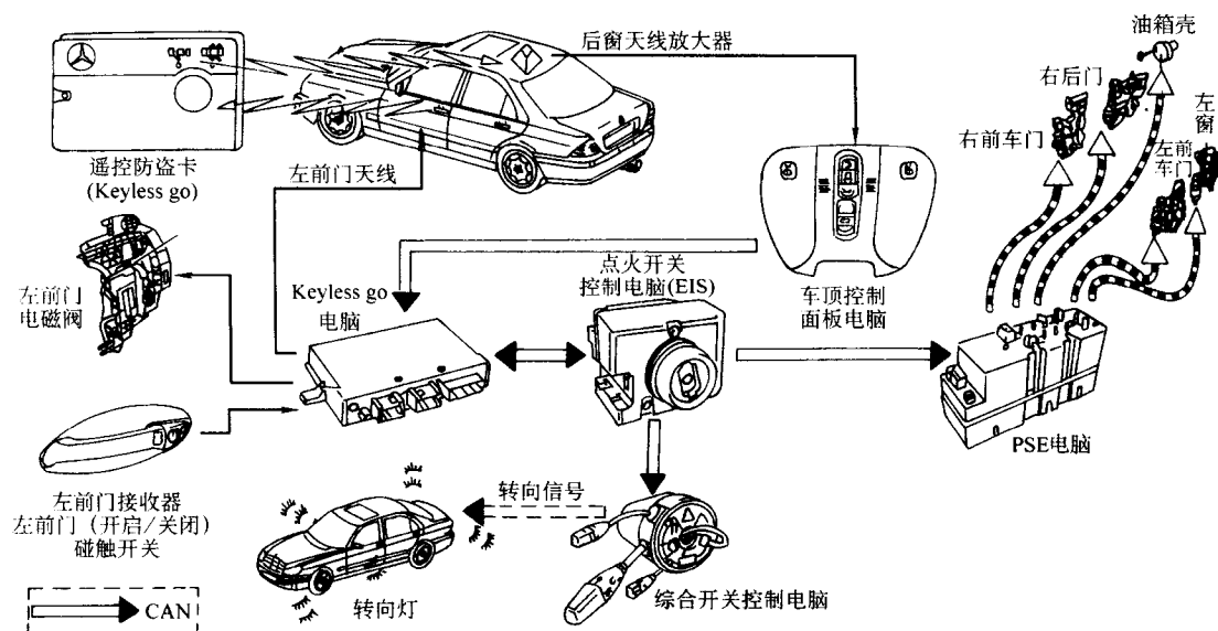
图 6-13 车门的开启功能
