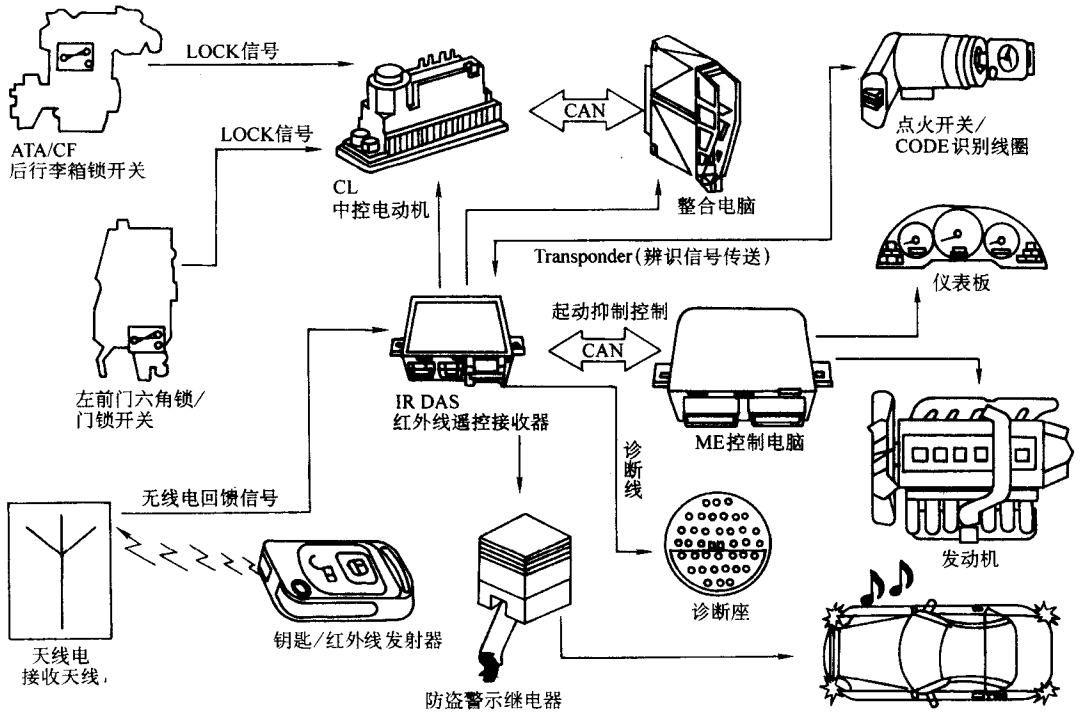
图 6-28 1998 年美规 R170 底盘中控防盗控制图
