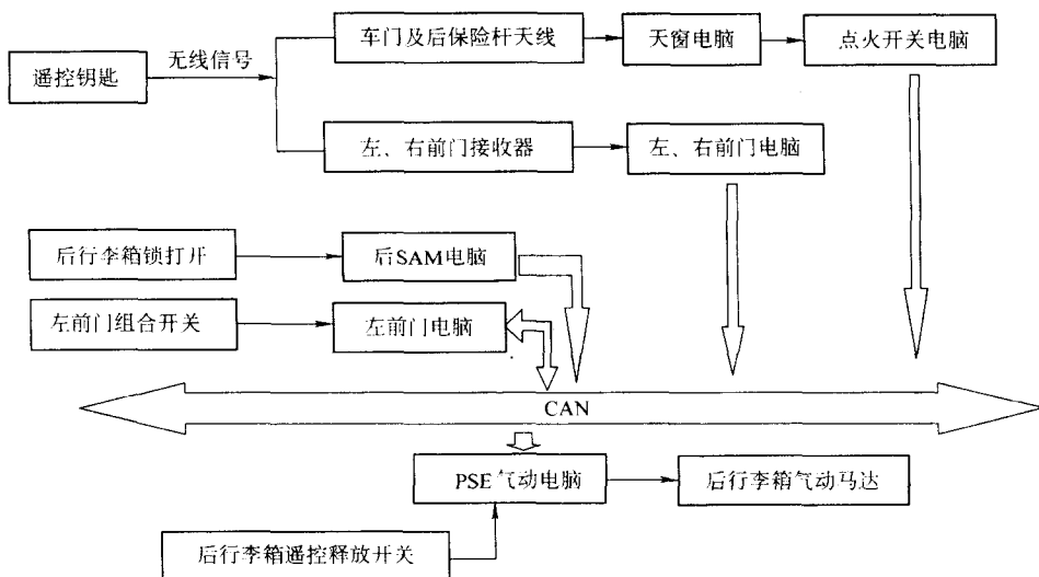
图 6-23 工作流程
