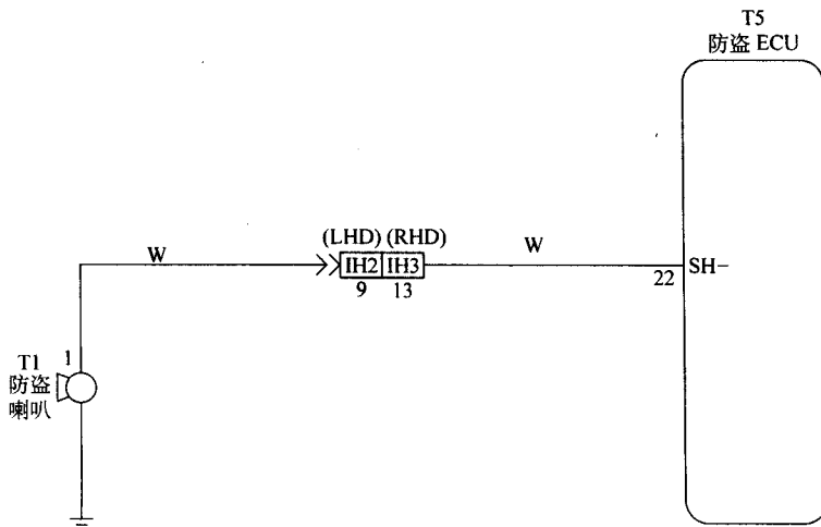
图 2-33 防盗喇叭电路
