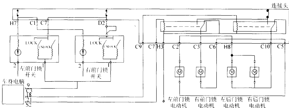
图 12-3 Concorde、Intrepid、LHS、Neon、New Yorker 和 Vision 中控线路
