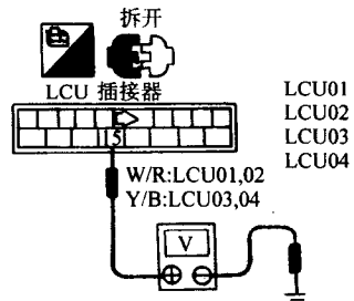
图 3-31 测量 BCM 电源不同电压
