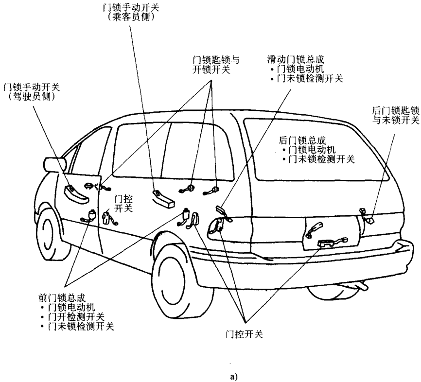
图 2-1 防盗系统元件位置
