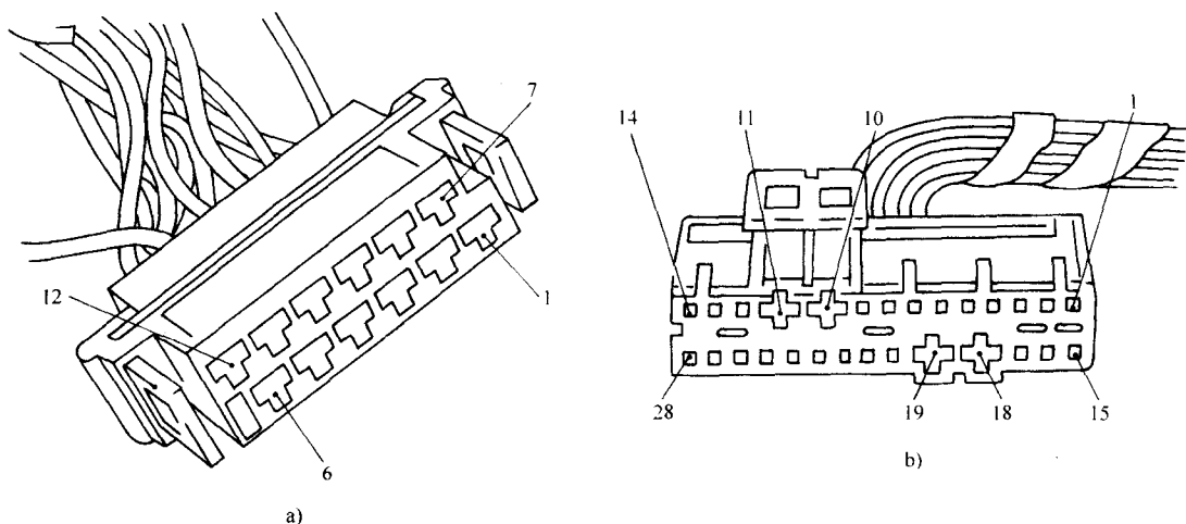
图 9-6 防盗报警系统和中央门锁系统控制单元配线连接器
