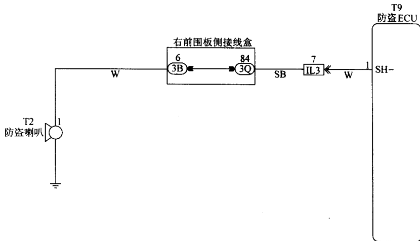
图 2-6 防盗喇叭电路
