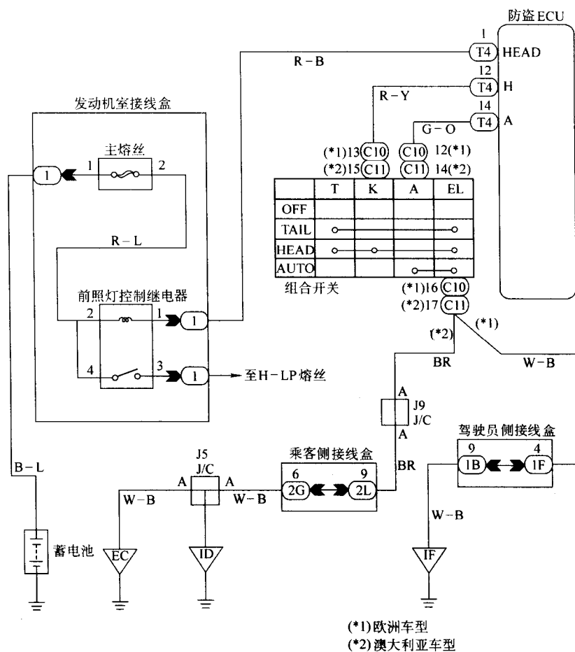
图 2-46 灯控制开关电路
