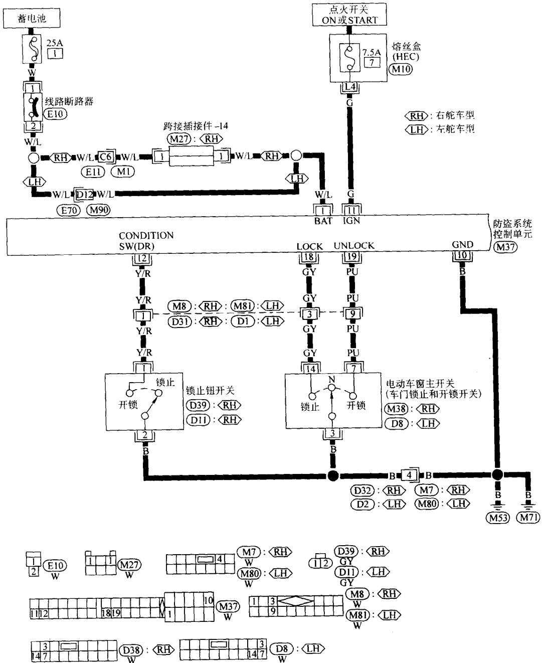
图 3-47 车门锁控制电路
