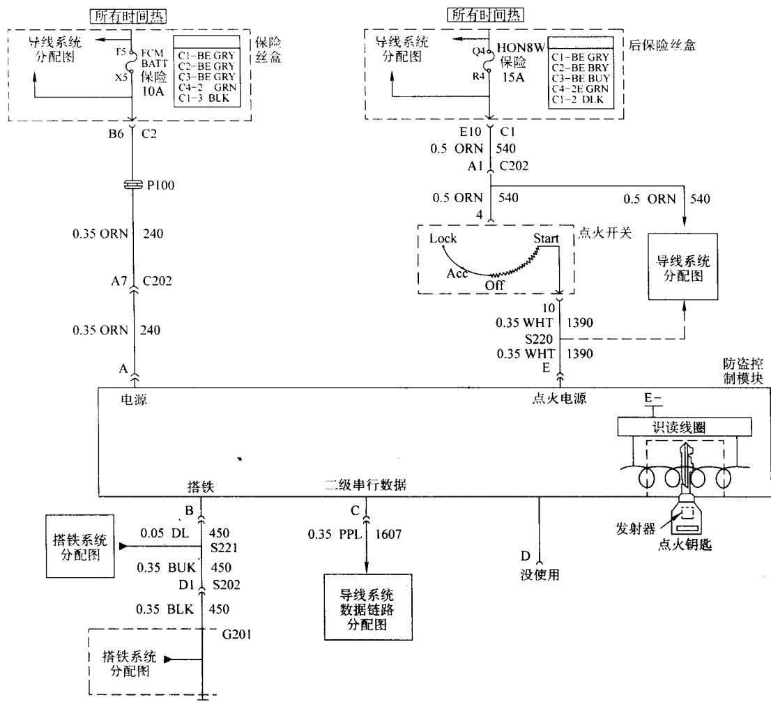
图 10-5 PASS-KEY III 防盗系统典型电路
