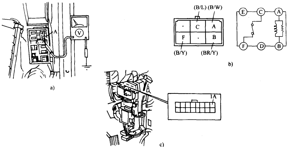
图 4-9 起动机工作的排除
