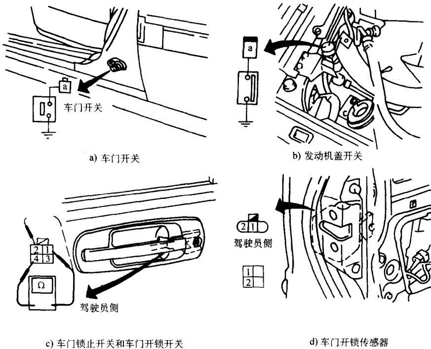
图 3-65 诊断步骤 7 中的检测
