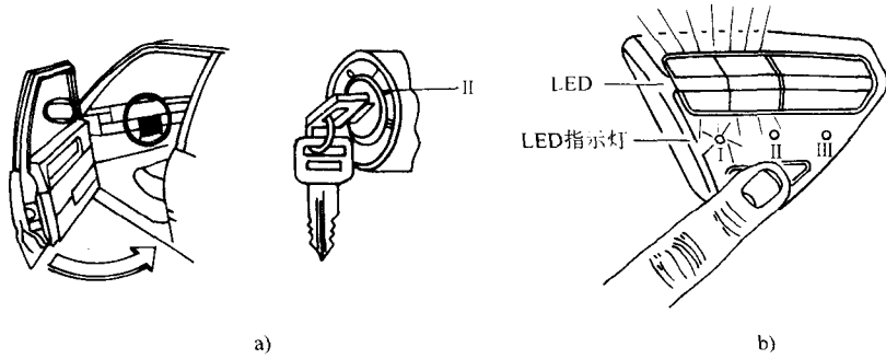
图 8-3 防盗系统遥控器设定方式 a) 关闭车门 b) 遥控接收器
