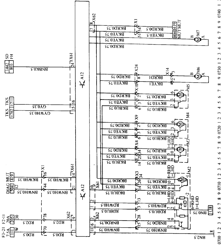
图 9-5 赛飞利汽车防盗报警系统和中央门锁系统电路
