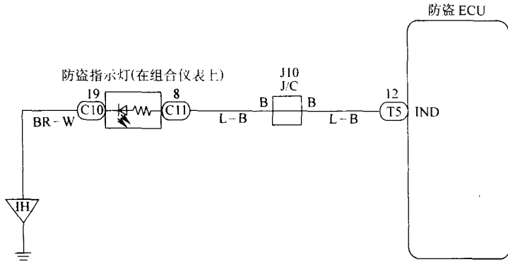
图 2-42 指示灯电路
