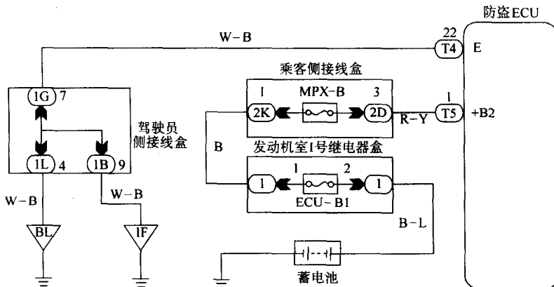
图 2-43 防盗 ECU 电源电路
