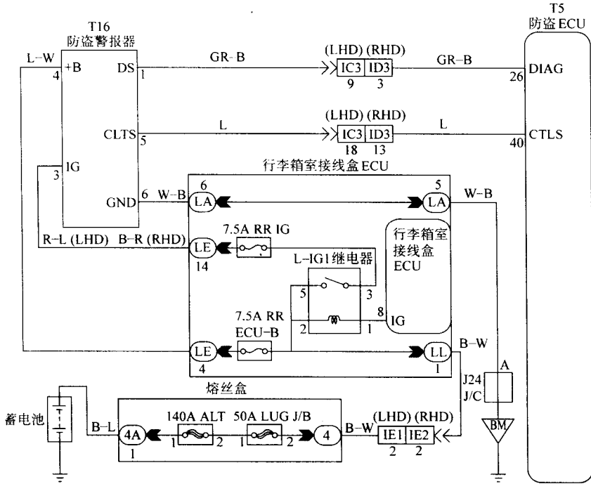
图 2-34 防盗警报器电路
