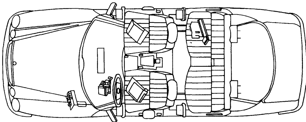
图 6-24 奔驰车中控防盗的元件位置
