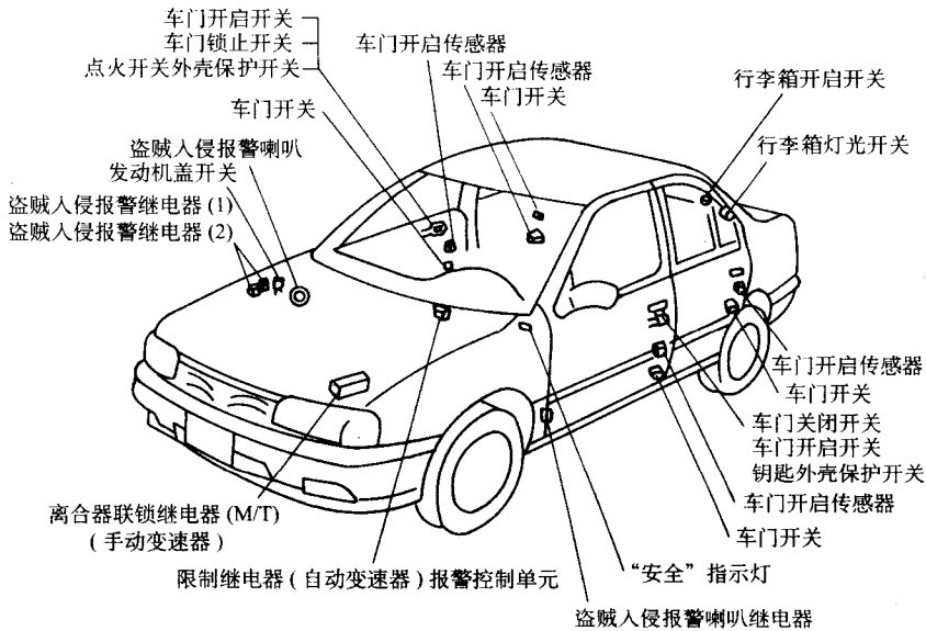
图 1-9 防盗装置在车辆上的布置
