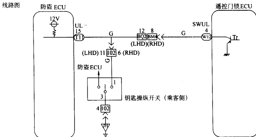
图 2-70 钥匙操纵开关电路检查
