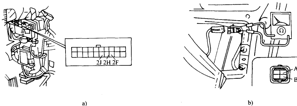
图 4-5 蜂鸣器不响、安全灯不闪烁的故障排除
