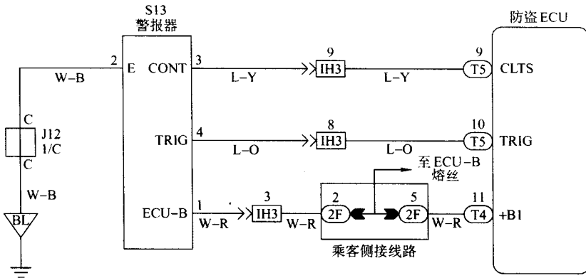
图 2-51 警报器电路
