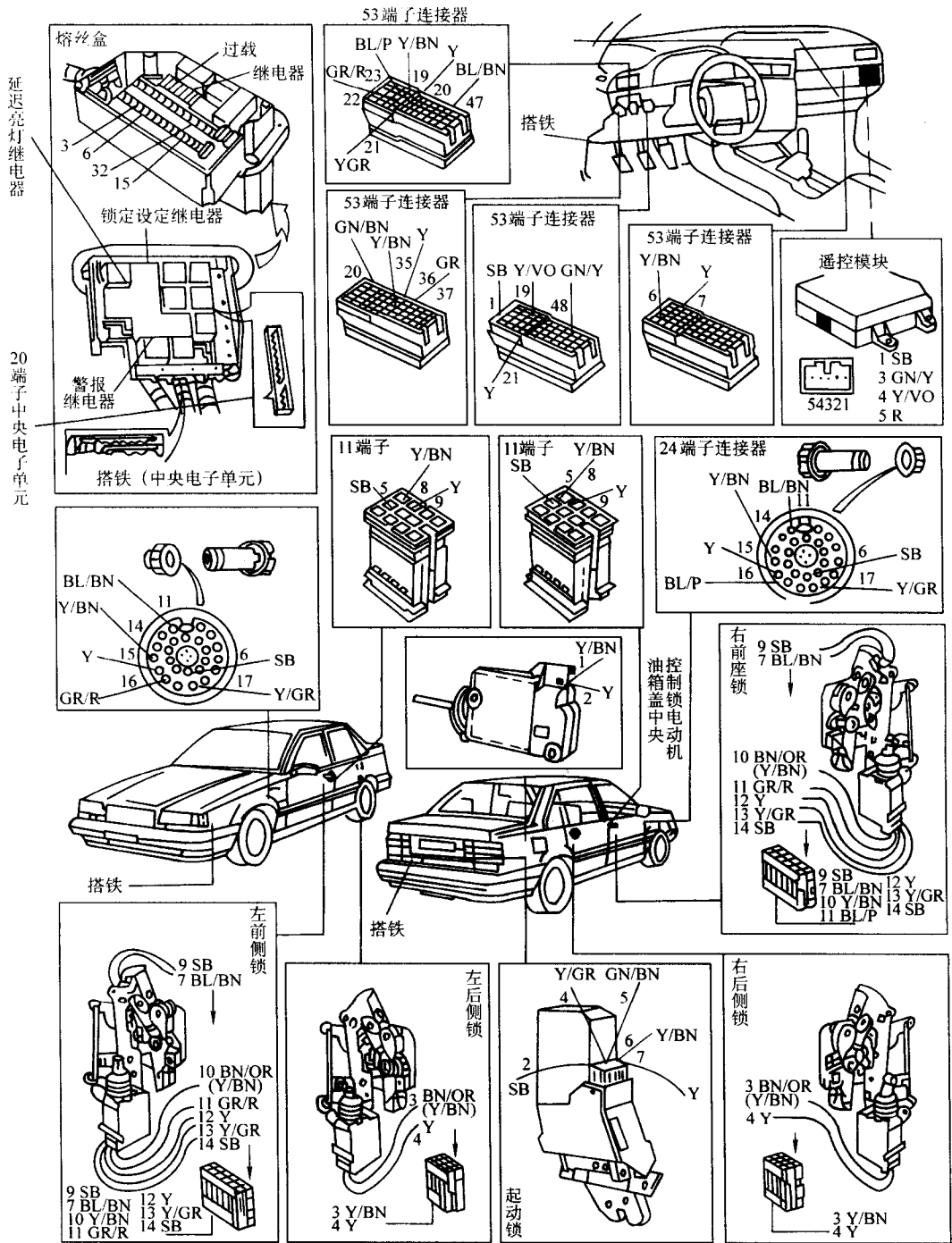
图 8-18 沃尔沃 850 防盗系统部件位置
