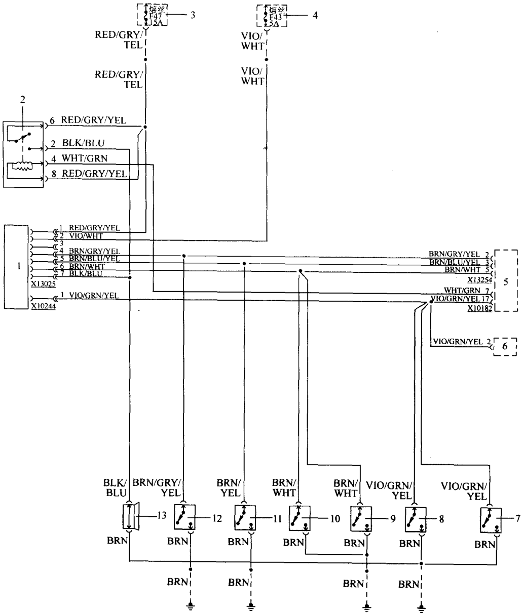
图 7-20 宝马 318i、318ic、318is、325i、325ic 和 325is 防盗系统电路 (1994 年, 后期生产)
