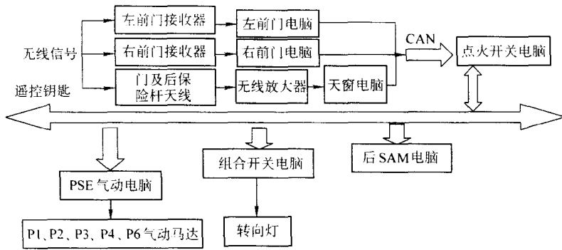
图 6-20 工作流程
