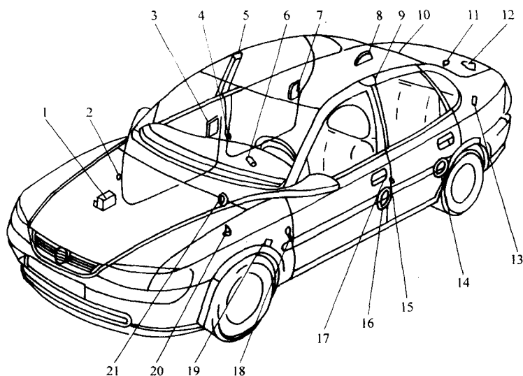
图 9 - 1 威达 - B 汽车防盗警报系统和中央门锁系统电控元件位置
