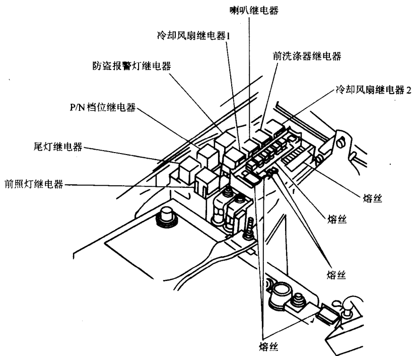
图 3-28 防盗系统元件位置
