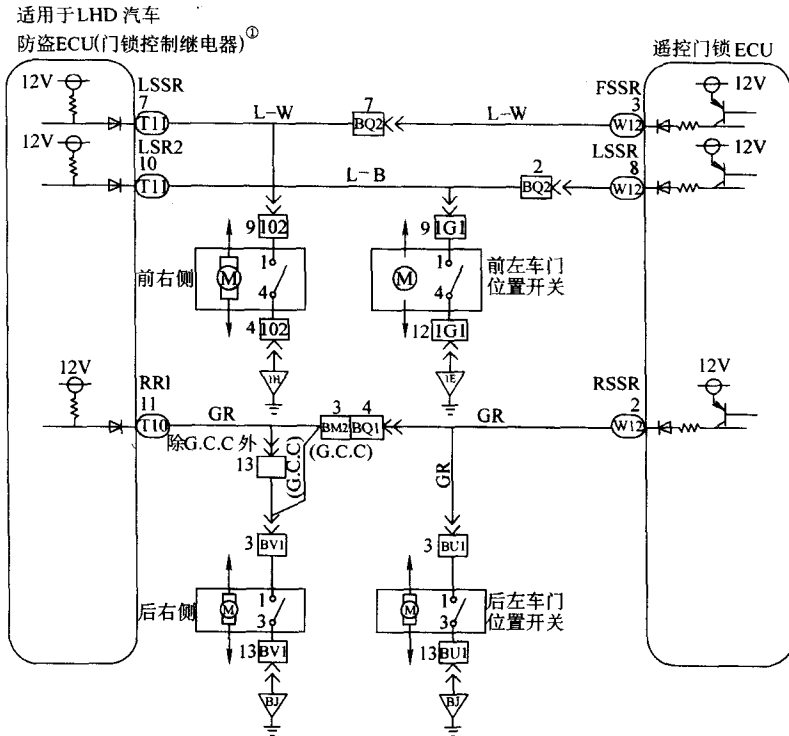
图 2-69 车门开关电路检查
