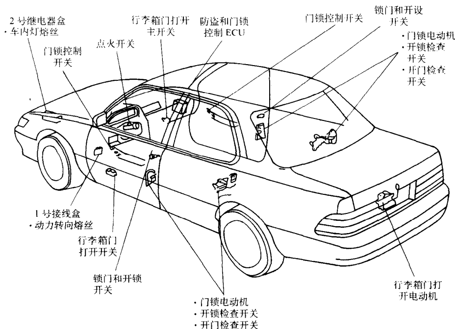
图 2-55 凌志 ES300 中央门锁系统元件位置
