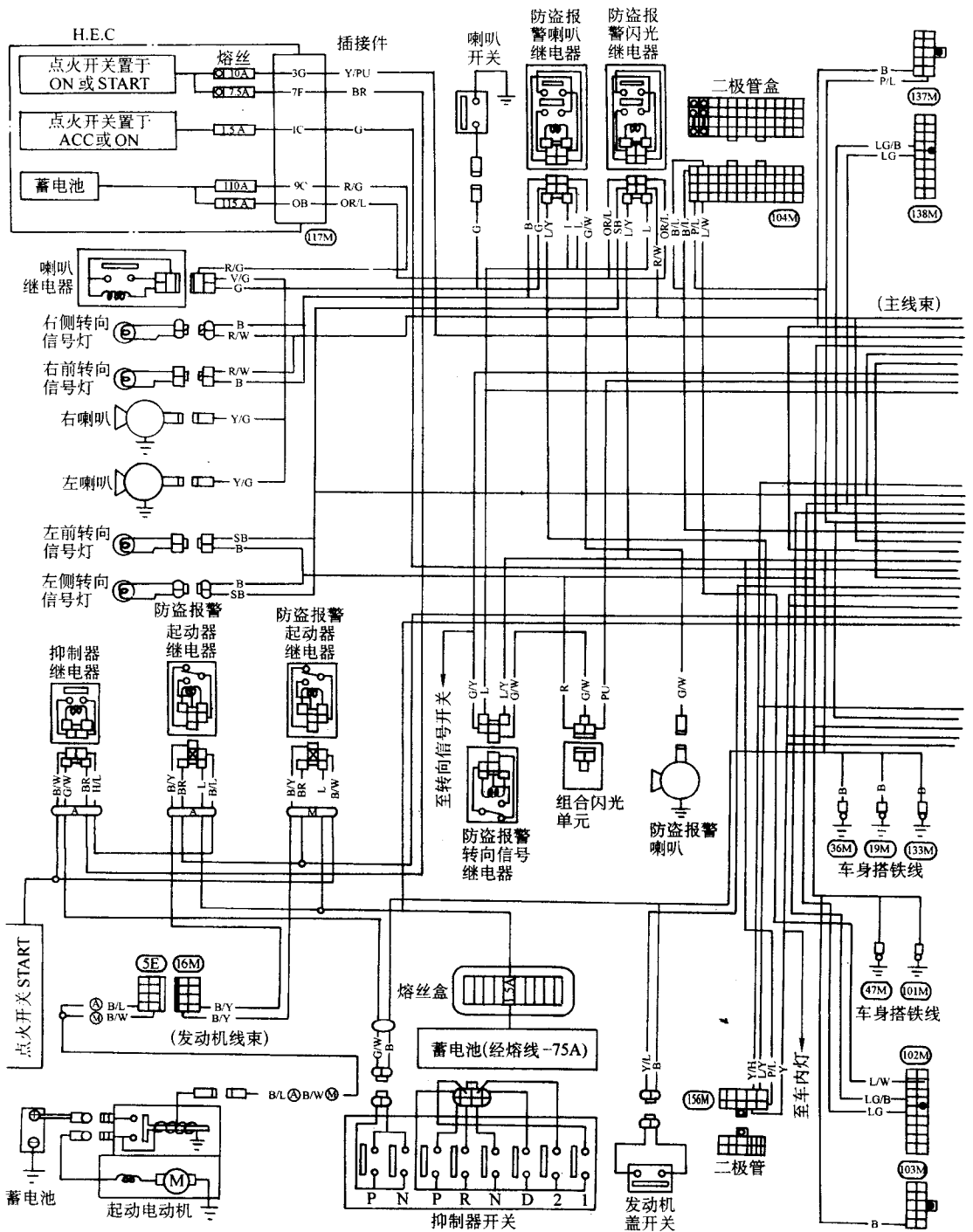
图 3-52 日产风度防盗系统电路
