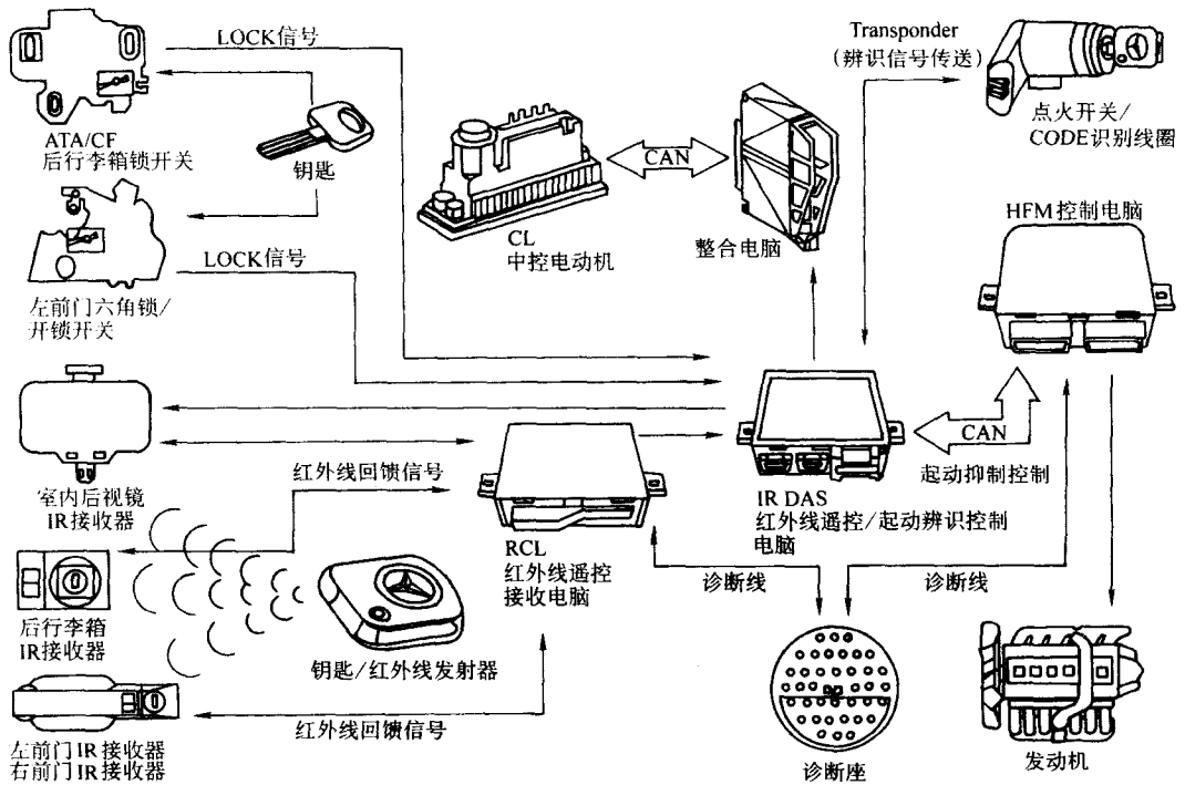
图 6-35 1997 年美规 W210 底盘中控防盗控制图
