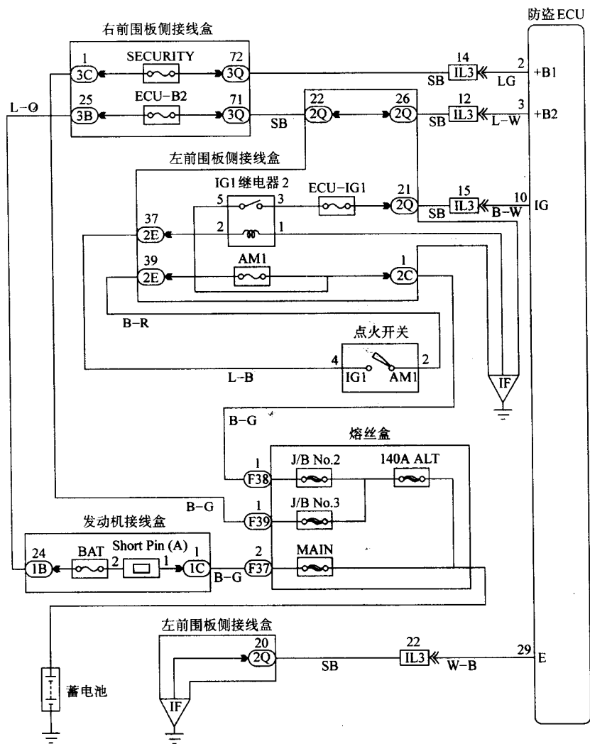
图 2-4 电源电路
