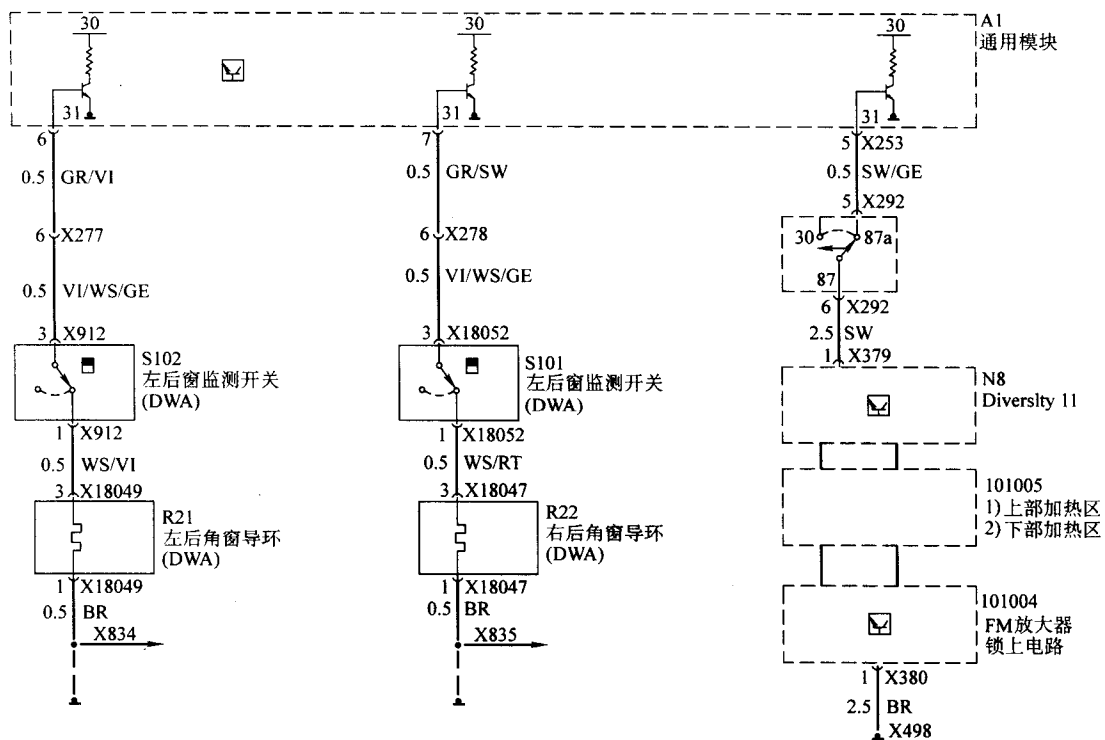
图 7-28 宝马 740i 和 750il (E38) 防盗系统后窗监测电路 (1996 年车型)
