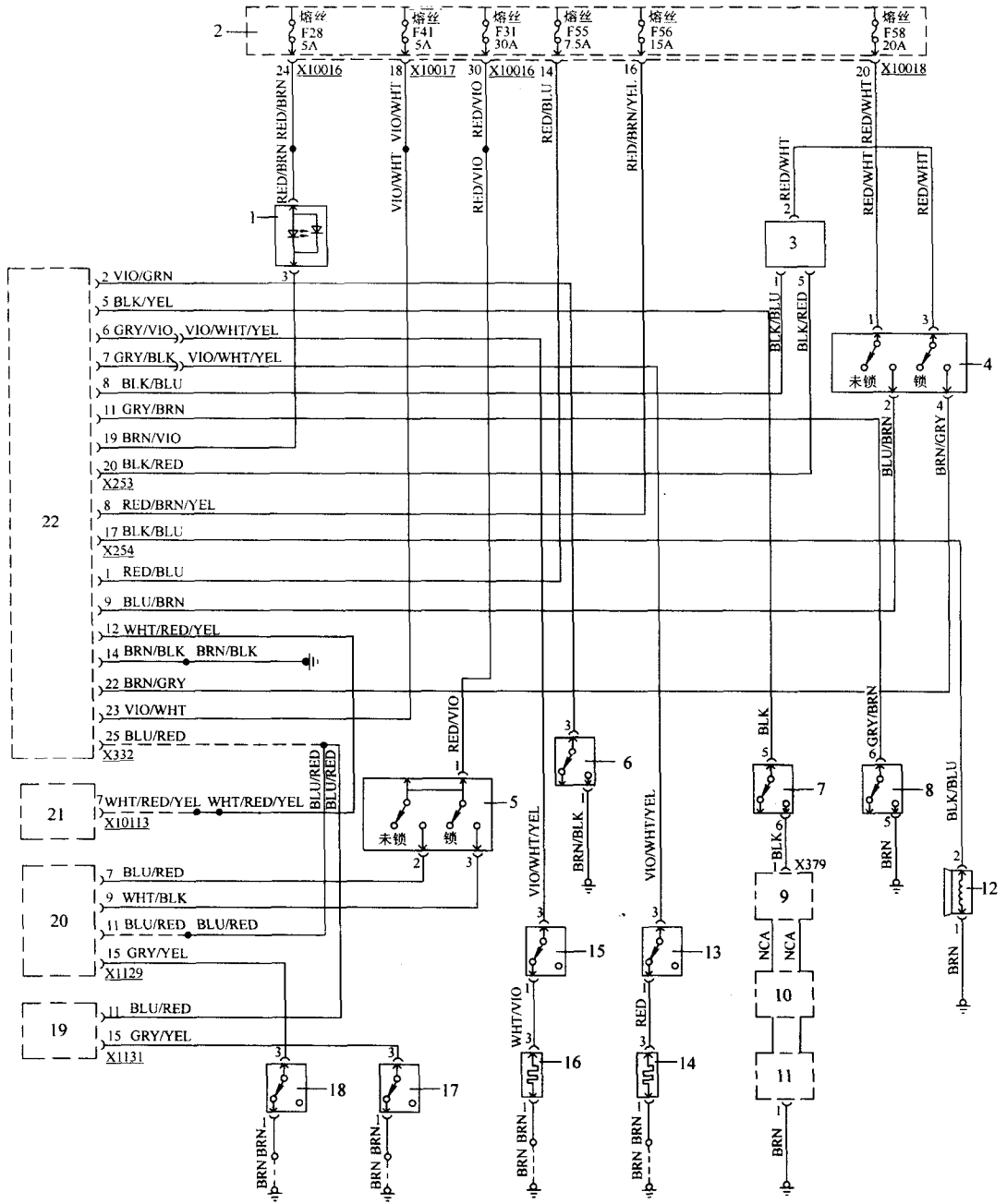
图 7-26 宝马 740i 和 740il 防盗系统电路 (1994 年车型)
