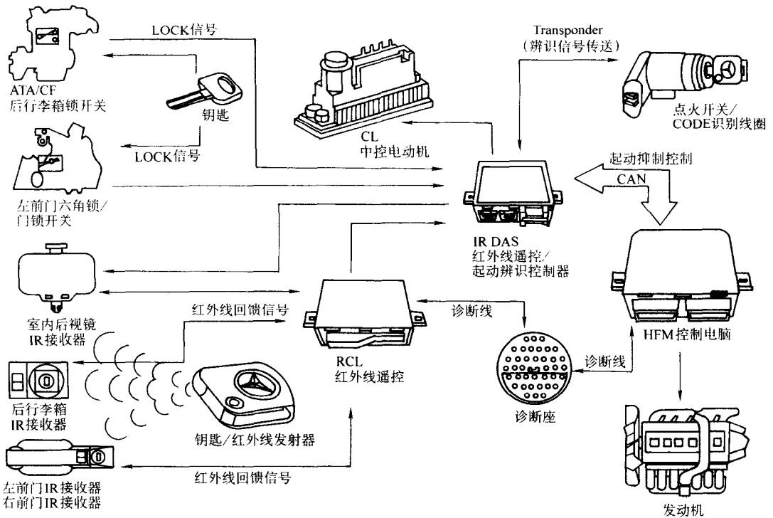
图 6-33 1997 年美规 W202 底盘中控防盗控制图
