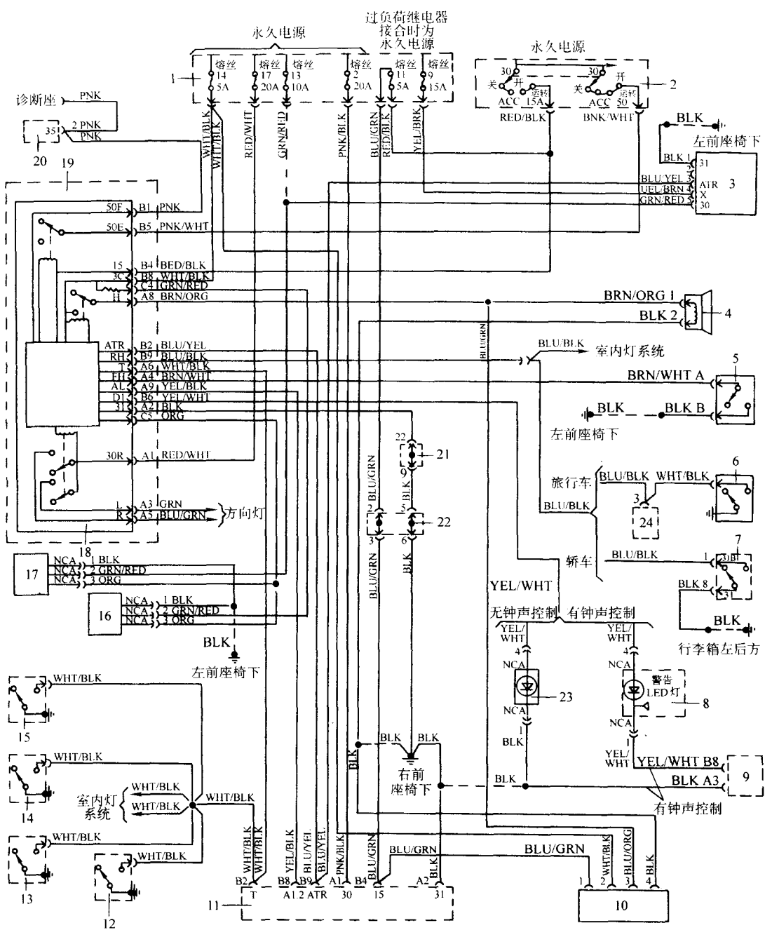
图 8-23 沃尔沃 960 Grand Alarm II 防盗系统电路
