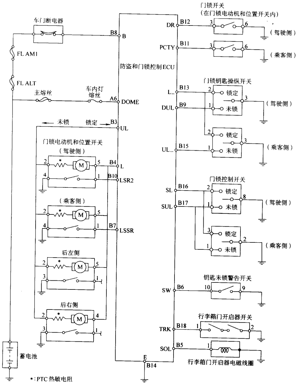
图 2-56 凌志 LS400 轿车中央门锁控制系统的电路
