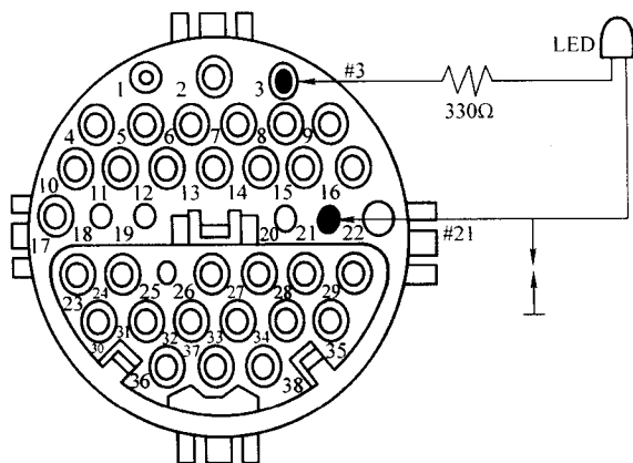
图 6-1 38 孔诊断座
