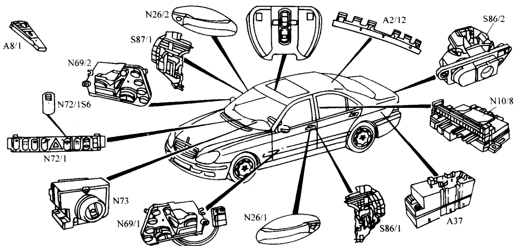
图 6-18 W220 底盘中控门锁元件位置
