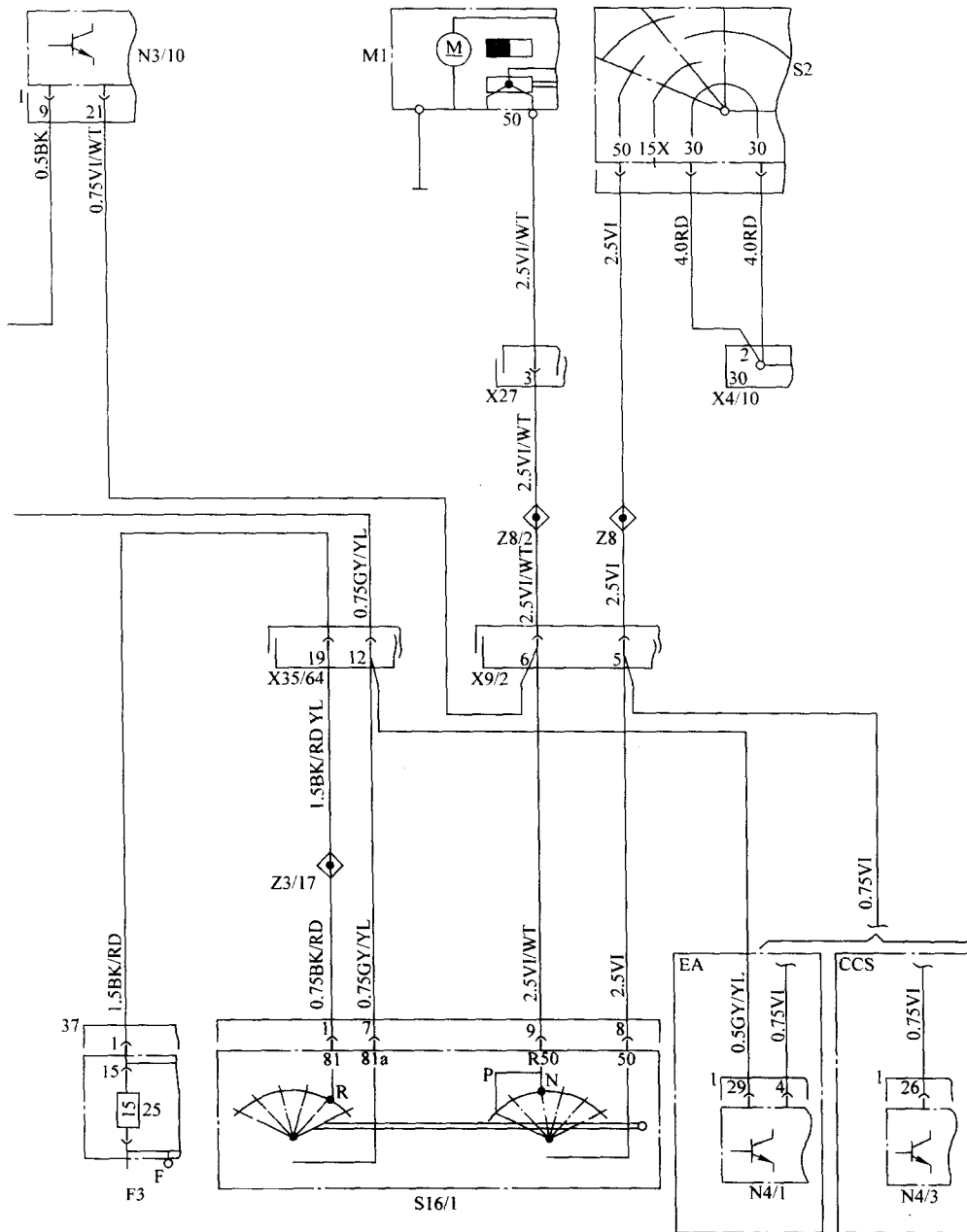
图 6-49 SL320 和 SL600 防盗报警系统电路图之四 (1997 车型)
