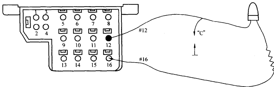
图 6-2 W129 中央门锁的故障码的读取与清除接线方法
