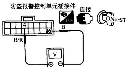
图 3-63 诊断步骤 6 流程
