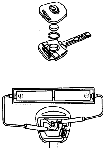
图 2-66 发射器的检查
