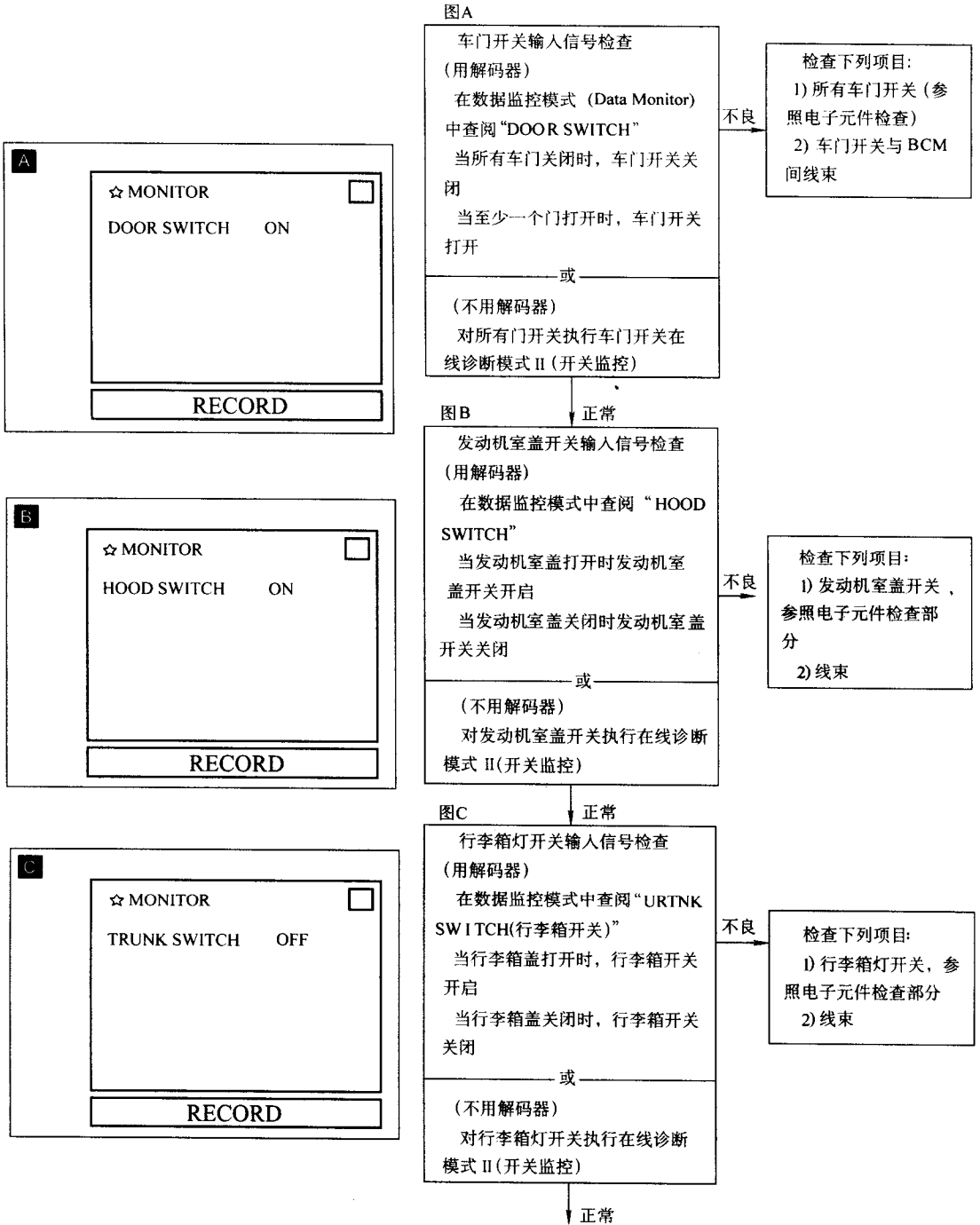
图 3-14 诊断程序 1
