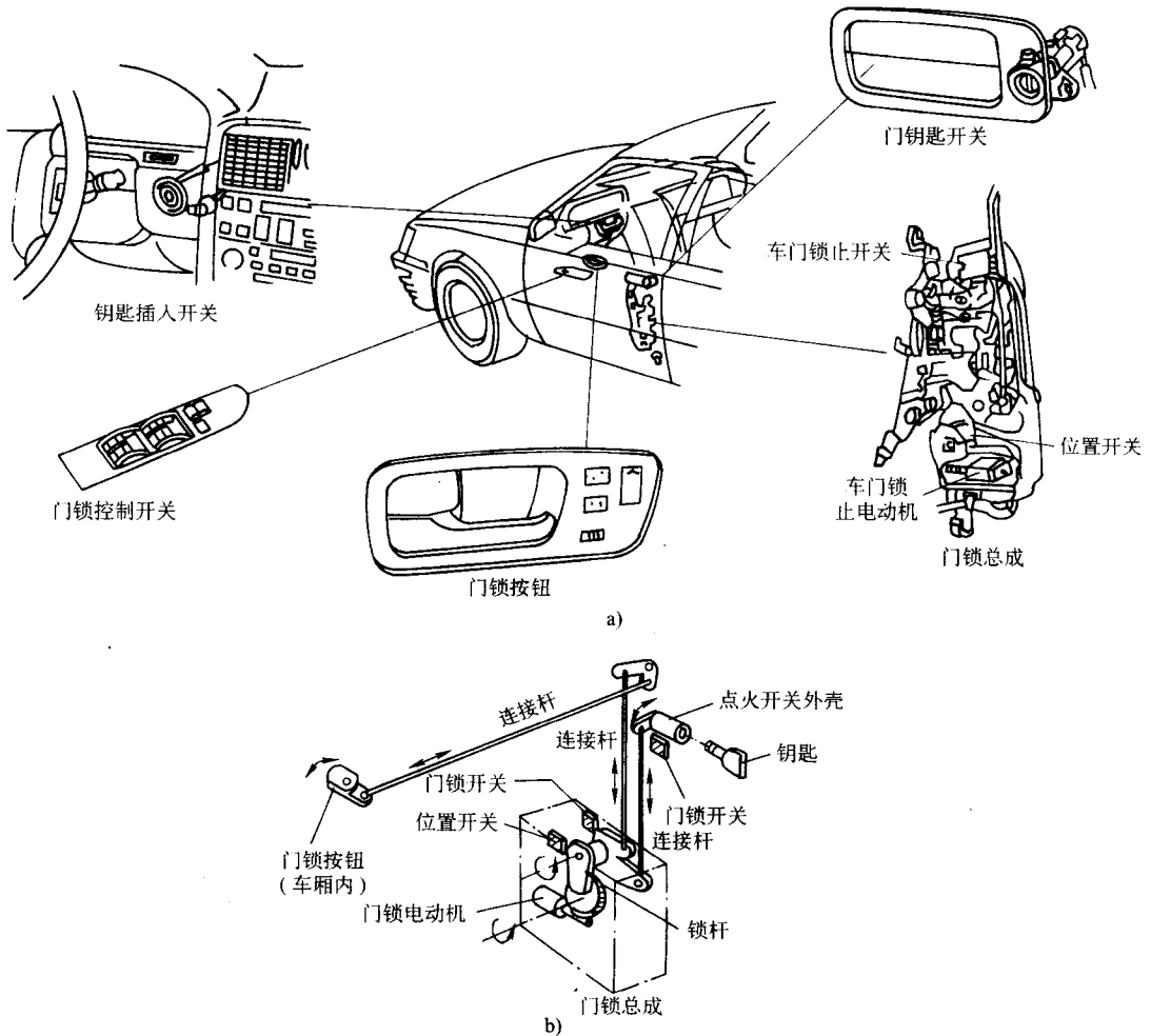
图 1-19 门锁机构
