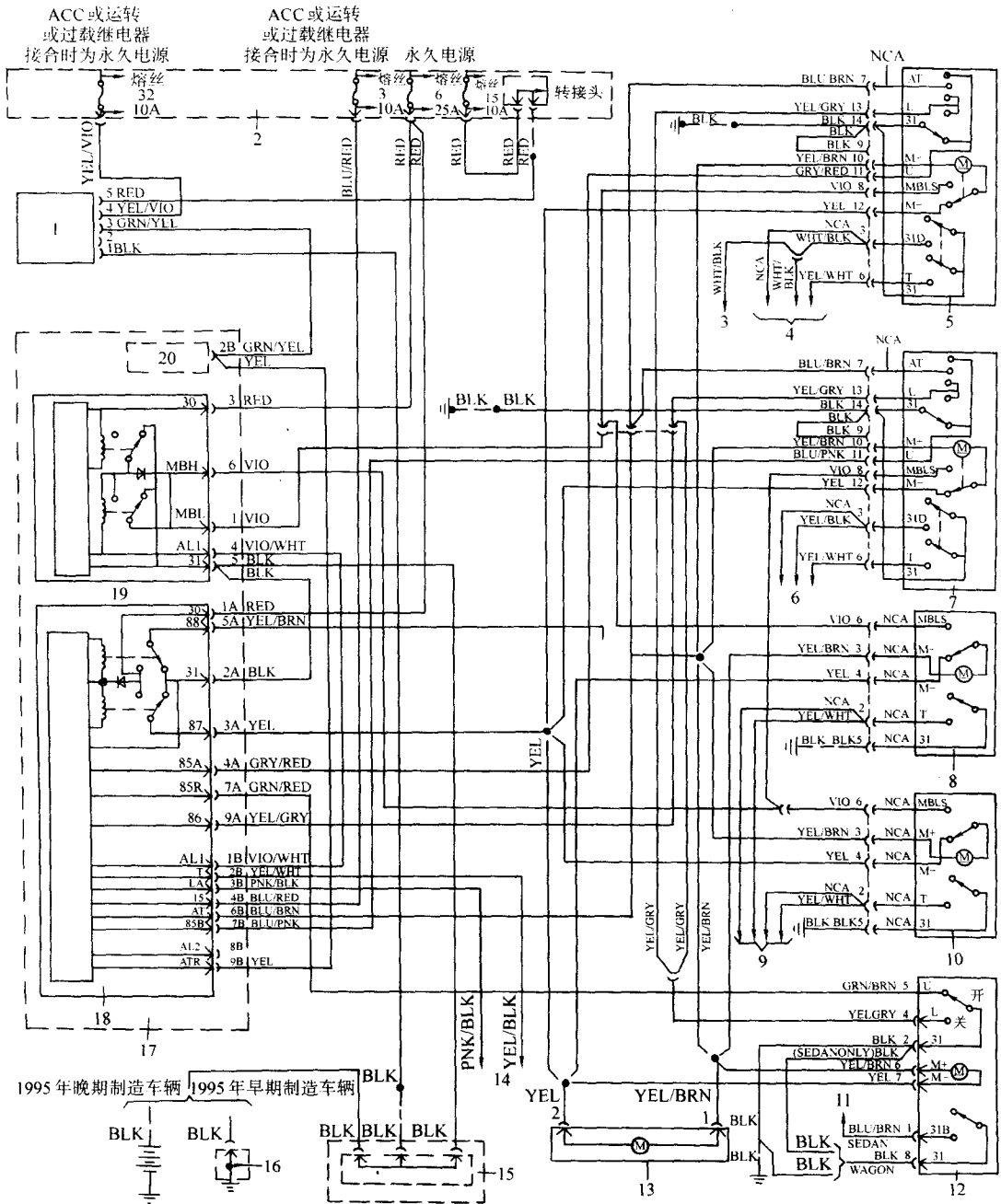
图 8-13 沃尔沃 850 中控遥控系统电路 (1995 年车型)
