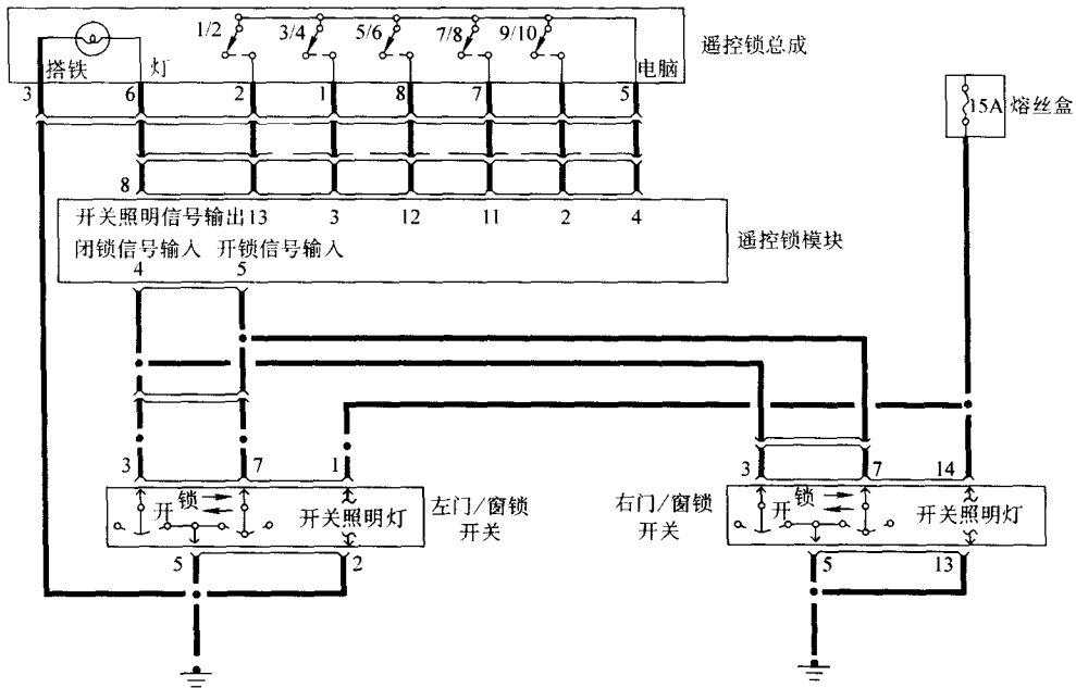
图 11-2 福特车系中央门锁及防盗系统电路
