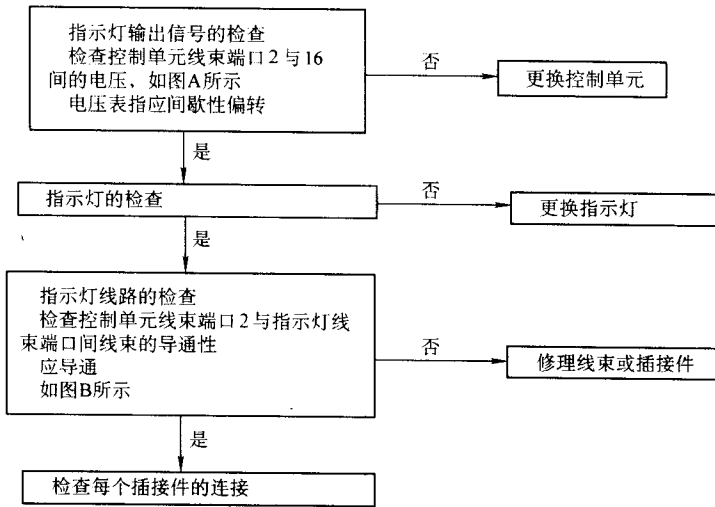
图 3-59 诊断步骤 2 流程
