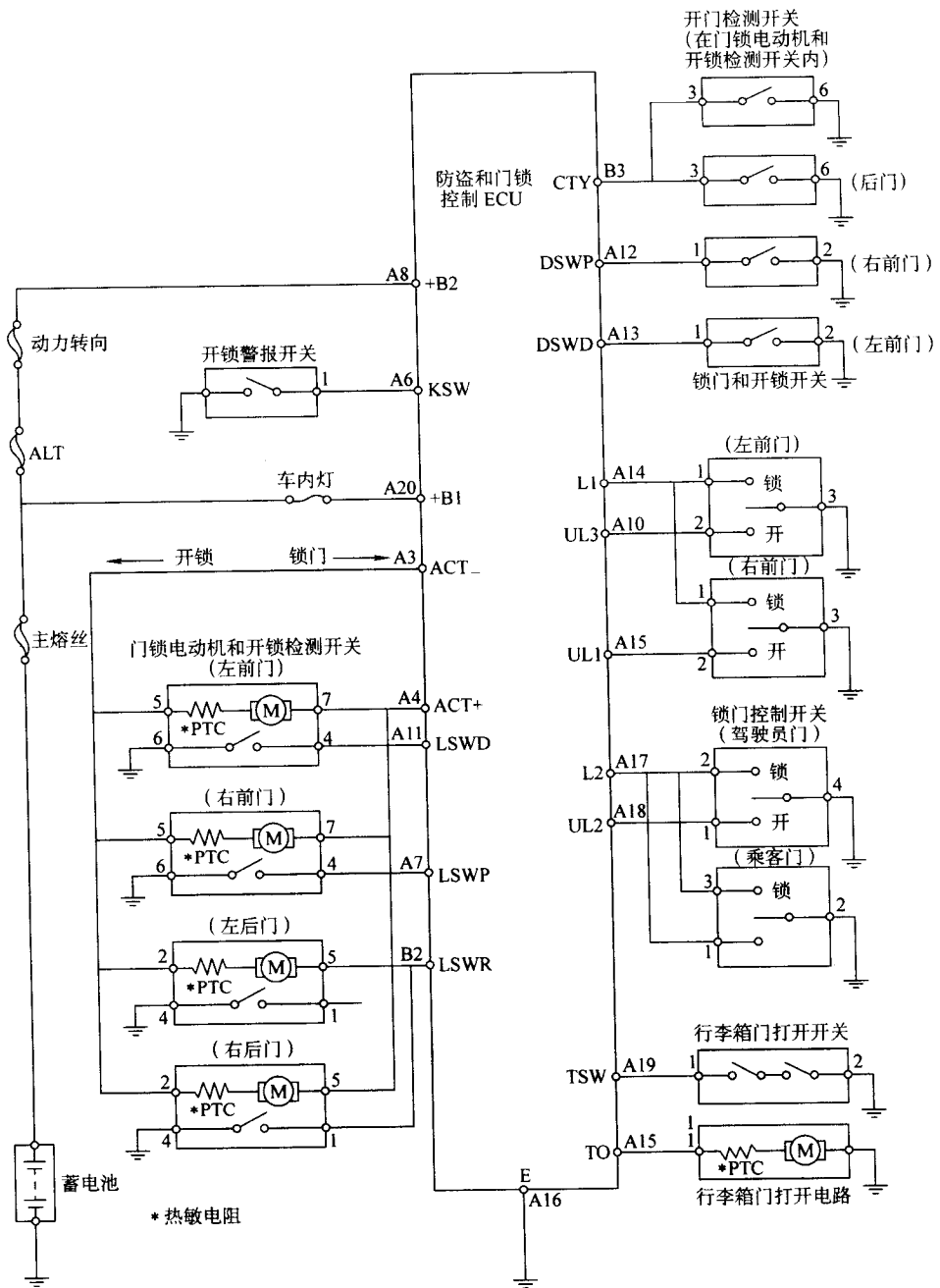
图 2-57 凌志 ES300 轿车中央门锁控制系统的电路
