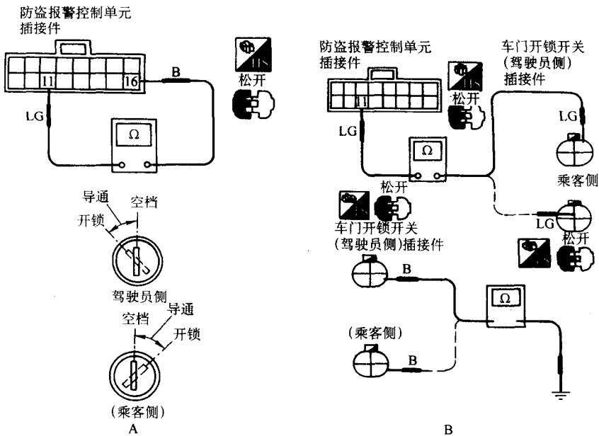
图 3-64 诊断步骤 7 流程
