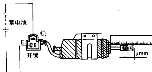
图 1-18 门锁电磁铁的检查
