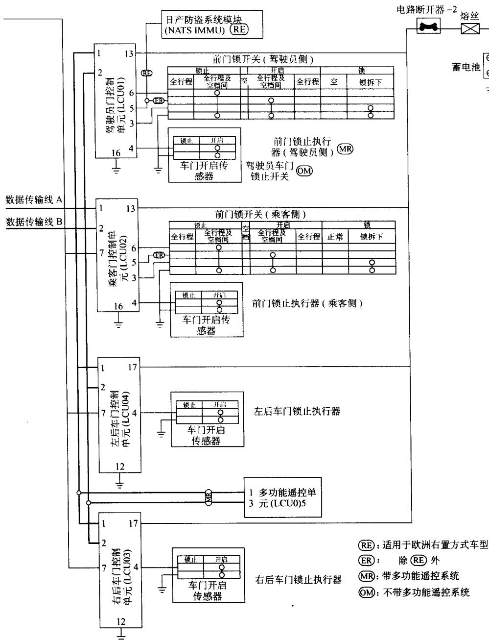
图 3-13 防盗系统原理
