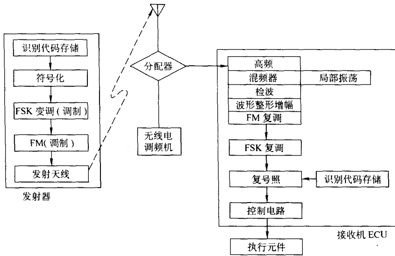
图 1-21 由微弱电波控制门锁用的发射器和接收器信号处理电路
