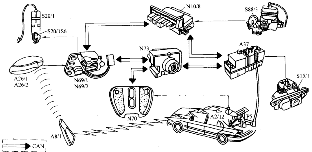
图 6-22 行李箱控制工作结构
