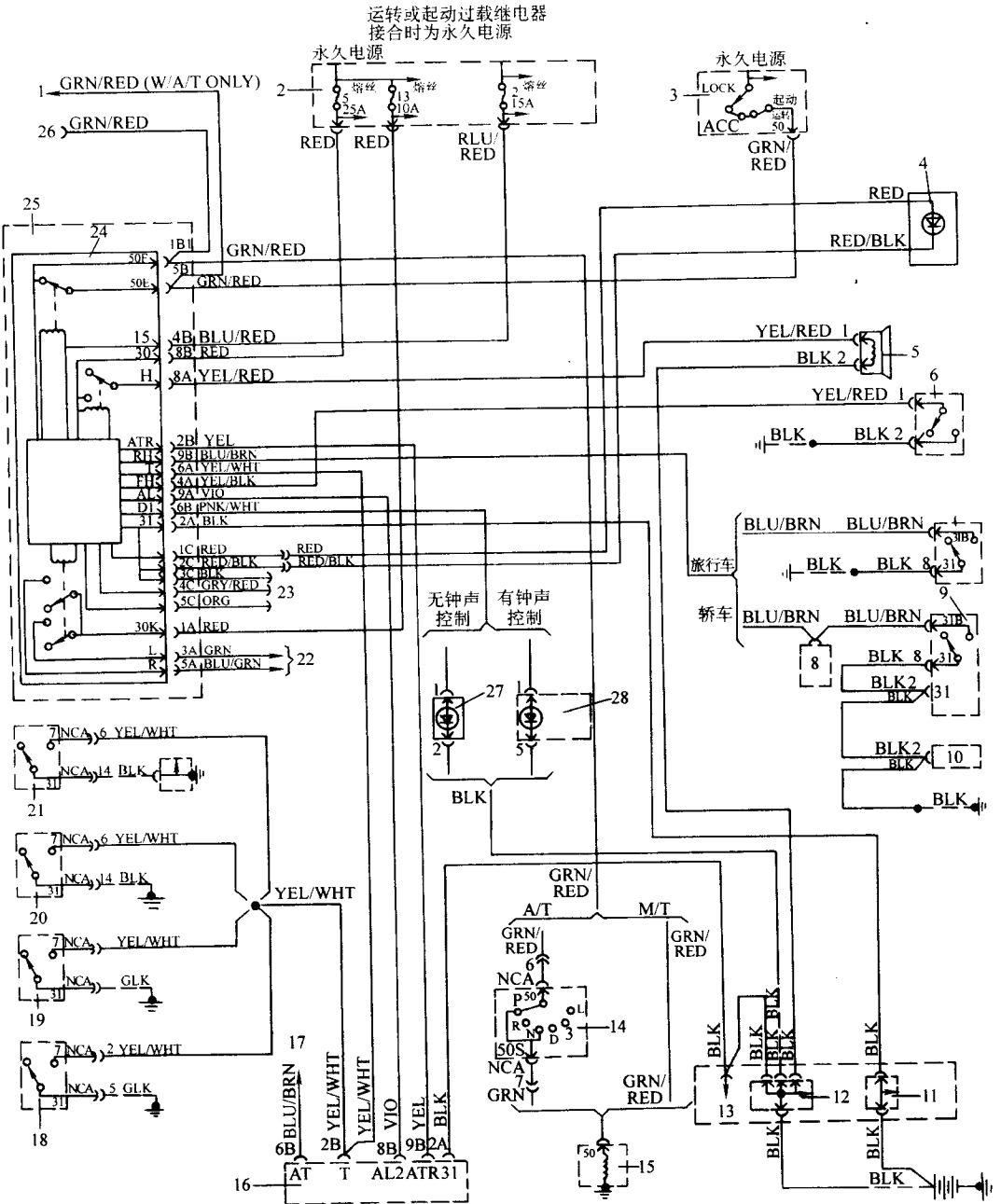
图 8-12 沃尔沃 850Grand Alarm II 防盗系统电路 (1995~1996 年车型)
