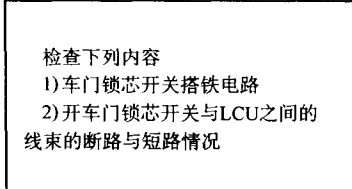
图 3-38 诊断步骤 4-1
