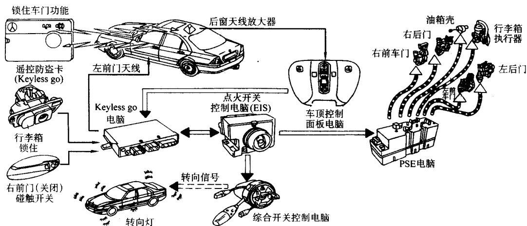
图 6-14 锁住车门工作流程
