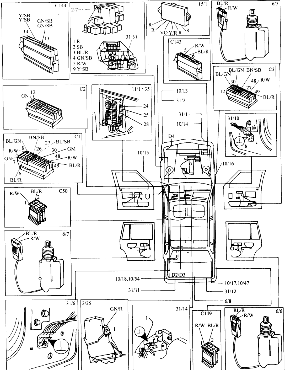
图 8-20 沃尔沃 960 中央门锁与防盗系统部件位置 (图注见图 8-19)
