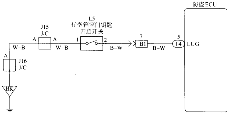
图 2-50 行李箱门钥匙锁止和开启开关电路
