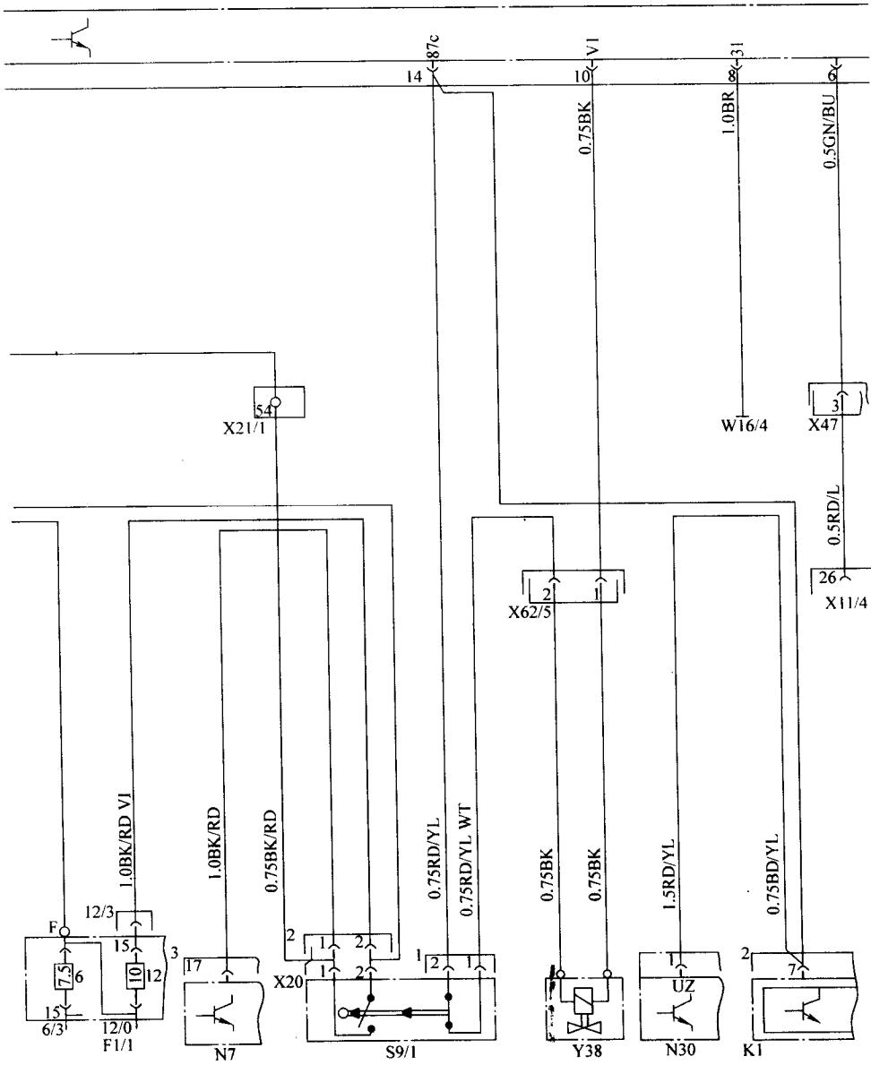
图 6-47 SL320 和 SL600 防盗报警系统电路图之二 (1997 车型)
