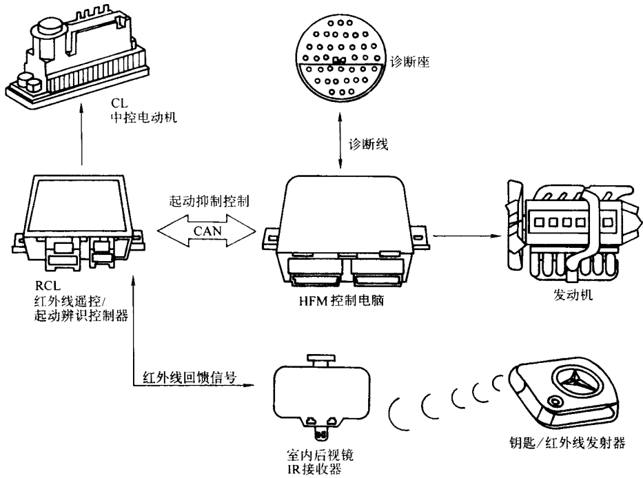
图 6-27 1996 年美规底盘 R129/W140/W202 中控防盗控制图
