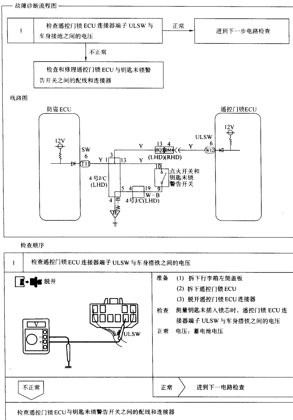
图 2-72 钥匙未锁警告开关电路检查
