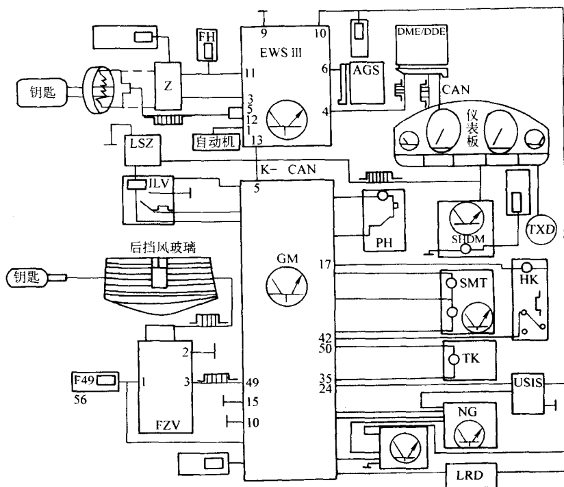
图 7-6 系统网络简图
