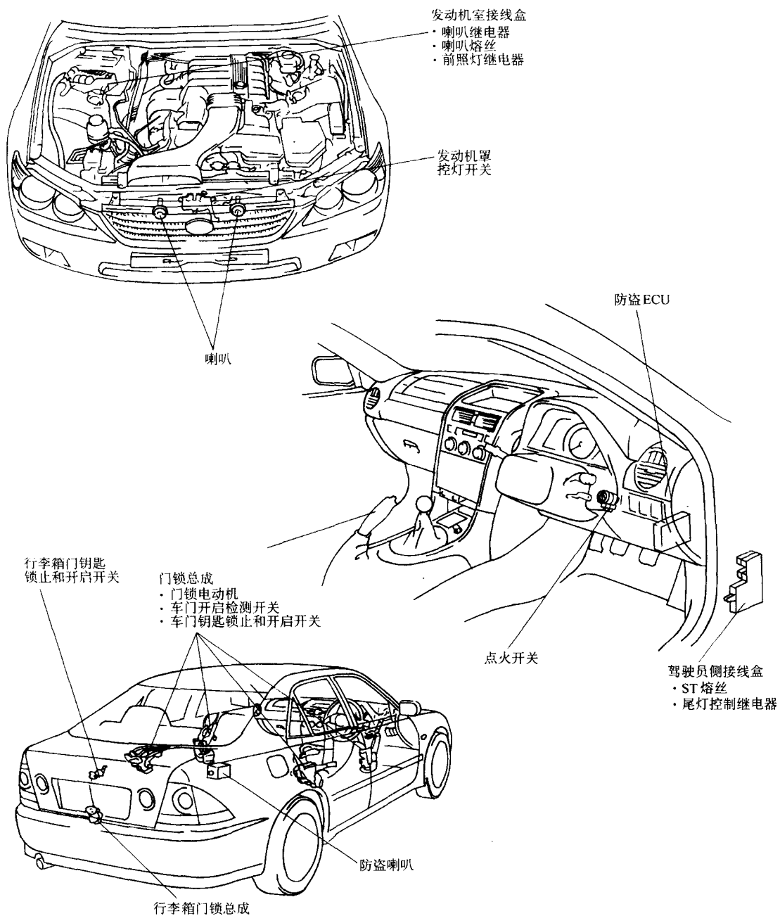
图 2-41 防盗系统电控元件位置
