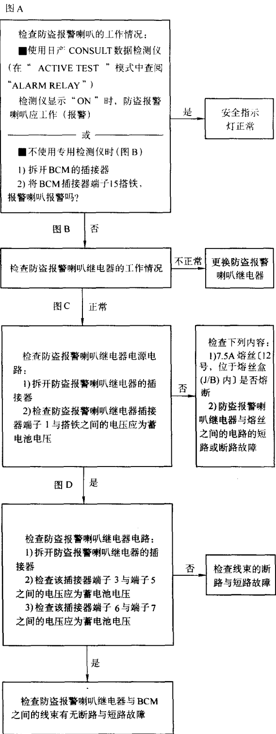
图 3-41 诊断步骤 6
