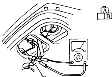
图 4-14 检查行李箱钥匙开关
