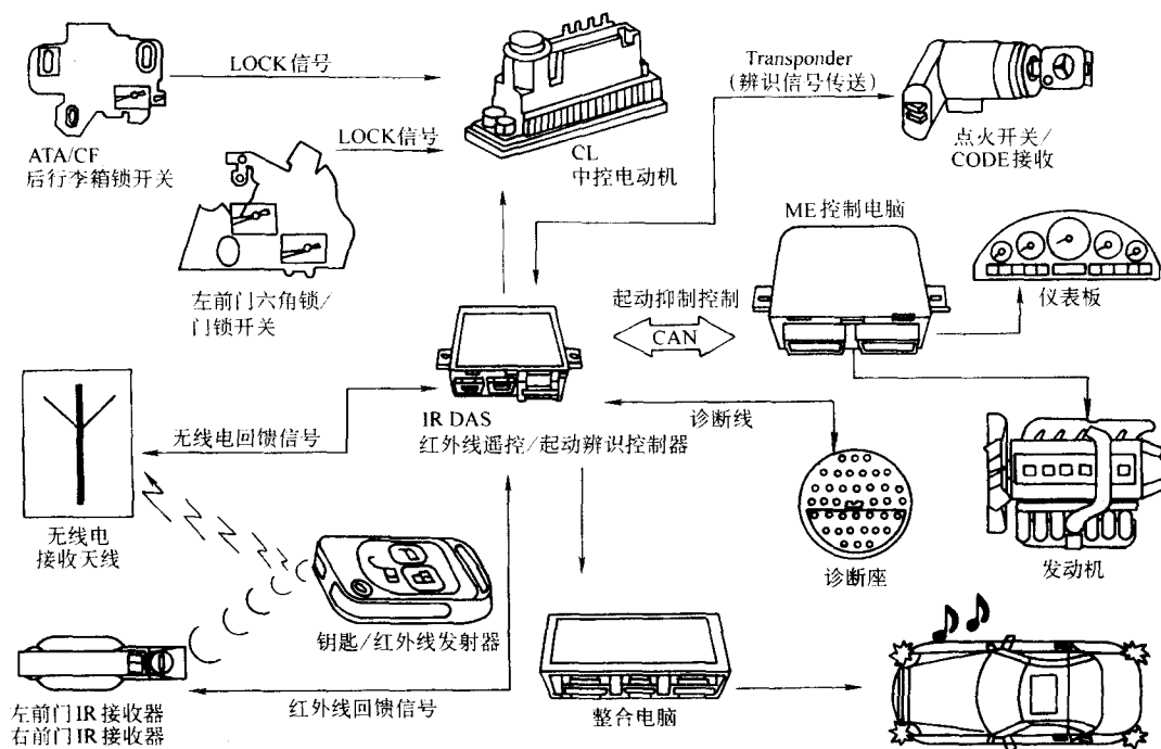
图 6-31 1998 年美规 W140 底盘中控防盗控制图
