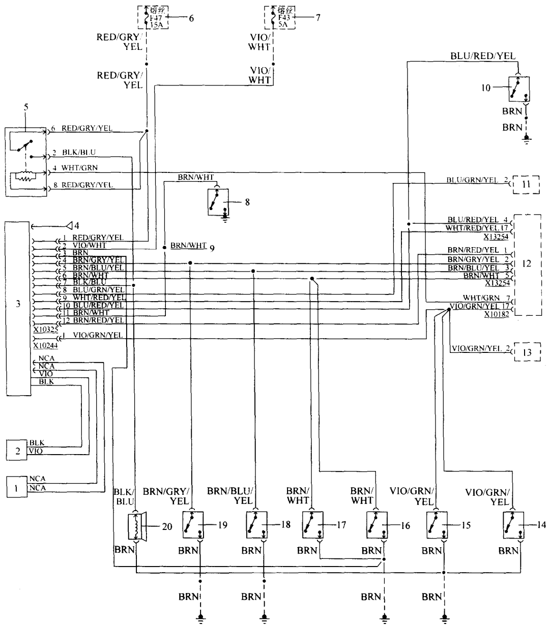
图 7-21 宝马 318i、318ic、318is、325i、325ic 和 325is 防盗系统电路 (1995 至 1996 年车型)
