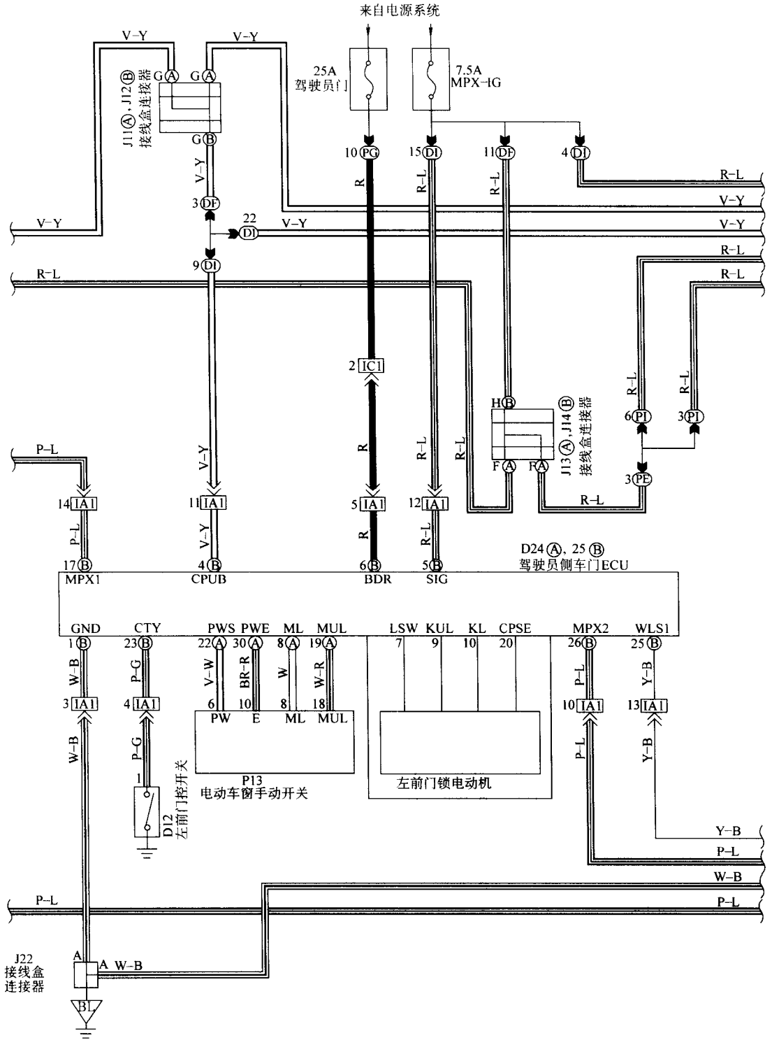
图 2-40 防盗系统 (不带智)
