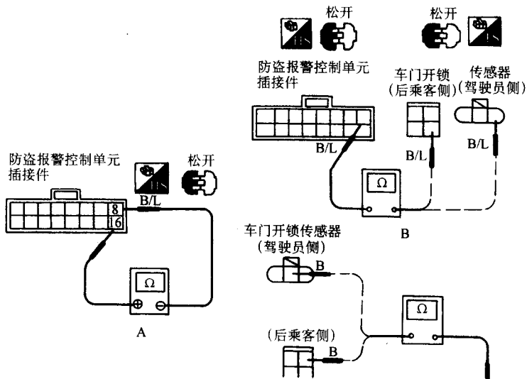
图 3-60 诊断步骤 3 流程
