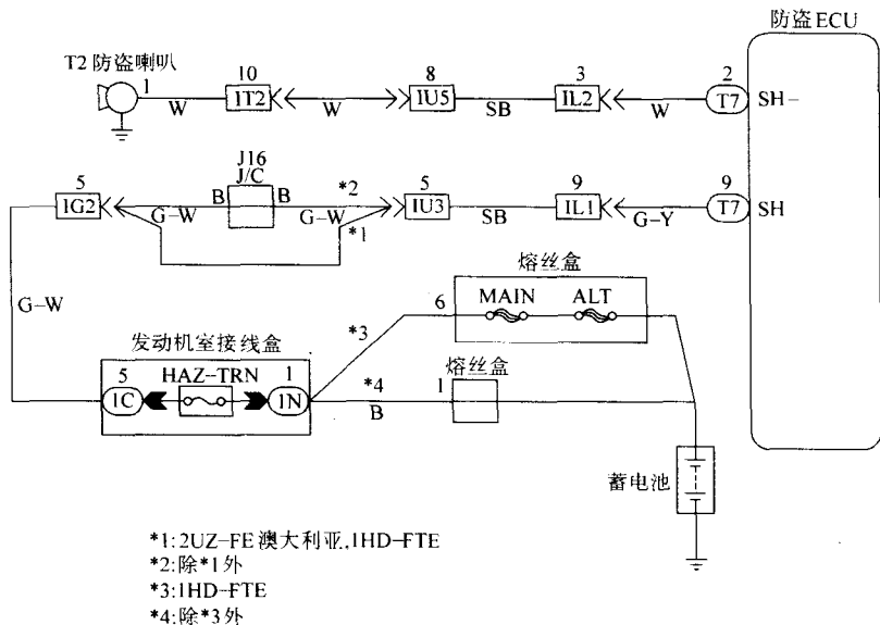
图 2-19 防盗喇叭电路
