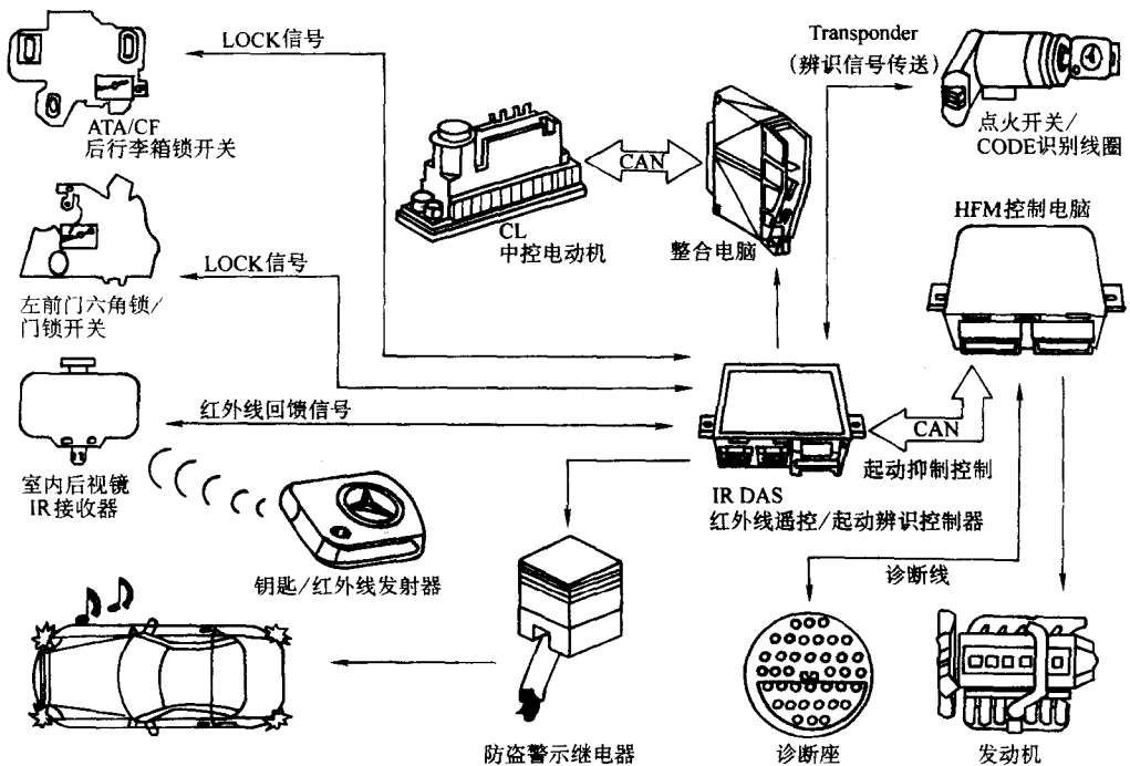
图 6-36 1996 年美规 W210 底盘中控防盗控制图
