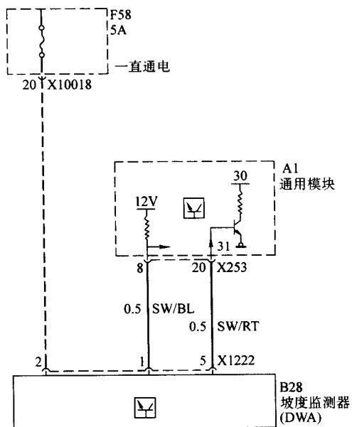
图 7-32 宝马 740i 和 750il (E38) 防盗系统倾斜传感器电路 (1996 年车型)
