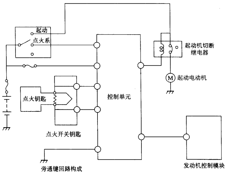
图 1-12 防止被盗车辆移动装置的基本构成
