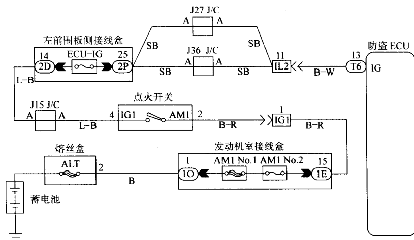
图 2-13 点火开关电路
