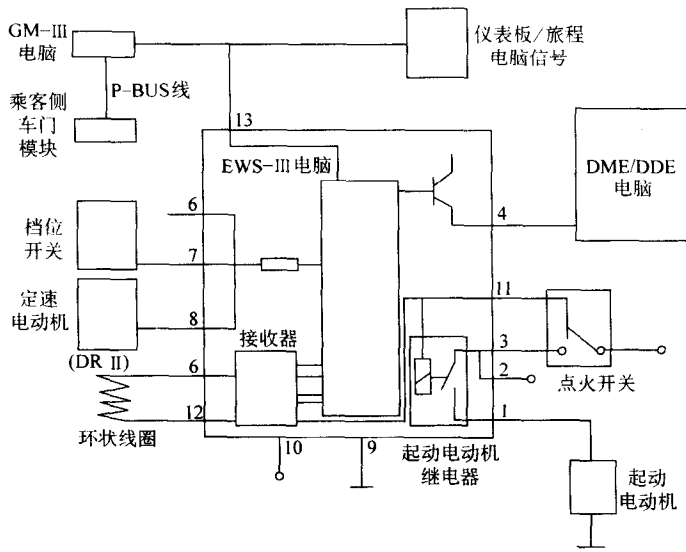
图 7-13 EWS-III 系统示意图
