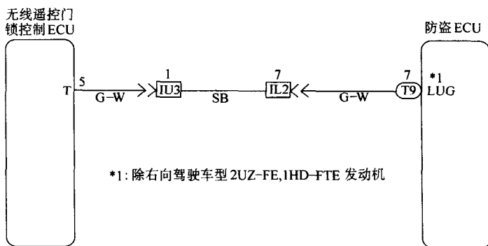
图 2-18 行李箱门钥匙锁止和开启开关电路
