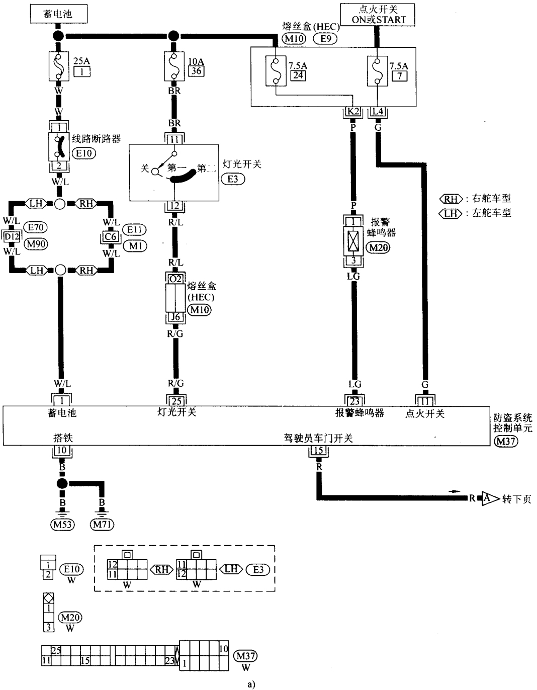
图 3-48 带电动车门锁型的蜂鸣器控制电路
