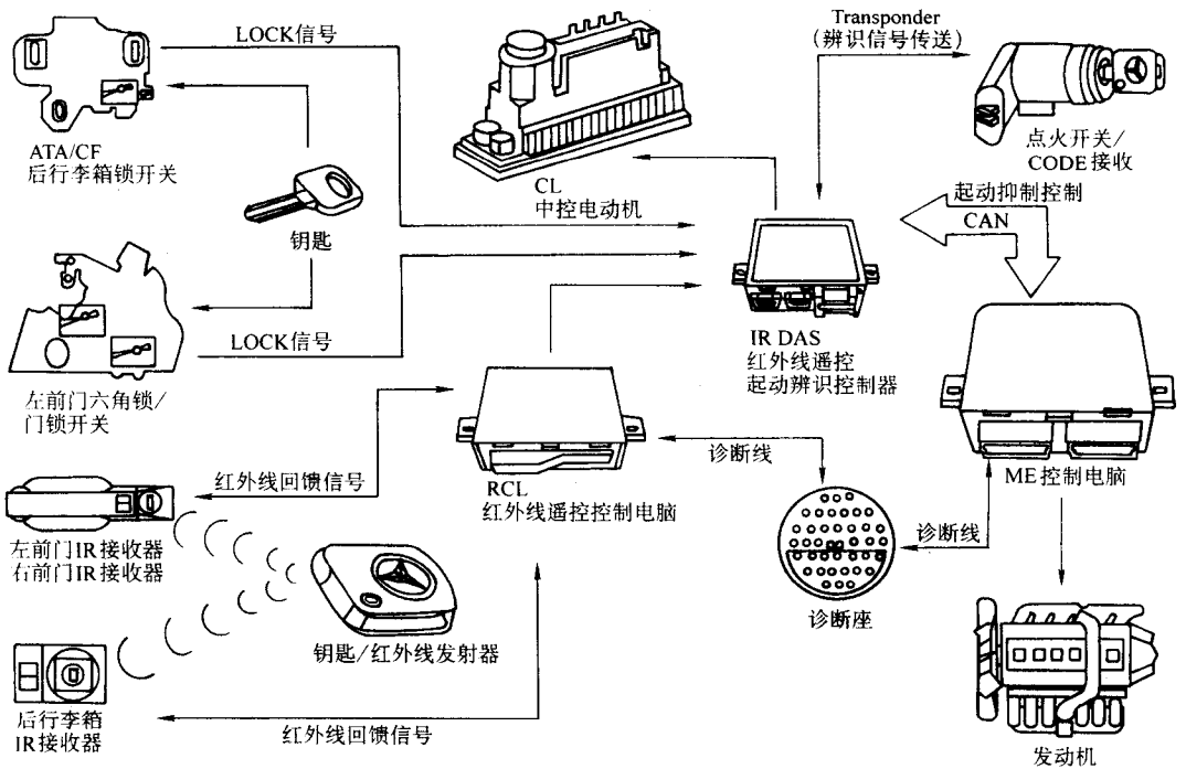
图 6-30 1997 年美规 W140 底盘中控防盗控制图
