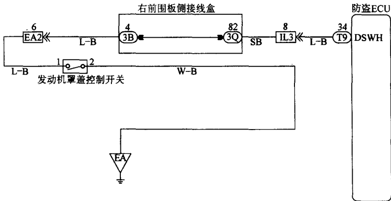
图 2-8 发动机室盖控制开关电路
