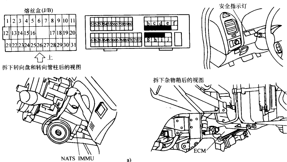
图 3-1 NATS 主要部件布置及控制原理
