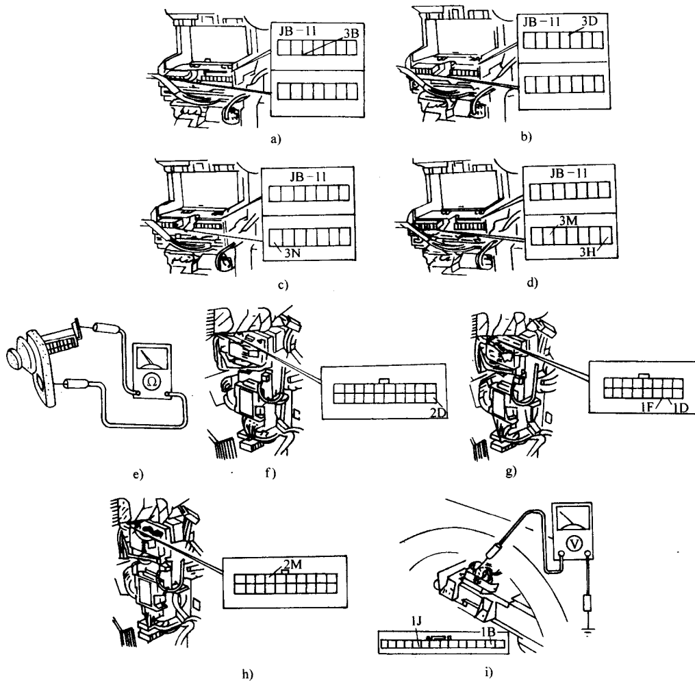
图 4-4 预警 1: 安全灯不亮、蜂鸣器不响的故障排除
