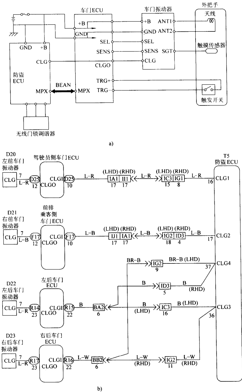
图 2-35 车门振动电路
