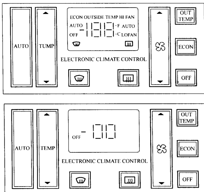
图 10-8 空调面板
