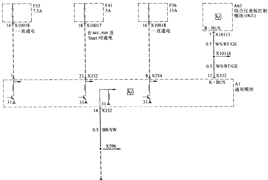
图 7-31 宝马 740i 和 750il (E38) 防盗系统电源及 K-BUS 电路 (1996 年车型)
