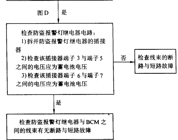
图 3-42 诊断步骤 7
