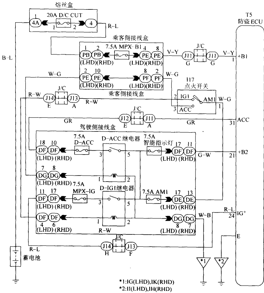
图 2-28 电源电路
