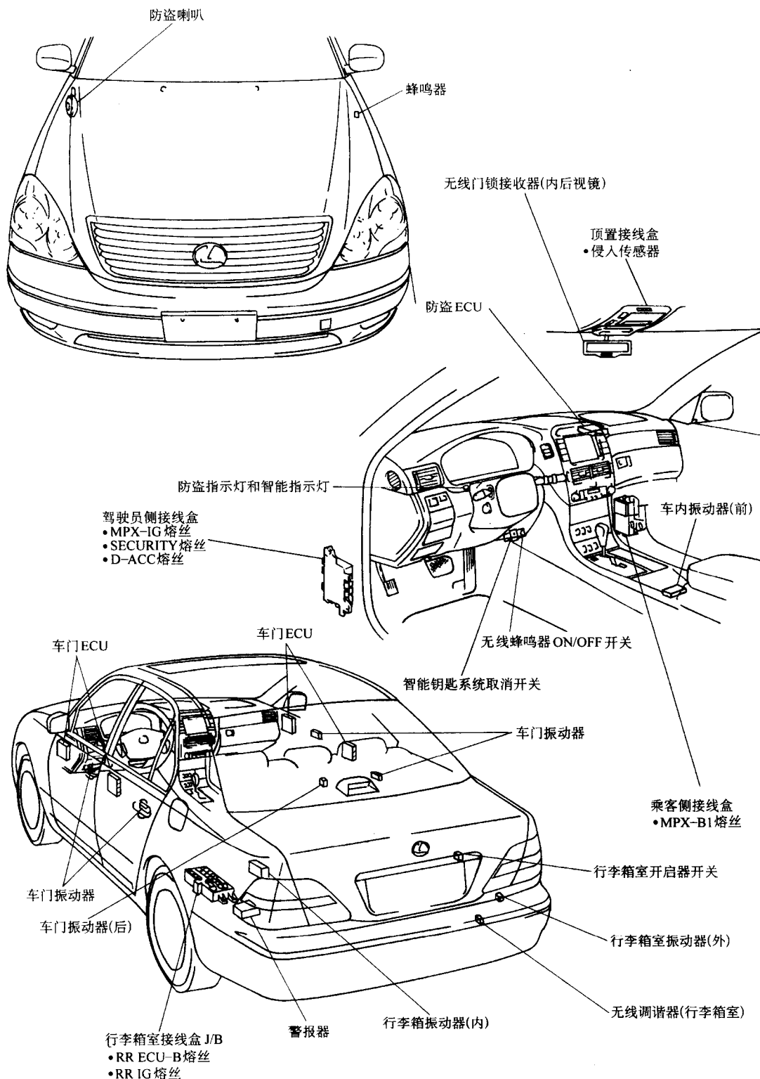
图 2-25 防盗系统电控元件位置
