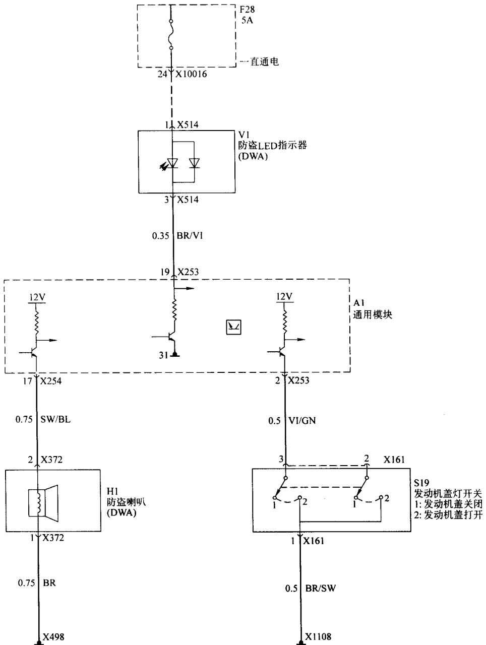
图 7-30 宝马 740i 和 750iL (E38) 防盗系统发动机盖开关、DMA-LED 及喇叭电路 (1996 年车型)
