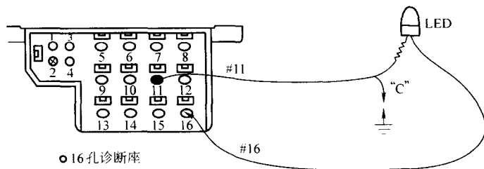
图 6-4 16 孔诊断座
