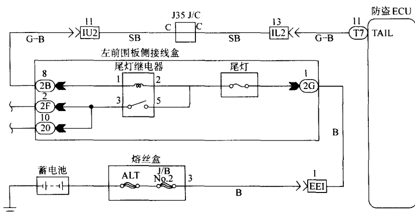
图 2-16 尾灯控制继电器电路
