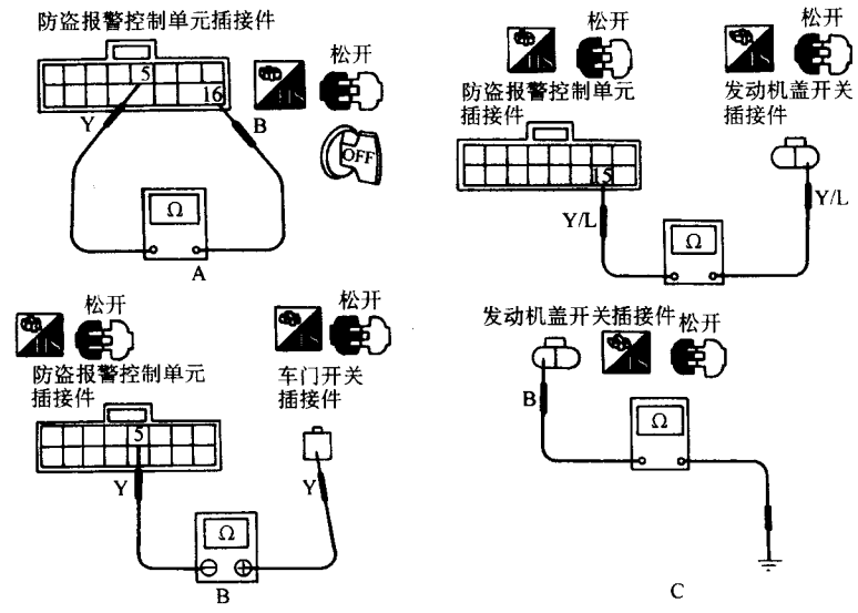
图 3-58 诊断步骤 1 流程
