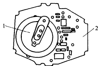
图 7-5 防盗钥匙晶片（另一侧）
