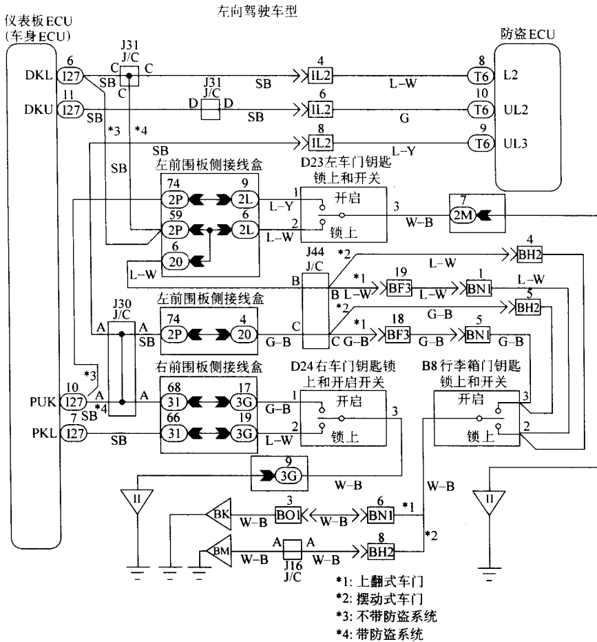
图 2-21 车门钥匙锁止和开启开关的电路
