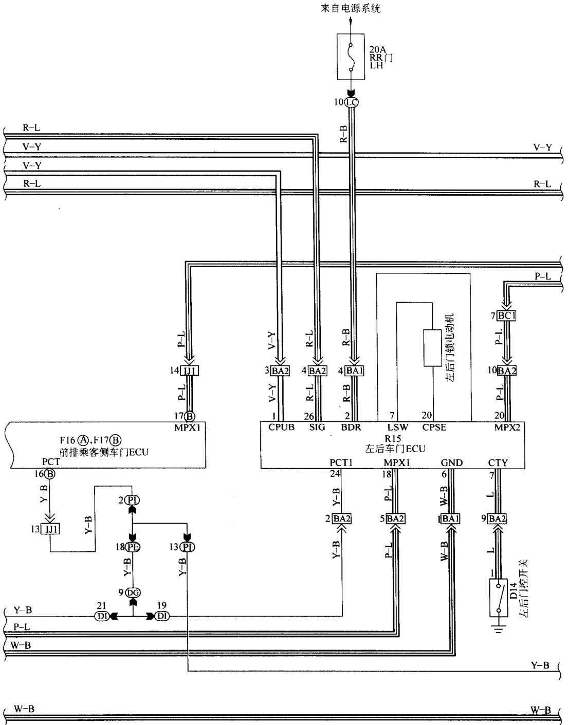
图 2-40 防盗系统 (不带智)
