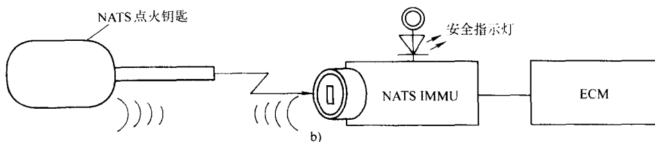
图 3-1 NATS 主要部件布置及控制原理 (续)
