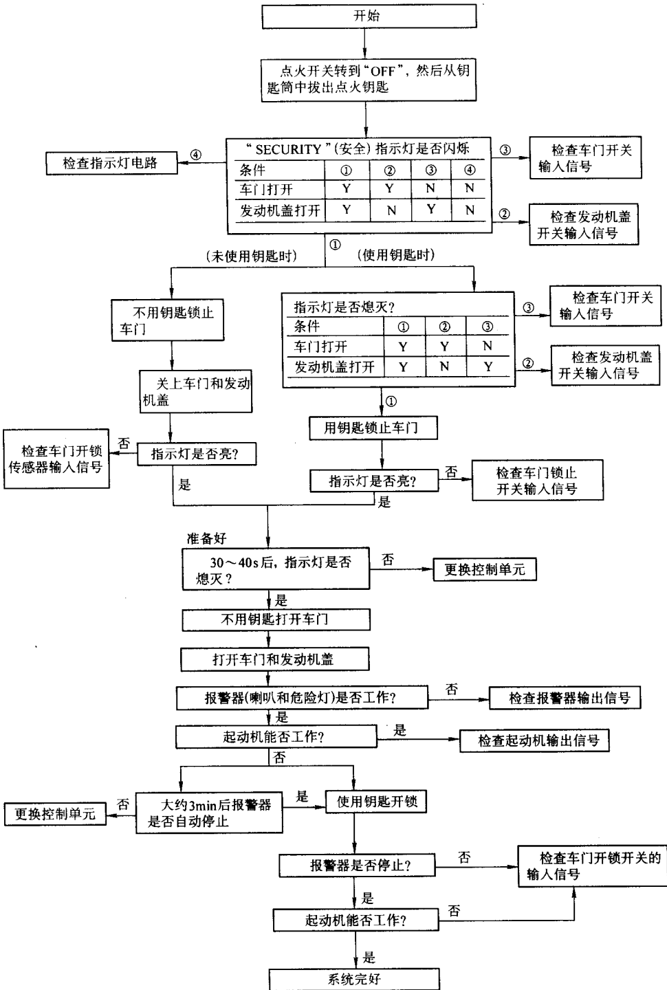
图 3-54 日产风度防盗系统故障框图
