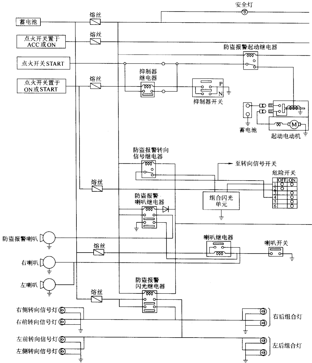
图 3-55 日产风度防盗系统故障诊断速查电路
