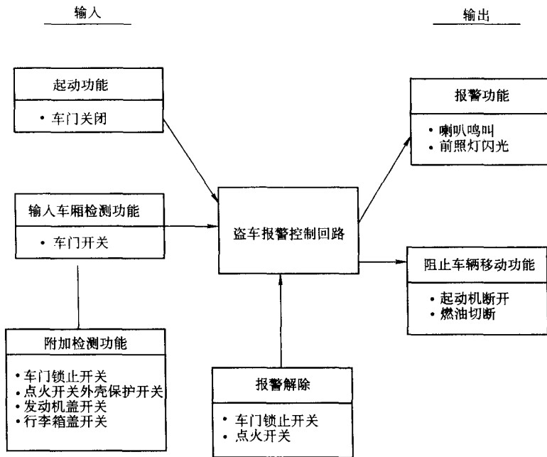
图 1-8 防盗装置的功能构成
