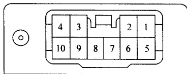
图 2-63 无线电遥控系统 ECU 的端子
