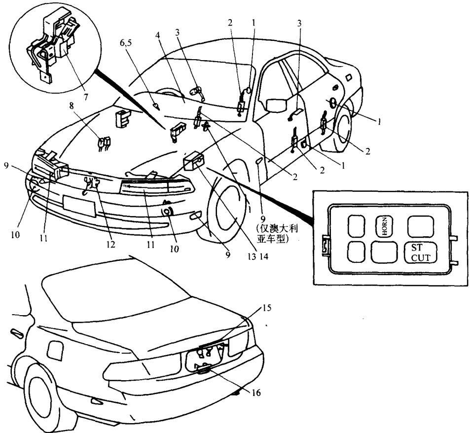
图 4-1 马自达 929 防盗系统元件位置
