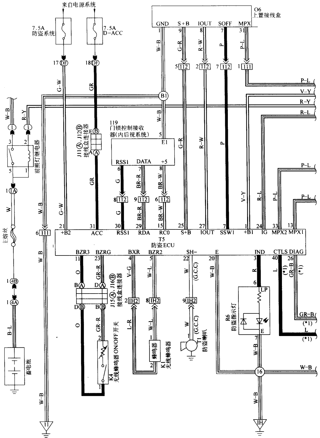
图 2-40 防盗系统（不带智能钥匙系统）电路
