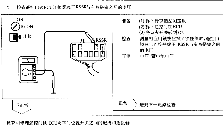
图 2-69 车门开关电路检查 (续)
