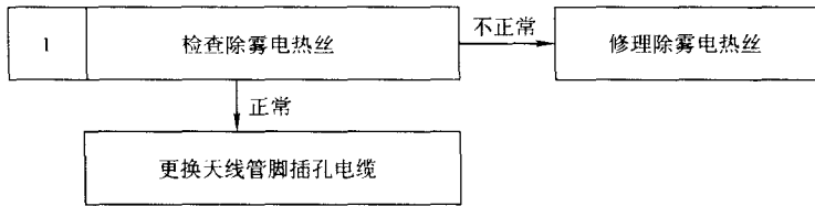
线路图
