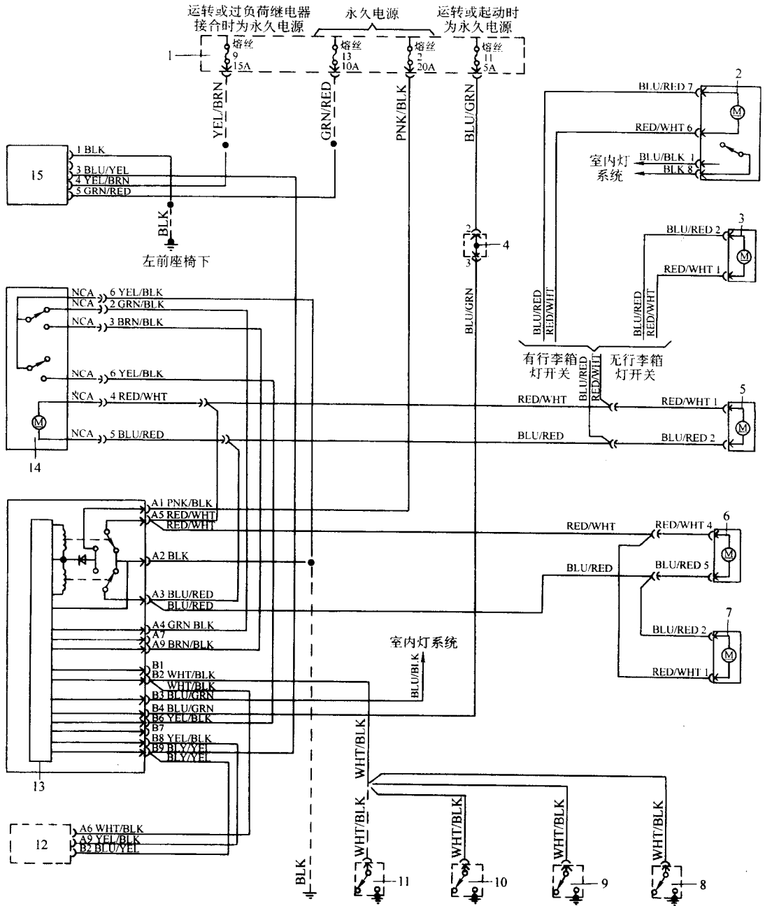
图 8-25 沃尔沃 960 遥控中控系统电路 (1995 年车型)
