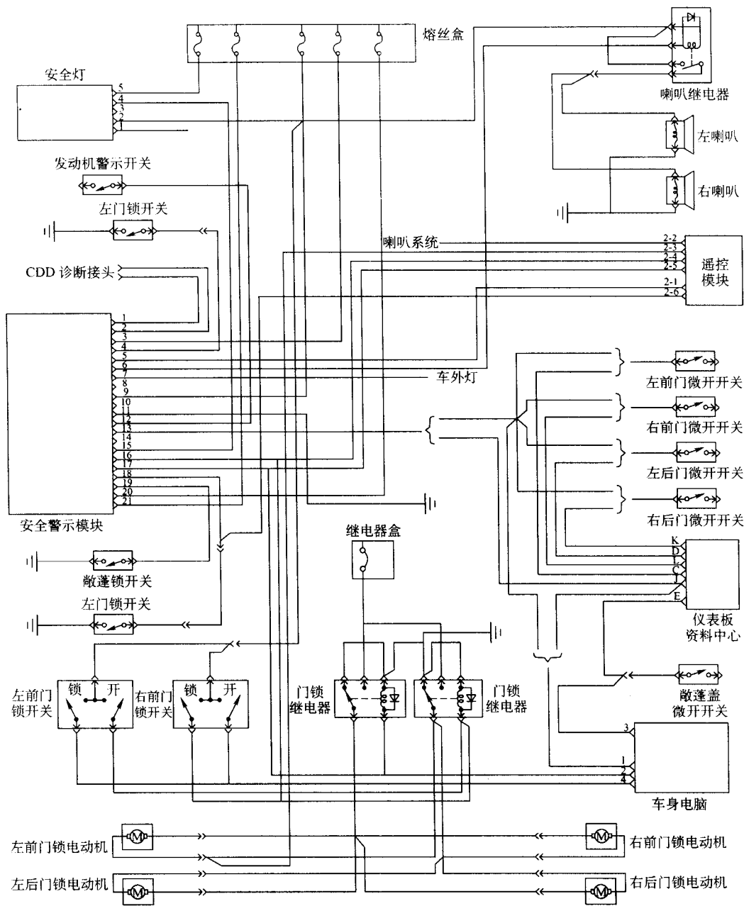
图 1-3 美国克莱斯勒帝王 (Imperial) 的防盗电路图
