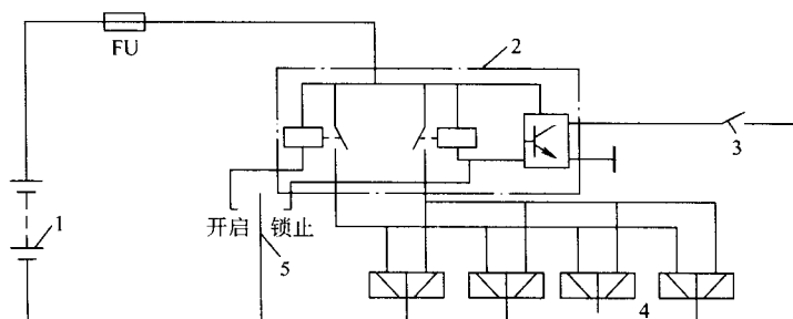
图 1-17 电控门锁电路
