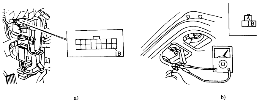
图 4-11 用钥匙打开行李箱、报警不停止的故障排除
