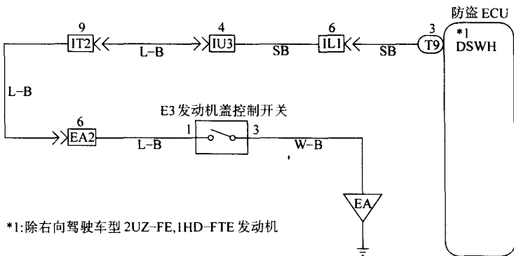
图 2-20 发动机室盖控制开关电路
