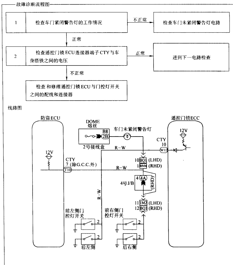
图 2-73 门控灯开关电路
