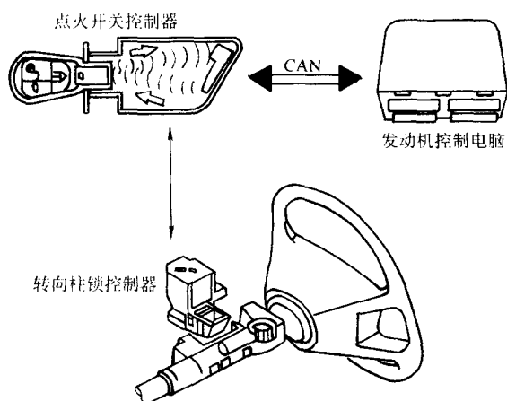
图 6-39 发动机控制电脑与转向柱锁控制器之间的通信
