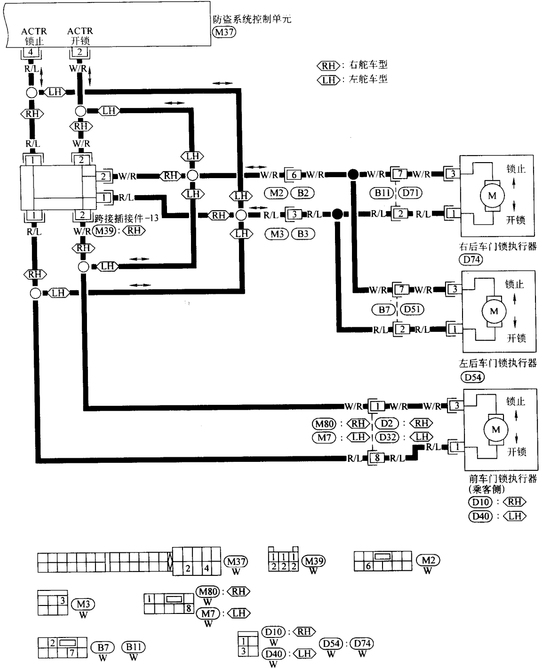
图 3-47 车门锁控制电路 (续)
