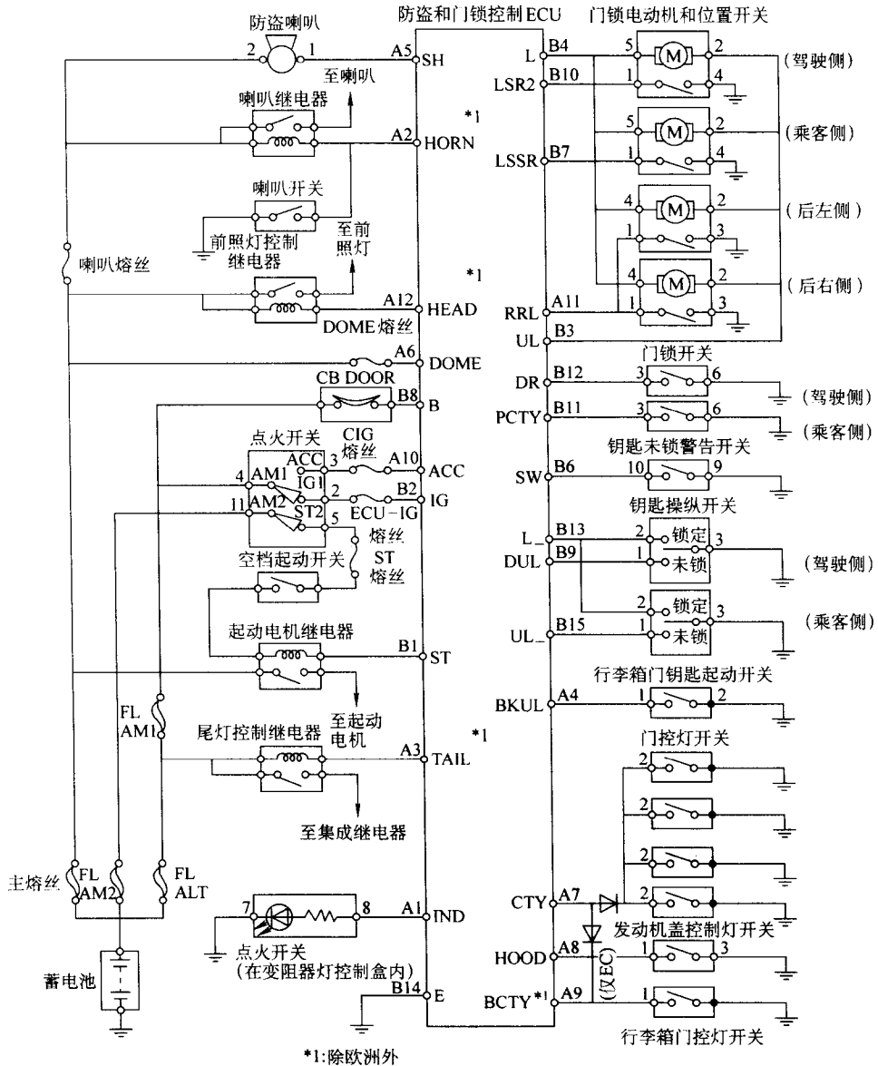
图 2-59 丰田凌志 LS400 与 ES300 防盗系统的电路
