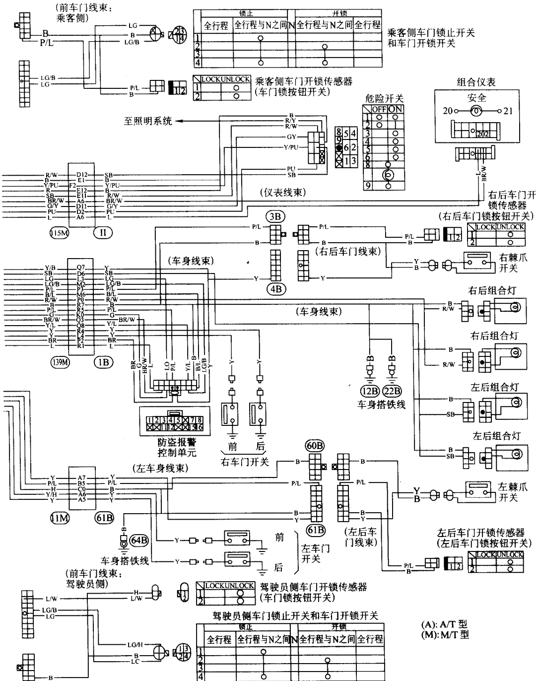
图 3-53 日产风度防盗系统电路
