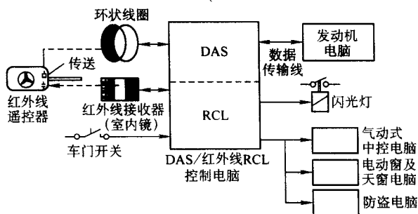
图 6-8 DAS2a/2b 工作示意图
