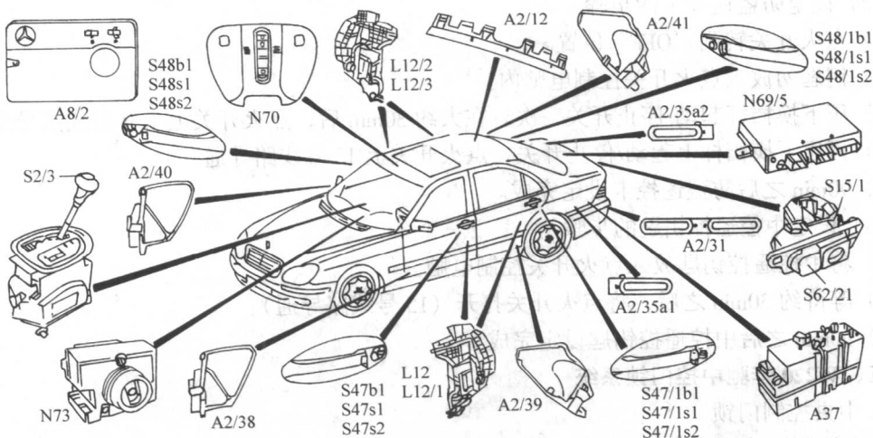
图 6-17 Keyless go 系统元件位置
