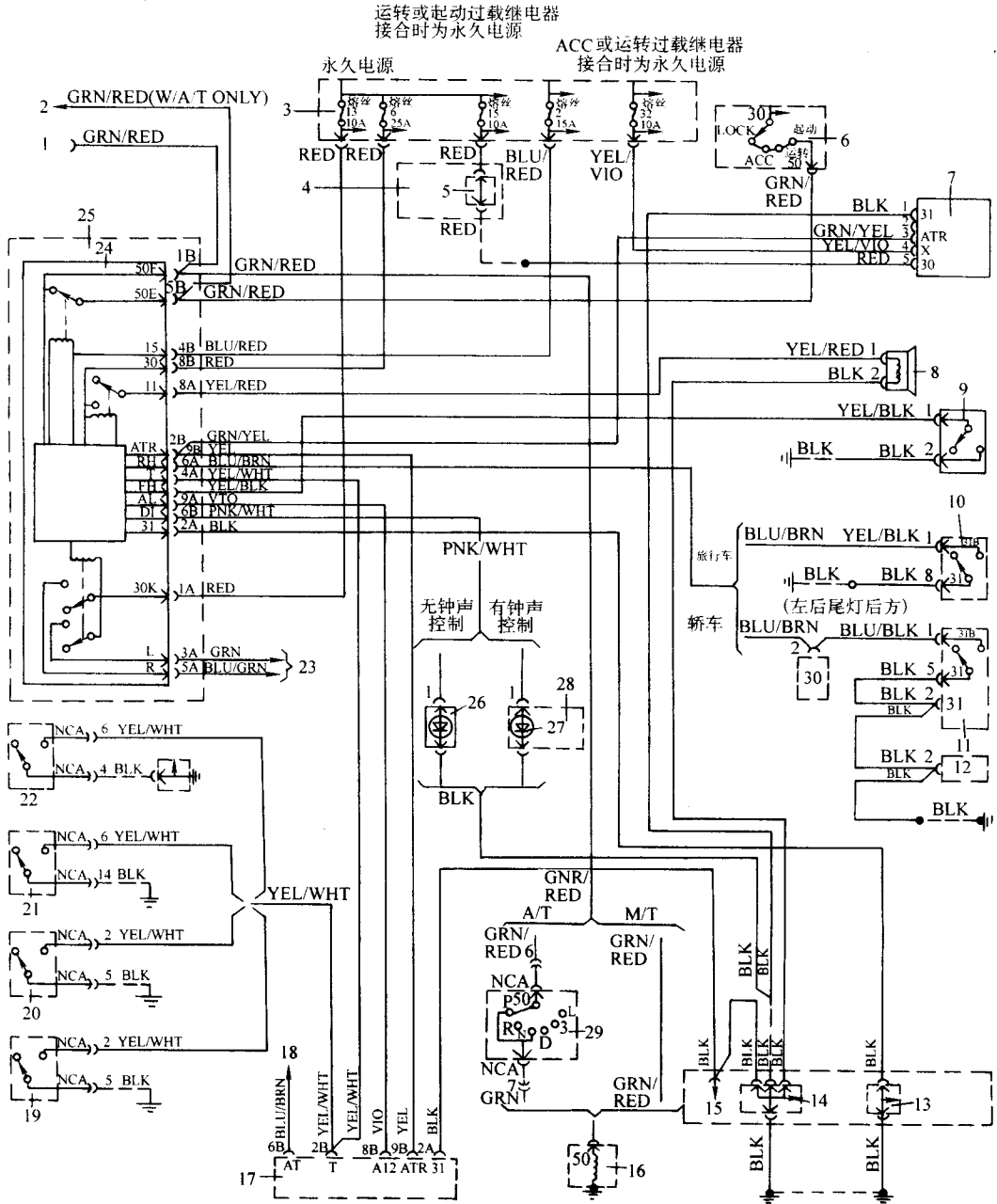
图 8-11 沃尔沃 850Base Model 防盗系统电路 (1995~1996 年车型)
