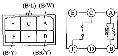
图 4-16 检查起动机断电继电器
