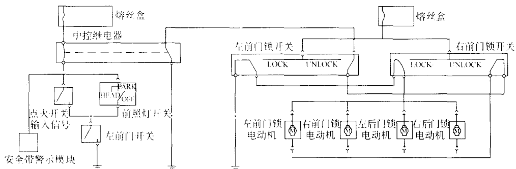
图 12-2 Acclaim、Lebaron Sedan 和 Sprit 中控电路
