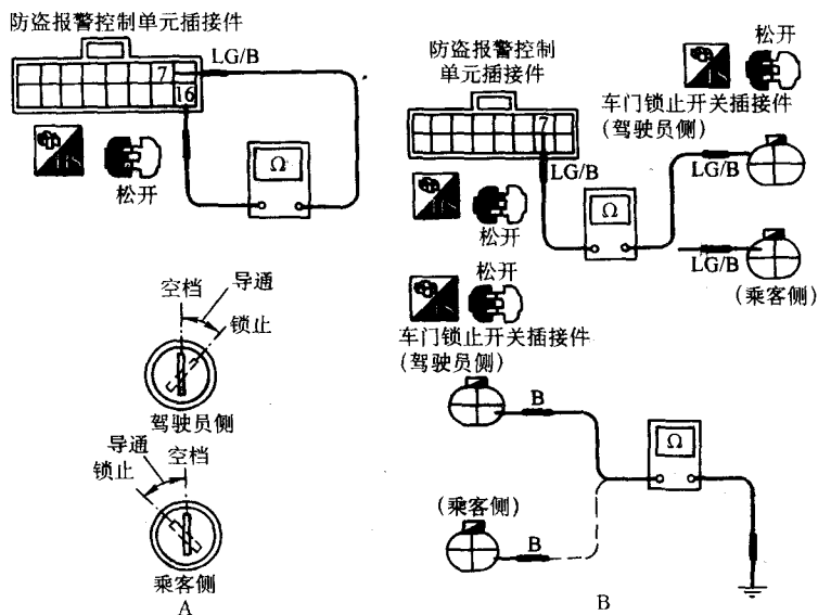
图 3-61 诊断步骤 4 流程
