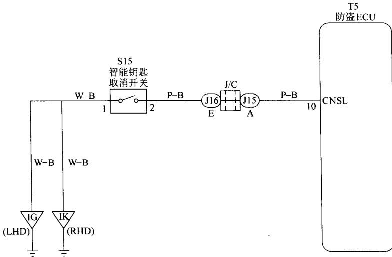
图 2-39 智能钥匙系统取消开关电路
