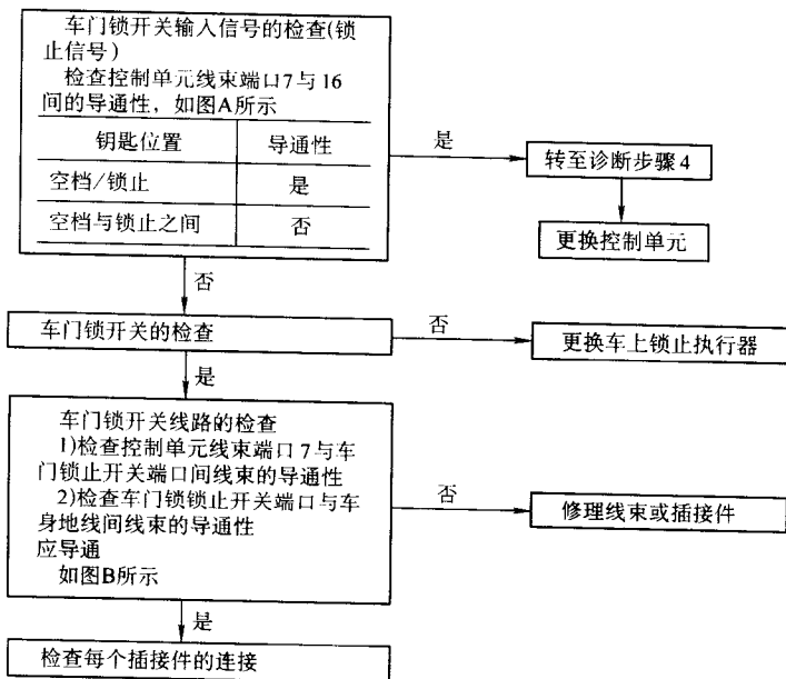
图 3-61 诊断步骤 4 流程 (续)
