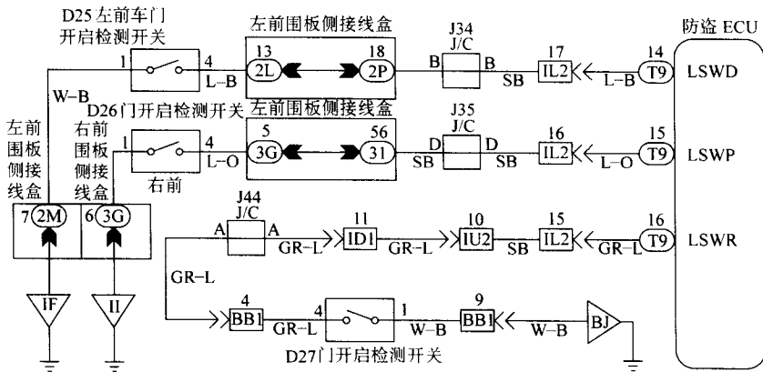
图 2-22 车门开启检测开关电路
