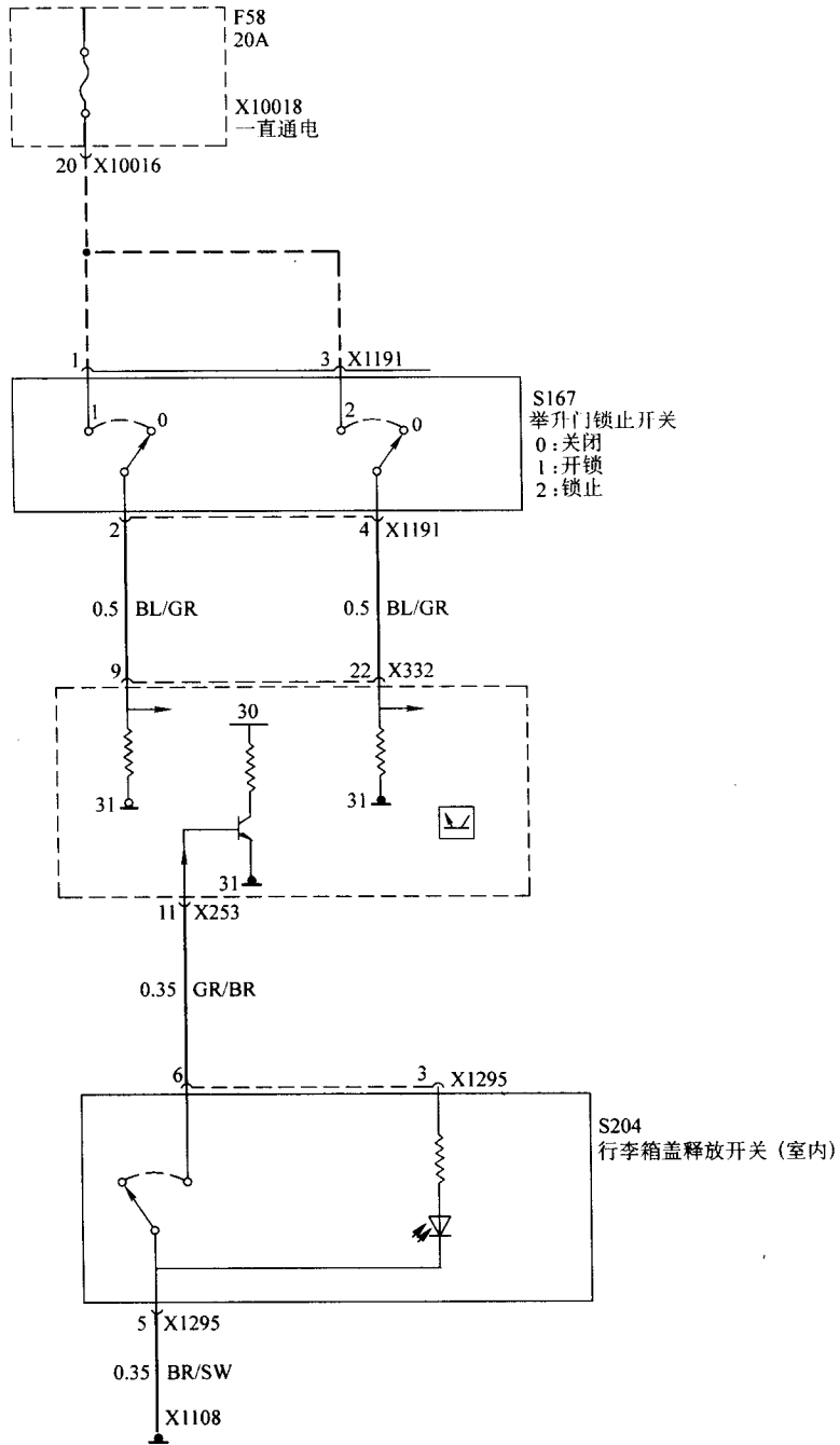
图 7-29 宝马 740i 和 750il (E38) 防盗系统行李箱盖开关电路 (1996 年车型)
