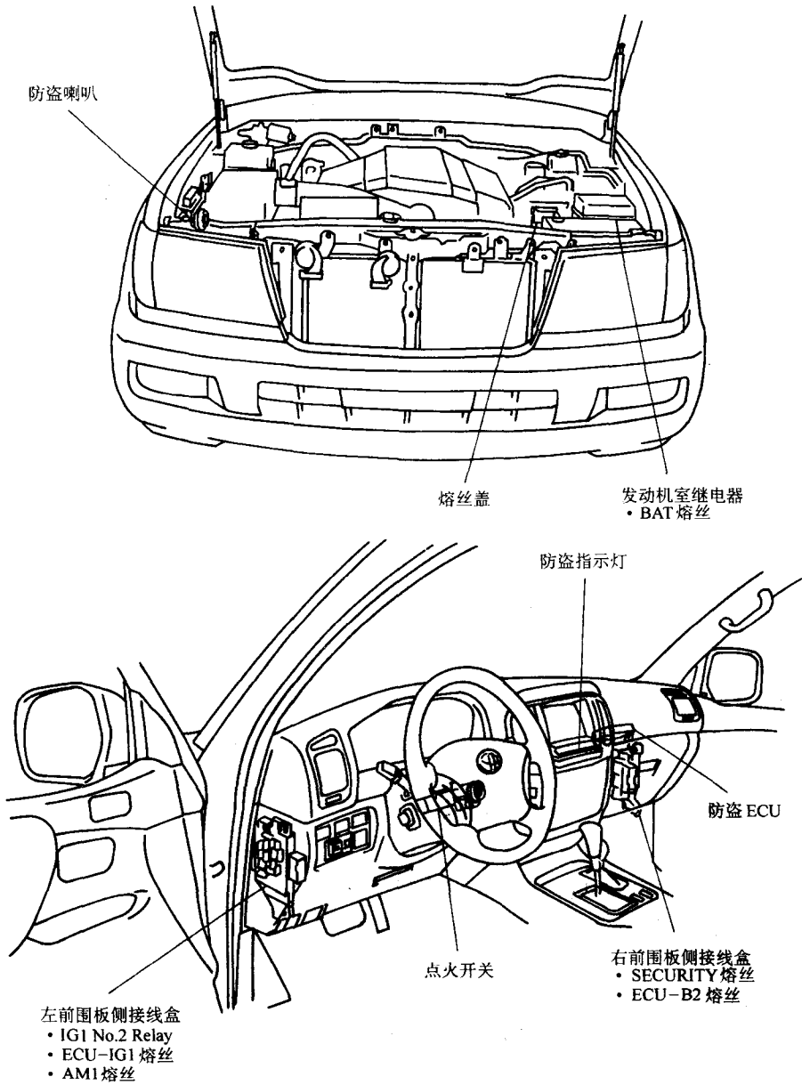
图 2-3 防盗系统电控元件位置
