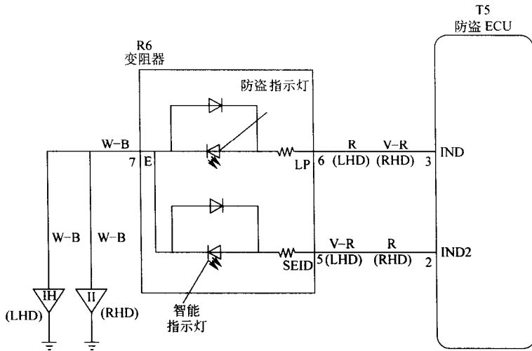
图 2-32 防盗指示灯电路
