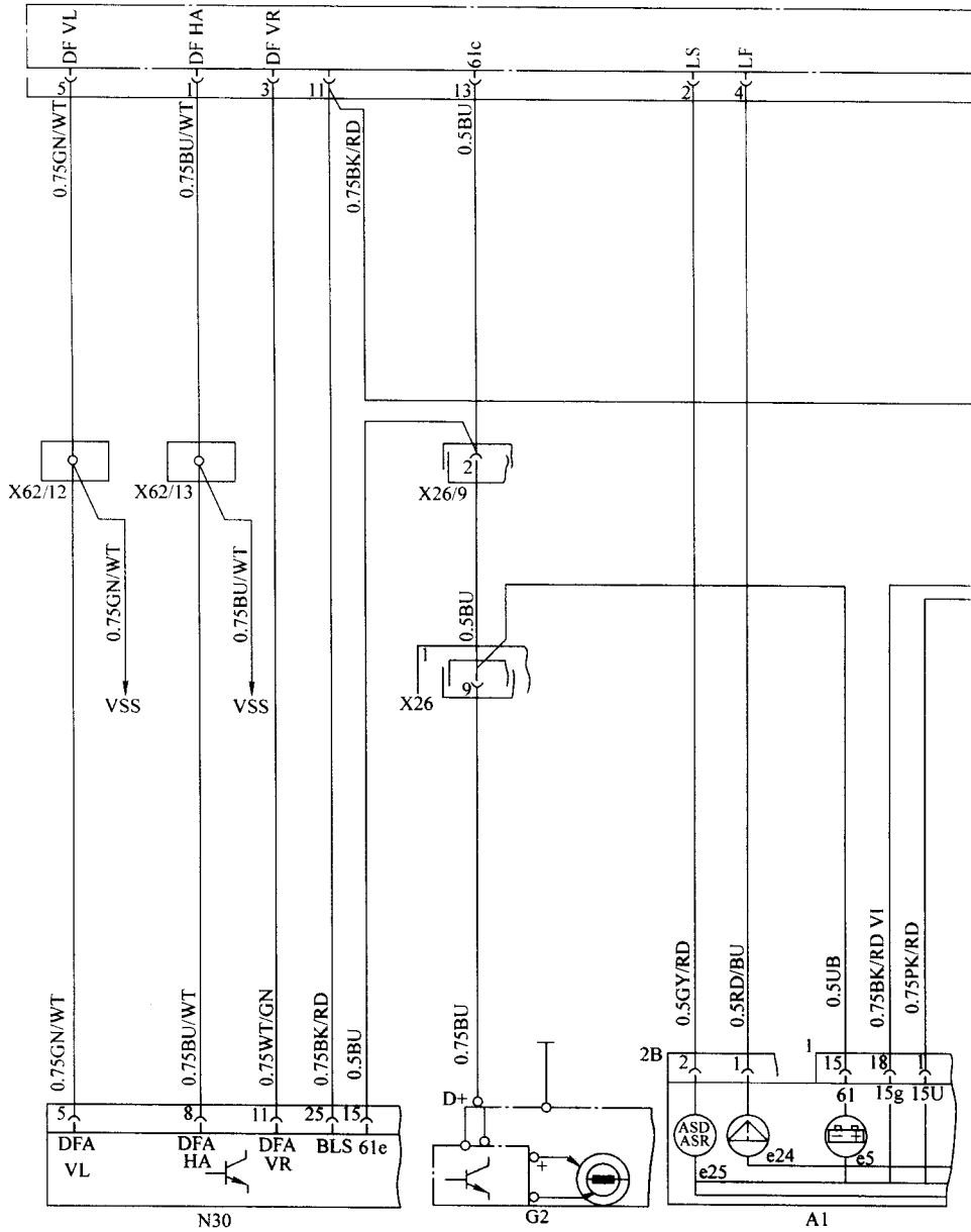
图 6-46 SL320 和 SL600 防盗报警系统电路图之一 (1997 车型)
