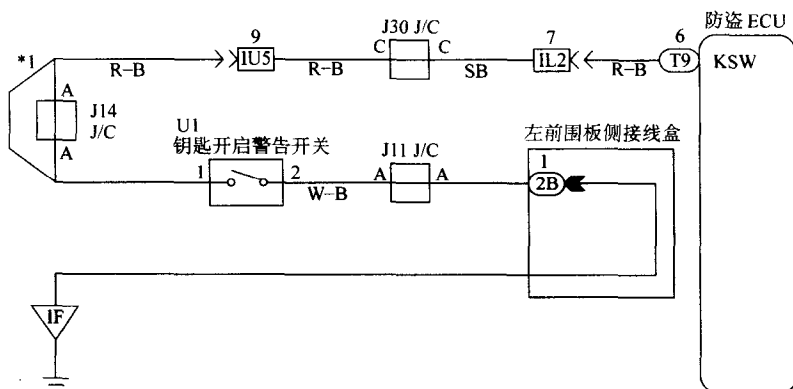
图 2-17 钥匙开启警告开关电路
