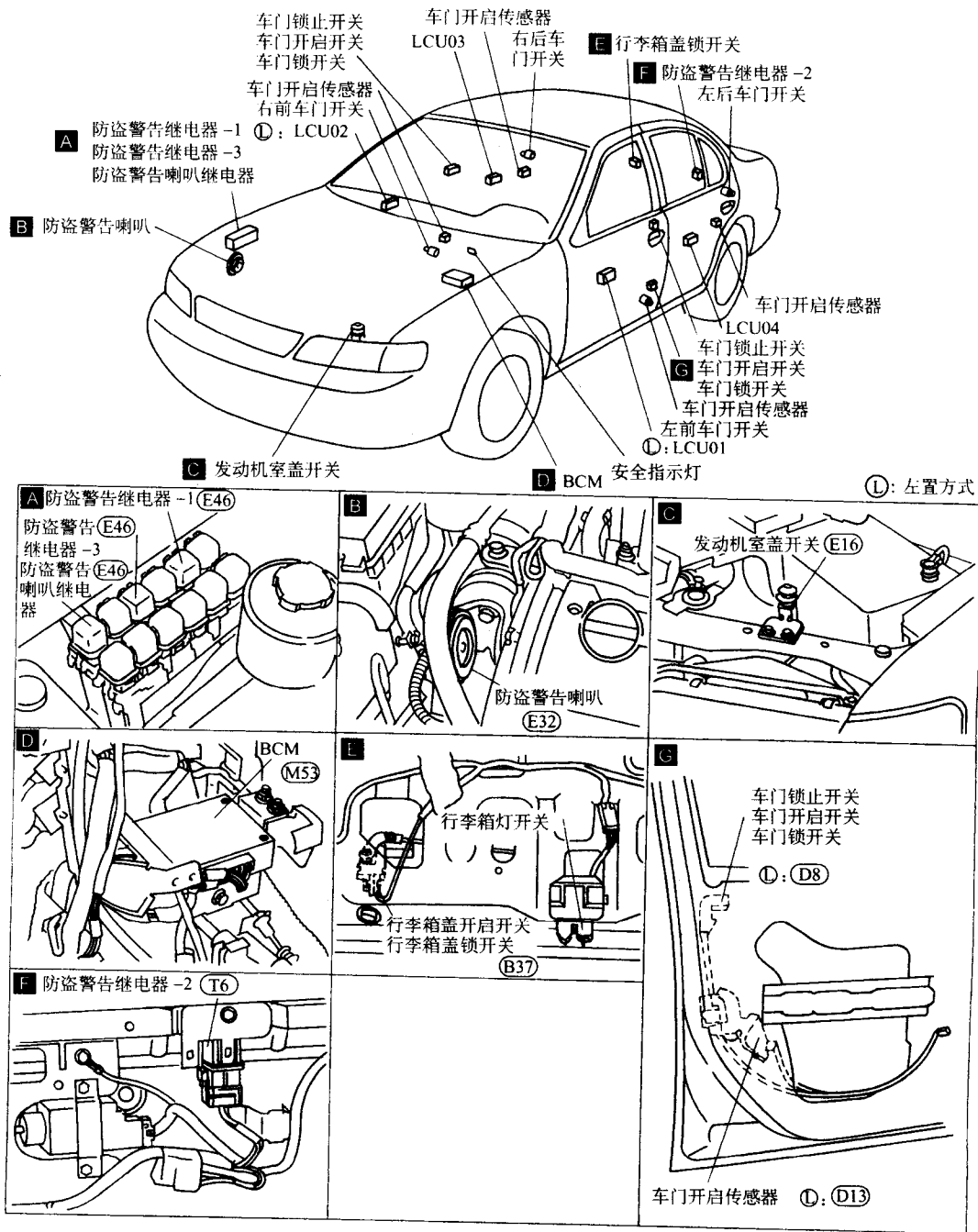
图 3-11 防盗系统零部件及线束接头位置
