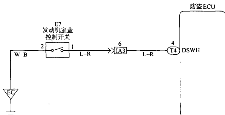
图 2-53 发动机室盖控制开关电路
