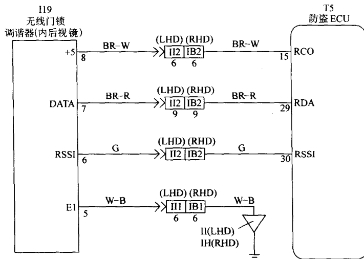
图 2-31 遥控门锁接收器(内后视镜)电路
