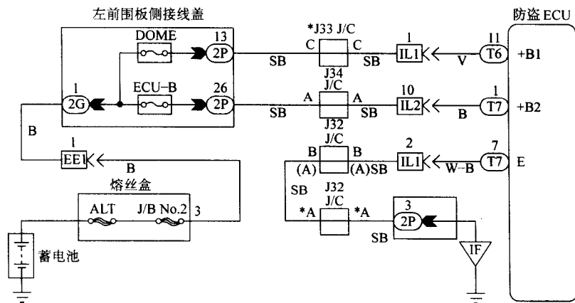
图 2-12 防盗 ECU 电源电路
