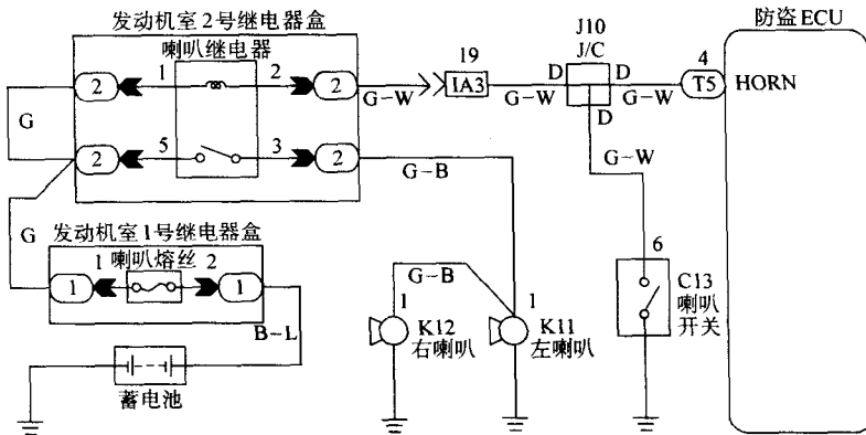
图 2-45 喇叭继电器电路
