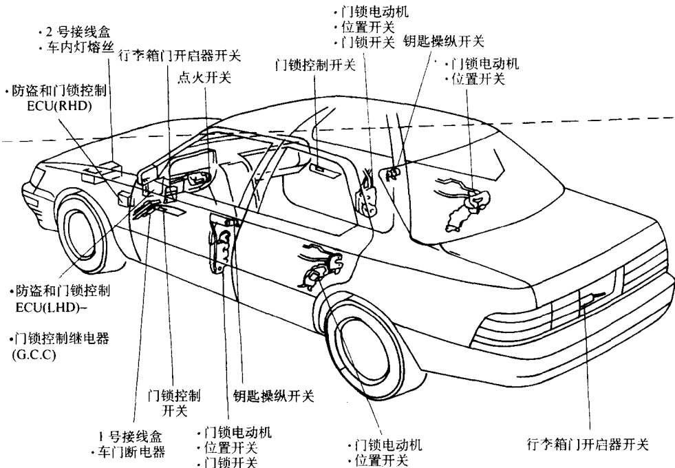
图 2-54 凌志 LS400 中央门锁系统元件位置
