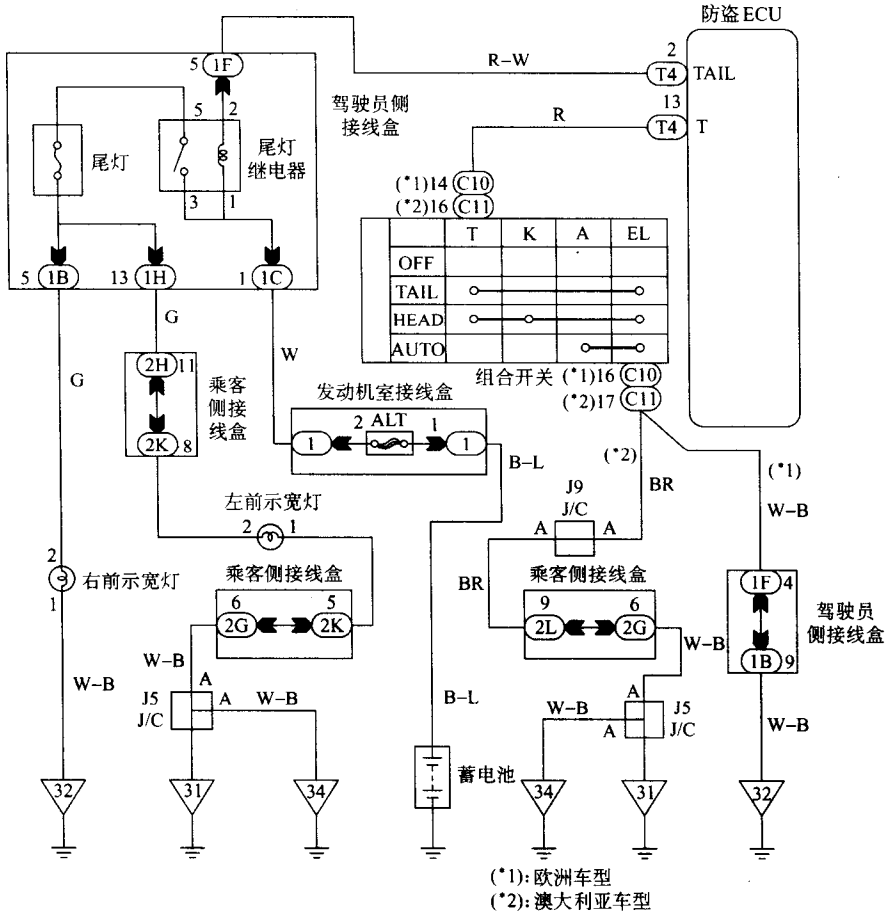
图 2-48 尾灯继电器电路
