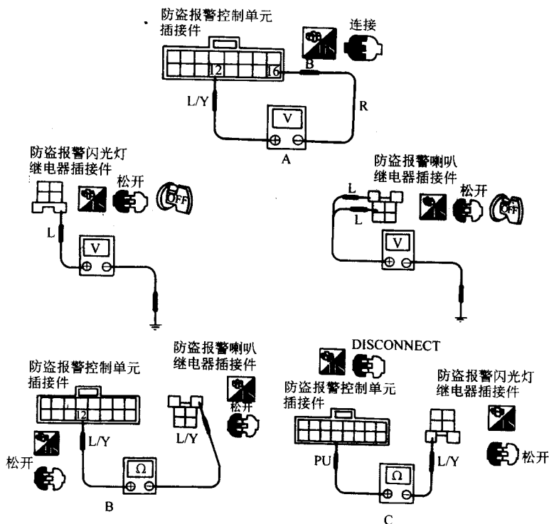
图 3-62 诊断步骤 5 流程
