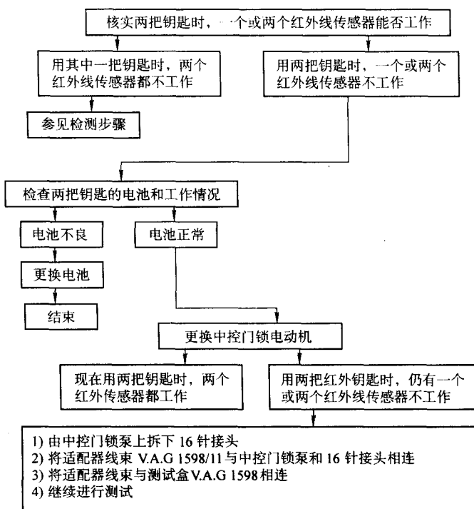
图 5-8 诊断流程
