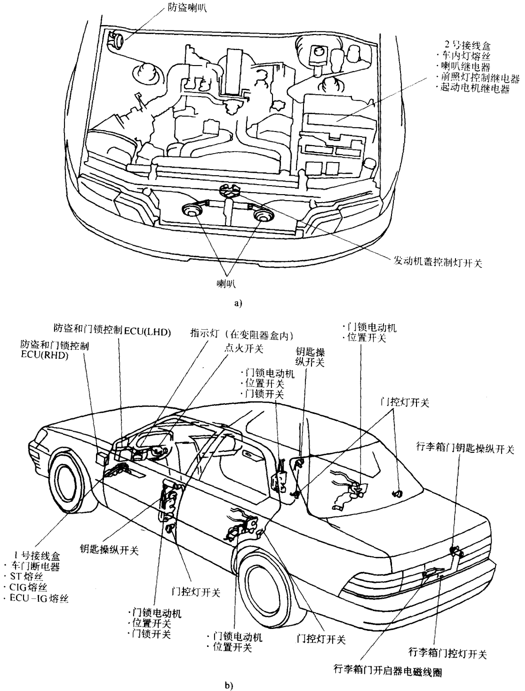
图 2-58 丰田凌志 LS400 与 ES300 防盗系统的元件布置
