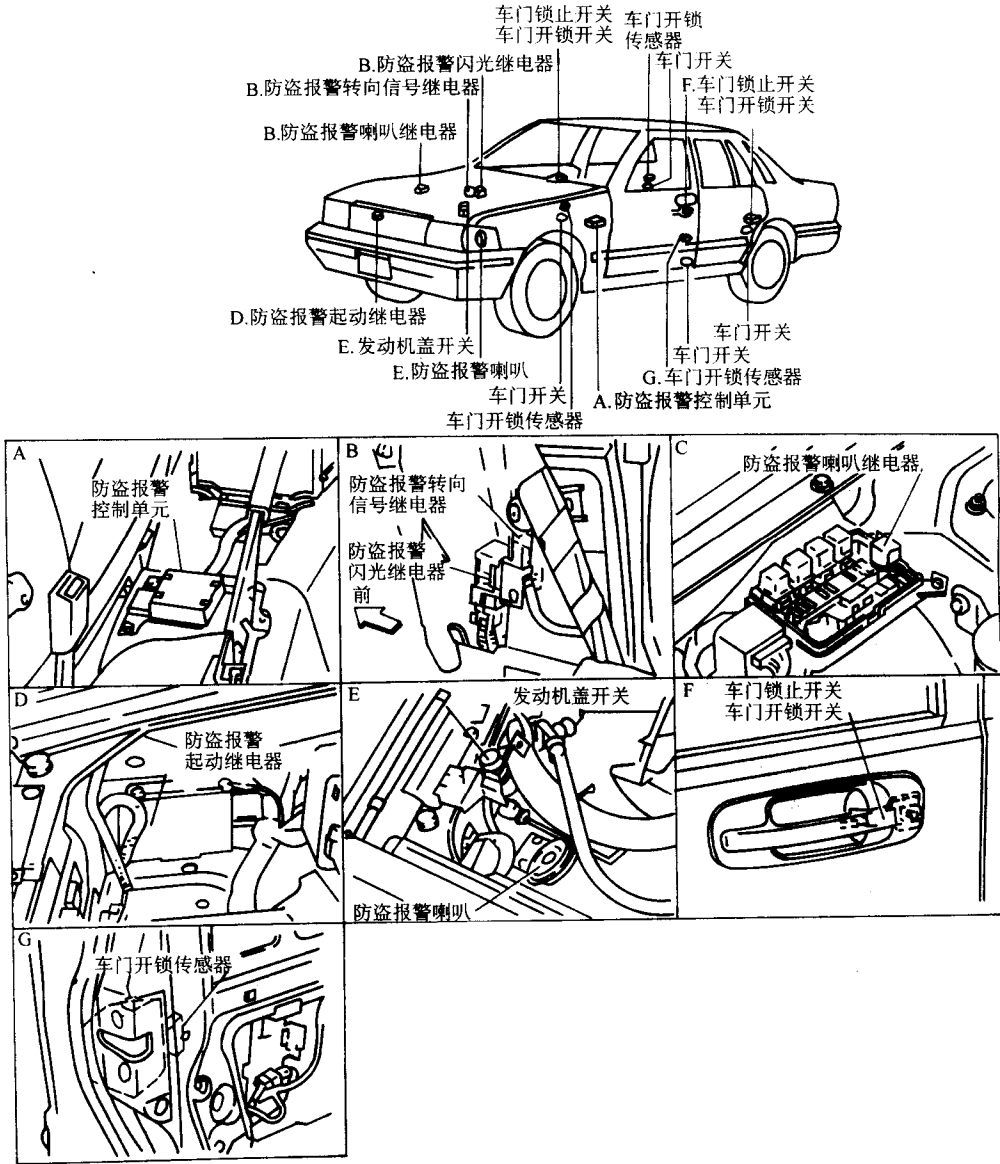
图 3-51 日产风度防盗系统元件位置
