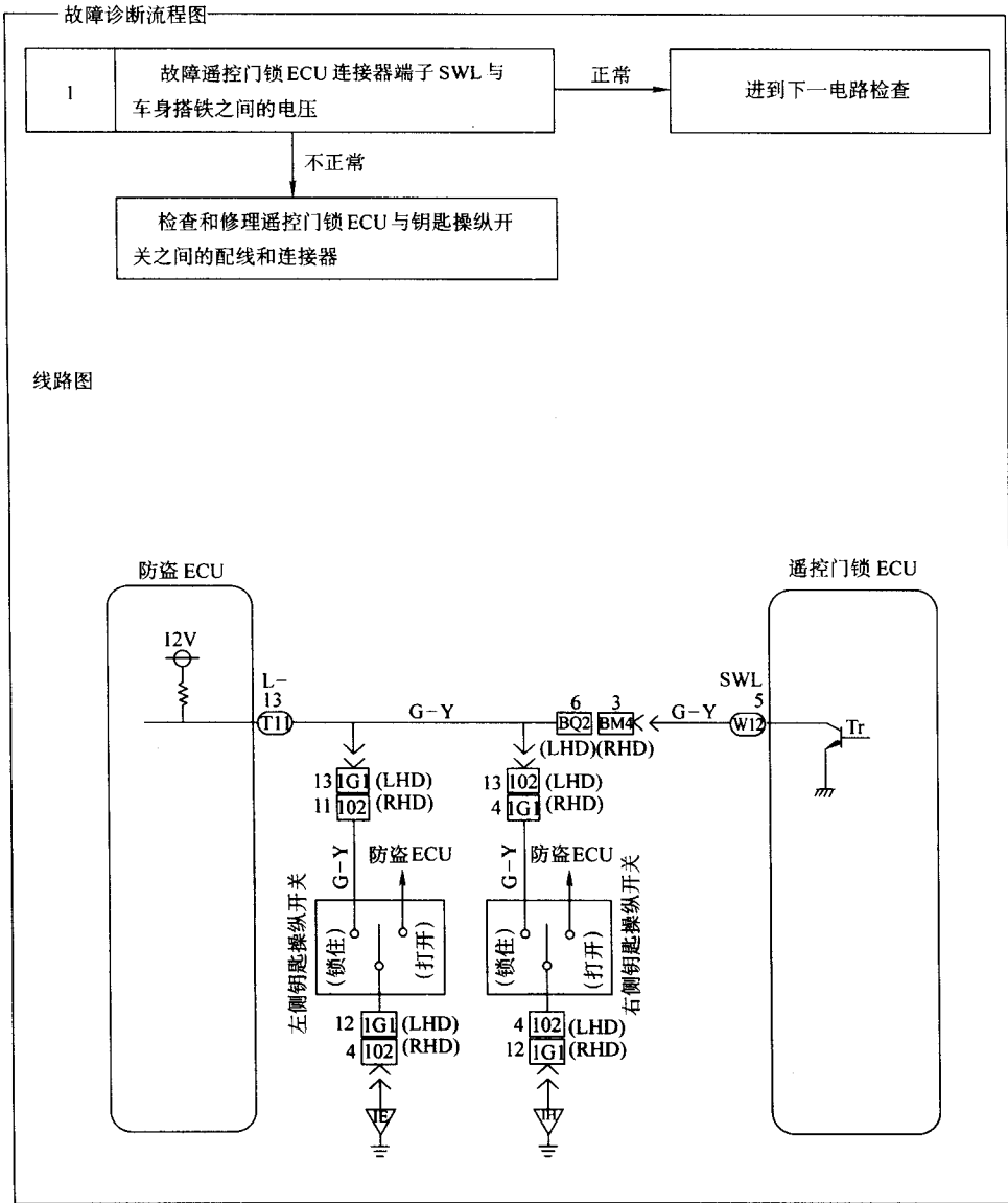
图 2-71 钥匙操纵开关电路检查
