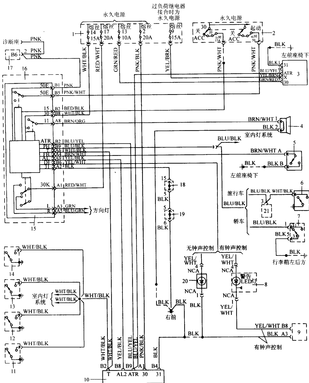
图 8-22 沃尔沃 960 BASE MODEL 防盗系统电路
