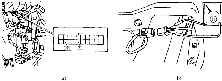
图 4-10 车门钥匙锁芯置于“UNLOCK”、报警不停止的故障排除
