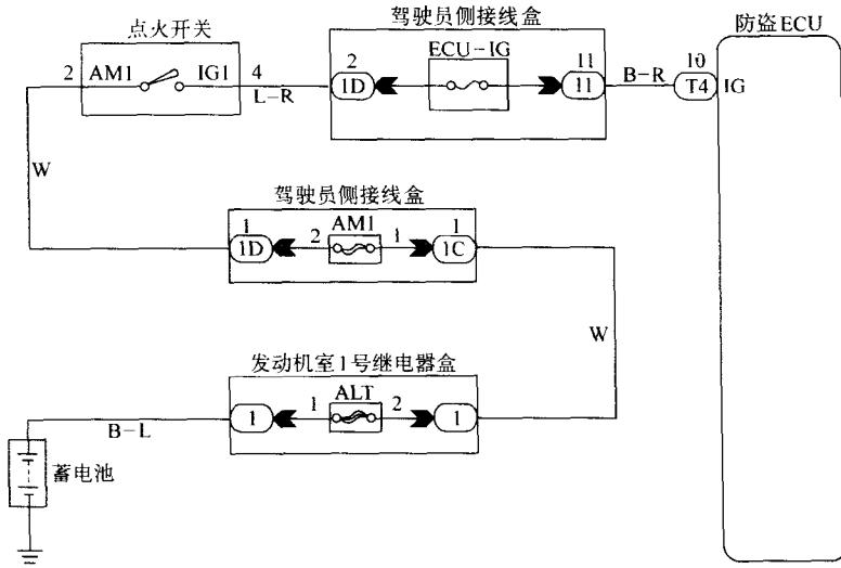
图 2-44 点火开关电路
