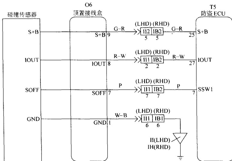
图 2-27 故障码 B2761 检查电路
