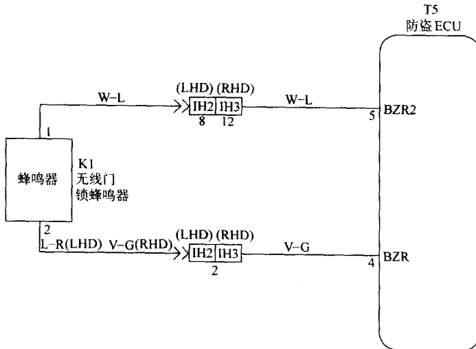
图 2-29 遥控门锁蜂鸣器电路
